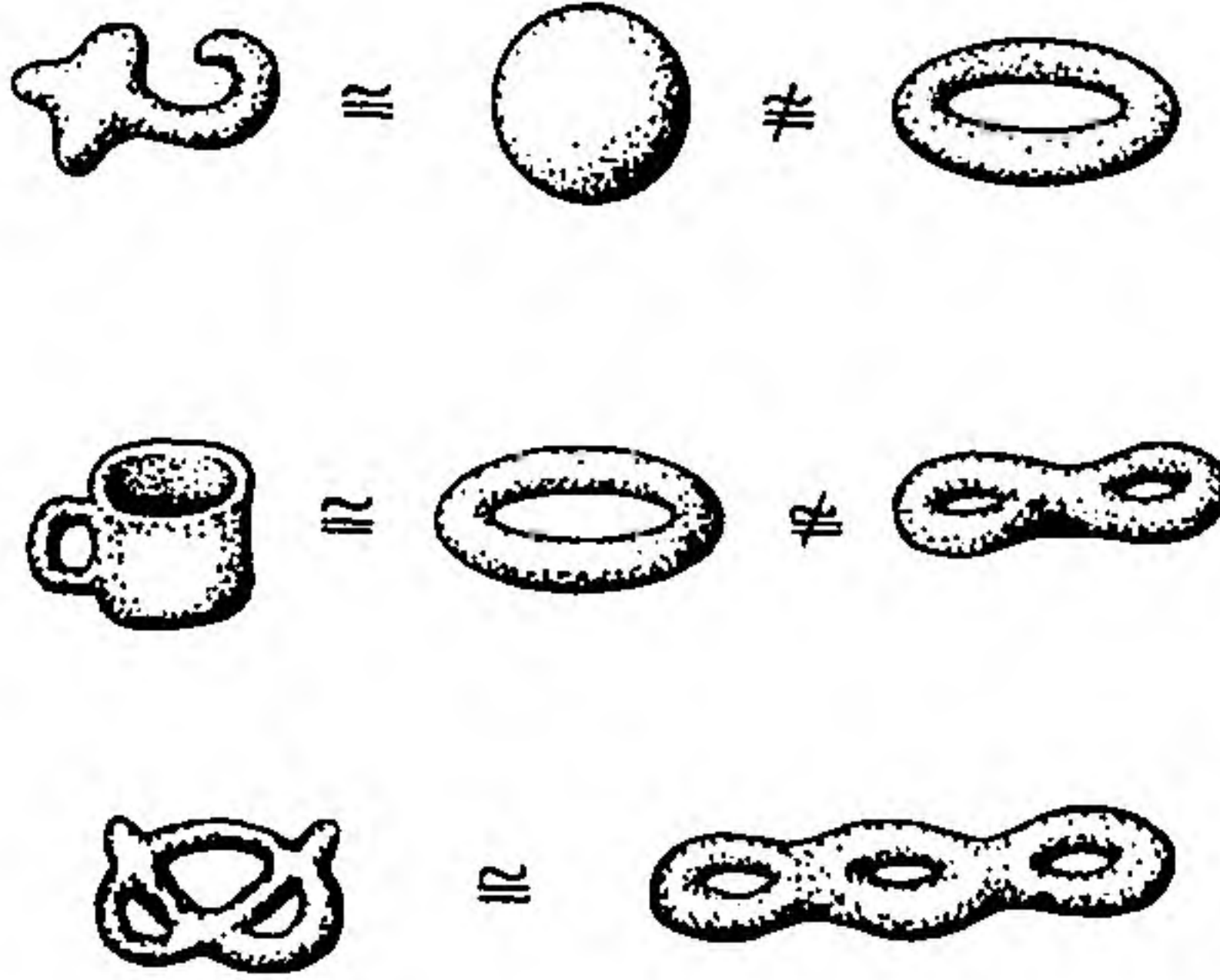
Şekil 7.14 İki boyutlu kapalı yüzeyler hesaplanabilir şekilde (kabaca “tutamakların” sayısının sayılmasıyla) sınıflandırılabilirler. Öte yandan dört boyutlu kapalı “yüzeyler” hesaplanabilir şekilde sınıflandırılmazlar.
