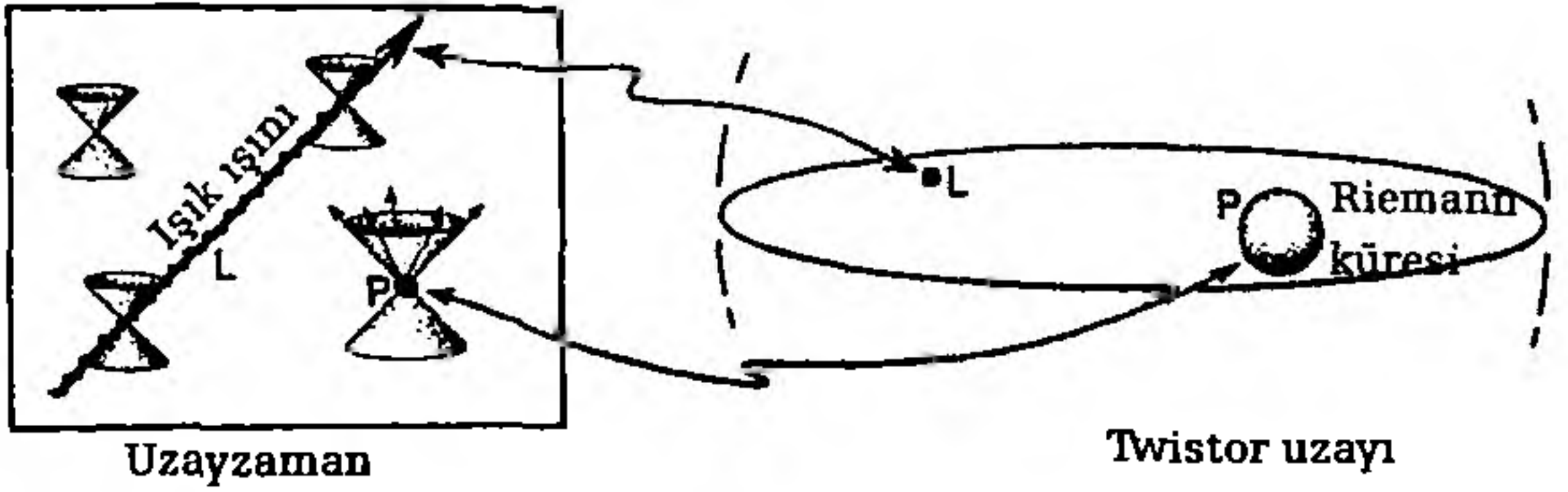
Şekil 7.17 Twistor kuramı ışık ışınlarının her birini birer noktayla, olayları da Riemann küreleriyle göstererek uzayzamanın betimlenmesinde alternatif bir fiziksel betimleme sağlar.
