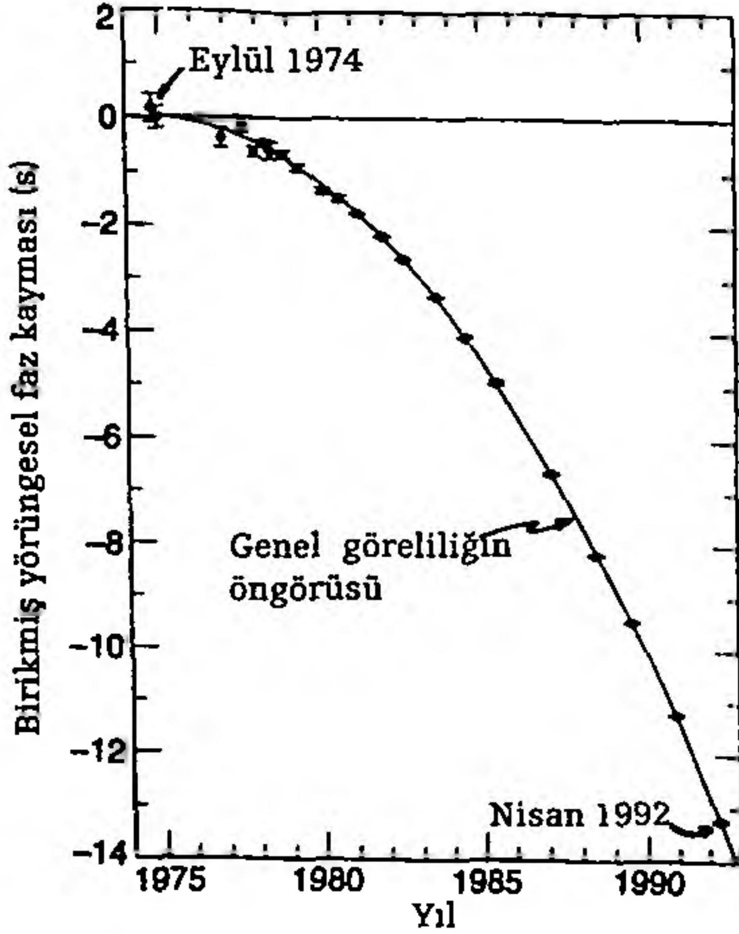
Şekil 4.11 Bu çizelge (Joseph Taylor'ın izniyle) 20 yıllık bir sürede pulsarın karşılıklı yörüngesinde gözlemlenen hızlanma ile Einstein'ın kuramına göre hesaplanan kütleçekim ışıması sebebiyle enerji kaybı arasındaki kesin örtüşmeyi göstermektedir.
