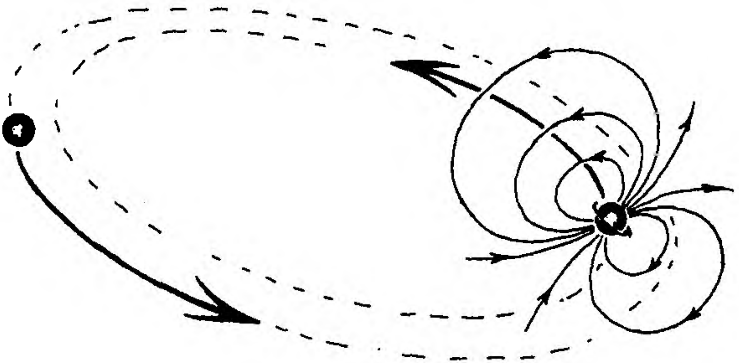
Şekil 4.9 PSR 1913 + 16. İki nötron yıldızı birbirleri etrafında dönmektedir. Bunlardan biri bir pulsardır ve yüklü parçacıkları yakalayan olağanüstü derecede güçlü bir manyetik alana sahiptir.
