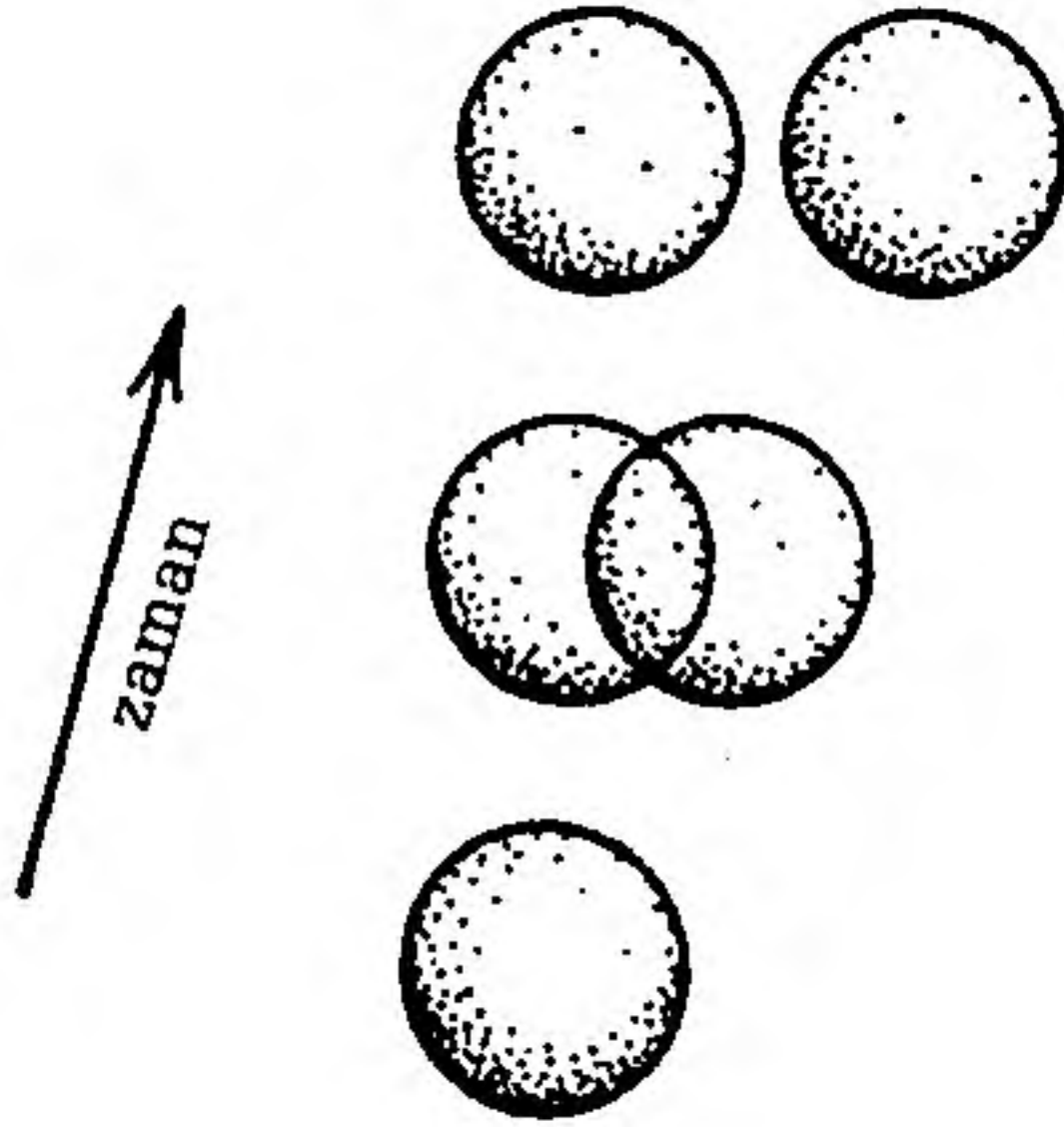
Şekil 6.6 İndirgenme süresi h/E 'yi hesaplamak için topağın bir parçasının diğerinden ayrıldığını hayal edin ve sadece kütleçekim çekmelerini dikkate alarak bunun bedeli olacak olan E enerjisini hesaplayın.
