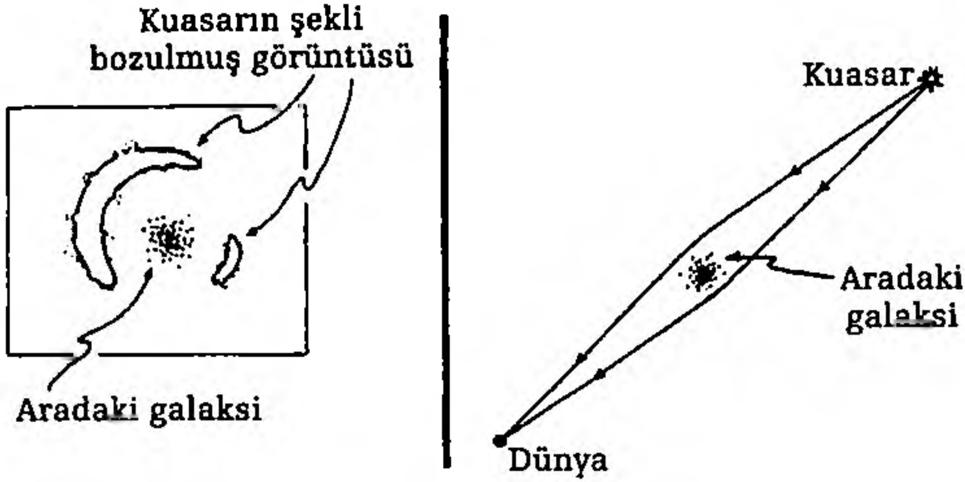
Şekil 4.8 Einstein'ın ışık bükülme etkisi bugün gözlemsel astronomide önemli bir araçtır. Arada bulunan bir galaksinin kütlesi onun uzaktaki bir kuasarın görüntüsünü ne kadar bozduğundan yola çıkılarak tahmin edilebilir.
