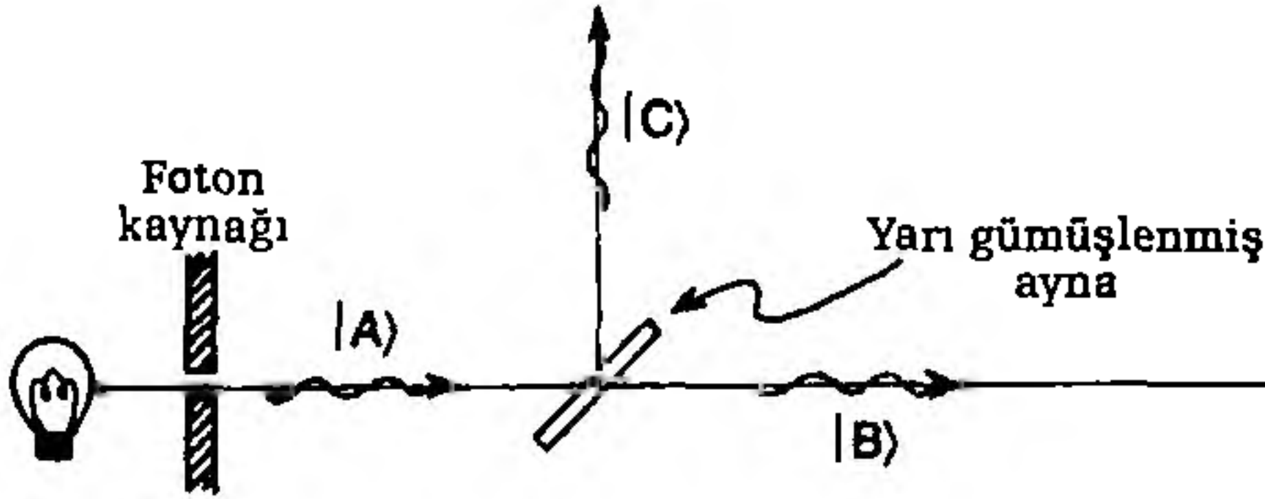
Şekil 5.11 |A\rangle durumunda bir foton yarı gümüş bir aynaya çarpıyor ve durumu (U sonucunda) |B\rangle + i|C\rangle şeklinde bir üst üste binmeye evrimleşiyor.
