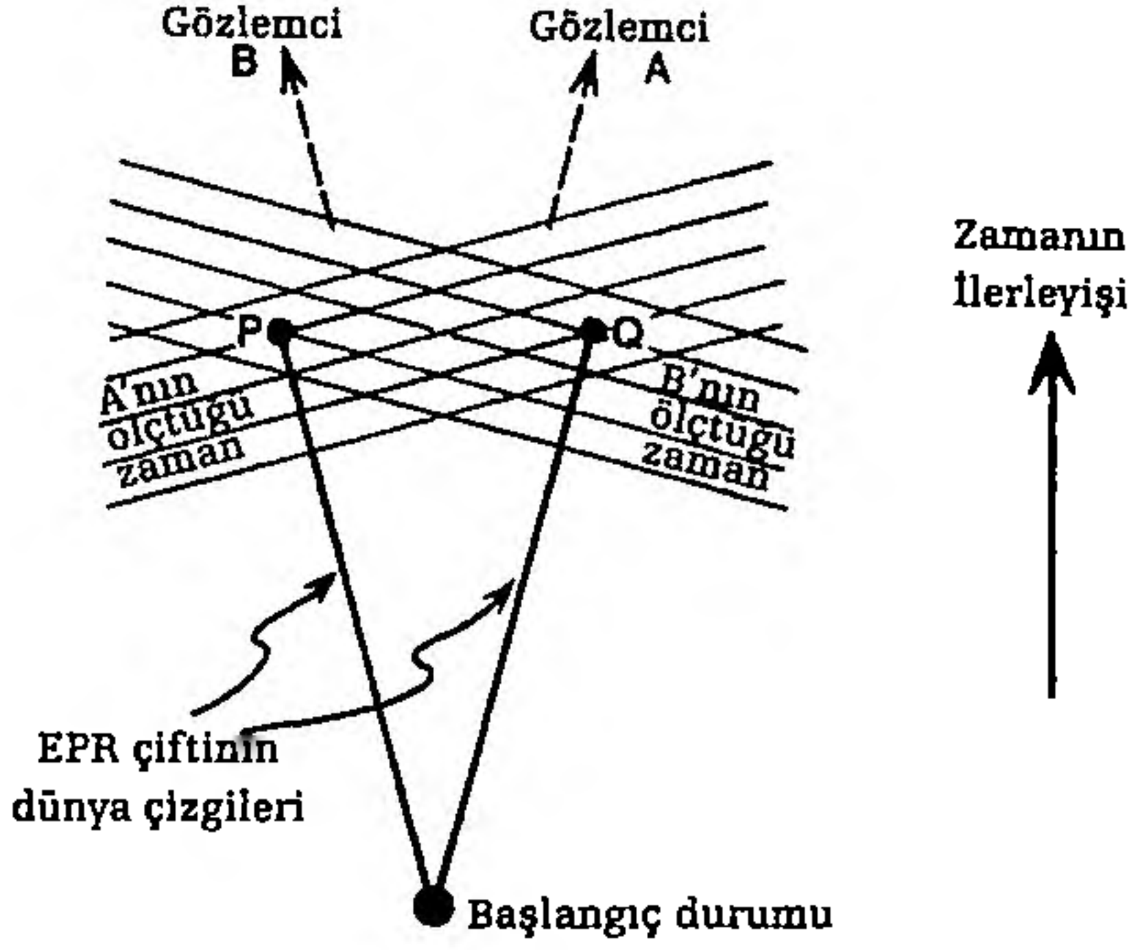
Şekil 5.26 Özel göreliliğe göre göreceli hareket eden A ve B gözlemcileri uzaysal olarak ayrılmış P ve Q olaylarından hangisinin daha önce gerçekleştiğine ilişkin farklı fikirlere sahiptir.
