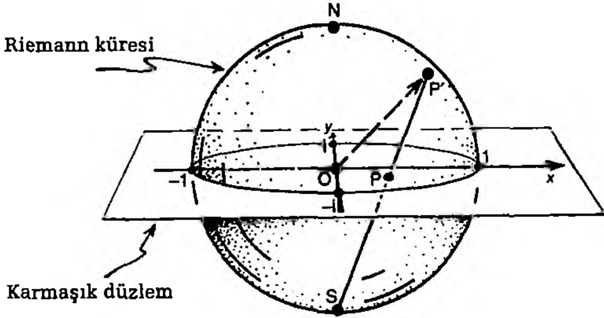
Şekil 5.19 Riemann küresi. Karmaşık düzlemde p = z/w 'yi temsil eden P noktası güney kutup noktası S'den küre üzerindeki P' noktasına yansıtılır (izdüşümü alınır). Kürenin merkezi O'dan başlayan OP yönü Şekil 5.15'teki genel 1/2 spin için spin yönüdür.
