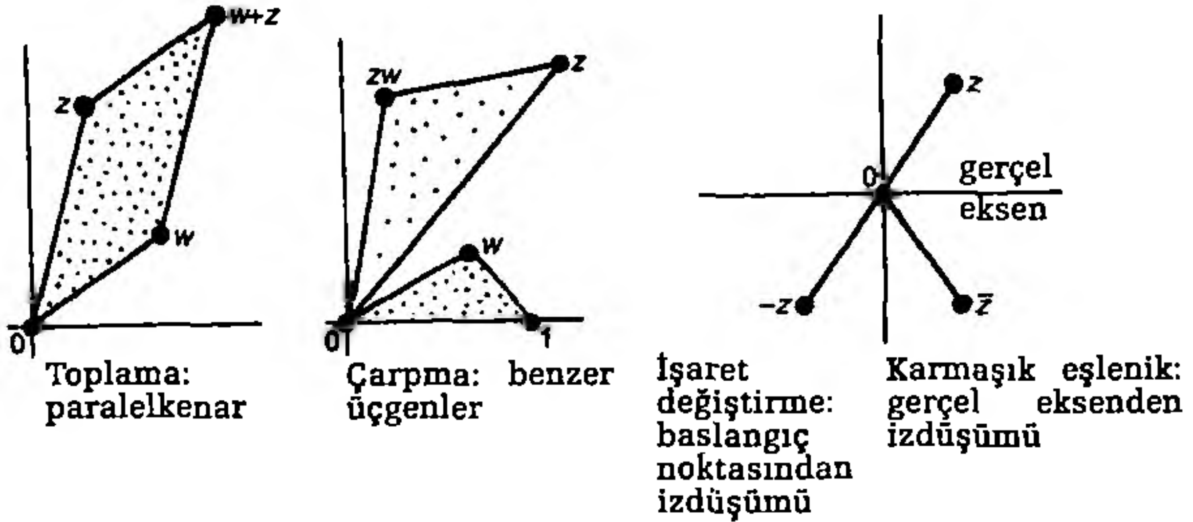
Şekil 5.17 Karmaşık sayılardaki temel işlemlerin geometrik temsilleri
