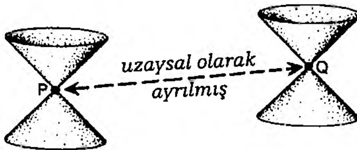
Şekil 5.25 Uzayzamanda iki olaya eğer ikisi de birbirinin ışık konisinin dışında yer alıyorsa uzaysal olarak ayrılmış denir (ayrıca bkz. Şekil 4.1) Bu durumda birbirlerini nedensel olarak etkileyemezler ve iki olayda yapılan ölçümler değişmeli olmak zorundadır.
