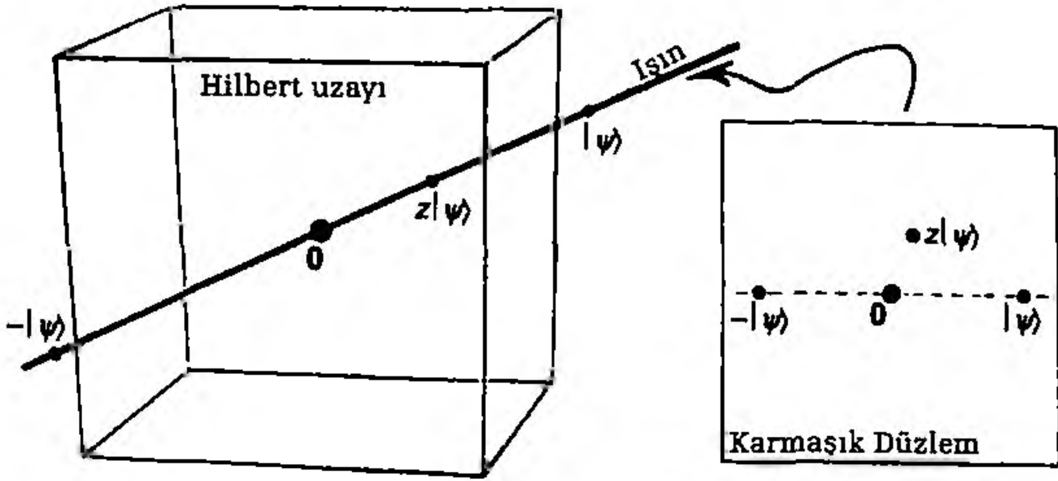
Şekil 5.23 Hilbert uzayında bir ışın, durum vektörü |\psi\rangle 'nün karmaşık katlarının hepsinden oluşur. Bunu Hilbert uzayı orijini 0'dan geçen düz bir çizgi olarak düşünüyoruz, ama bu düz çizginin gerçekte bir karmaşık düzlem olduğunu unutmamalıyız.
