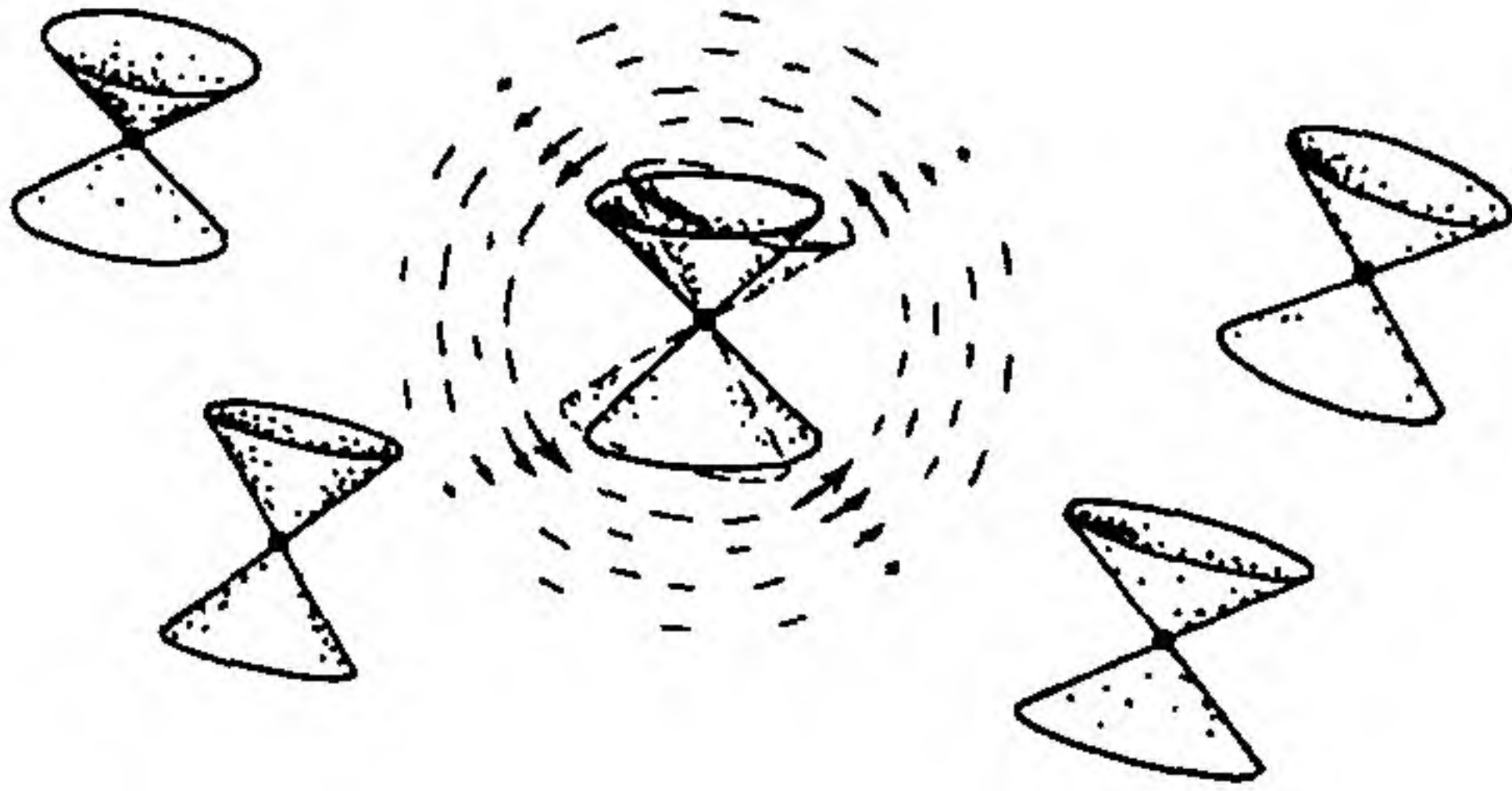
Şekil 4.6 Uzayzamanın üzerine ışık konileri çizilmiş olan bir lastik çarşaf olduğunu hayal edin. Herhangi bir ışık konisi döndürülerek (lastik çarşafı da kendisiyle birlikte taşıyarak) standart bir Minkowski tarifine getirilebilir.
