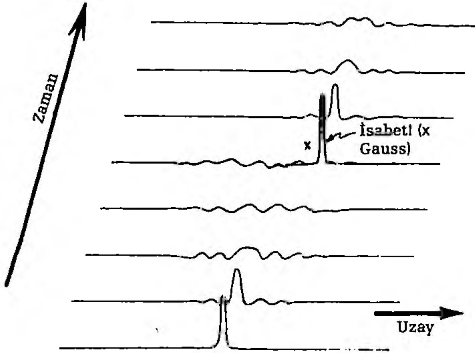
Şekil 6.2 Özgün Ghirardi-Rimini-Weber (GRW) düzenlemesinde dalga fonksiyonu çoğu zaman standart Schrödinger U evrimi uyarınca evrilir; ancak kabaca (parçacık başına) 10^8 yılda bir, durum bir "isabet" alır ve parçacığın dalga fonksiyonu tepe yapan bir Gauss fonksiyonuyla, diğer bir ifadeyle R'nin GRW versiyonuyla çarpılır.
