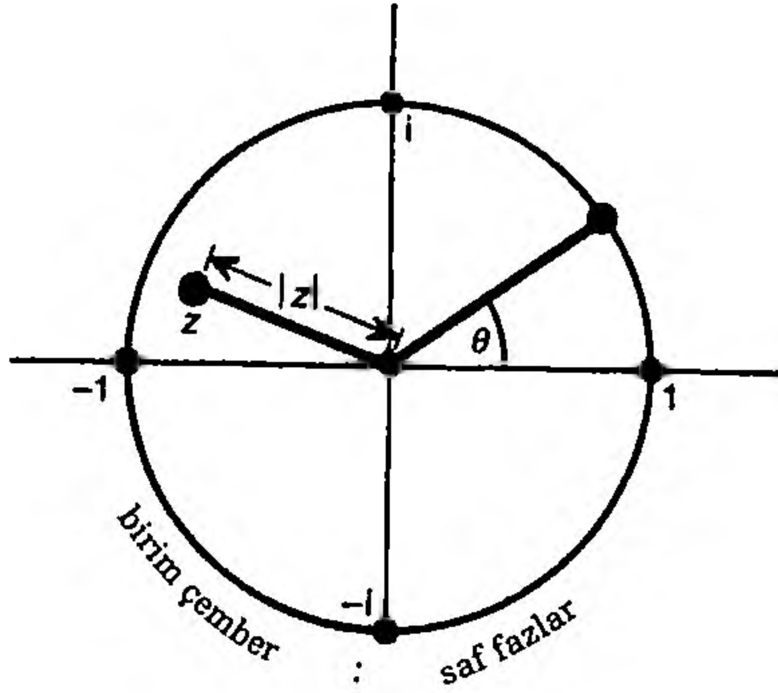
Şekil 5.18 Birim çember karmaşık sayılar z = e^{i\theta} ile \theta gerçel sayısından oluşur, diğer bir deyişle |z| = 1 'dir.
