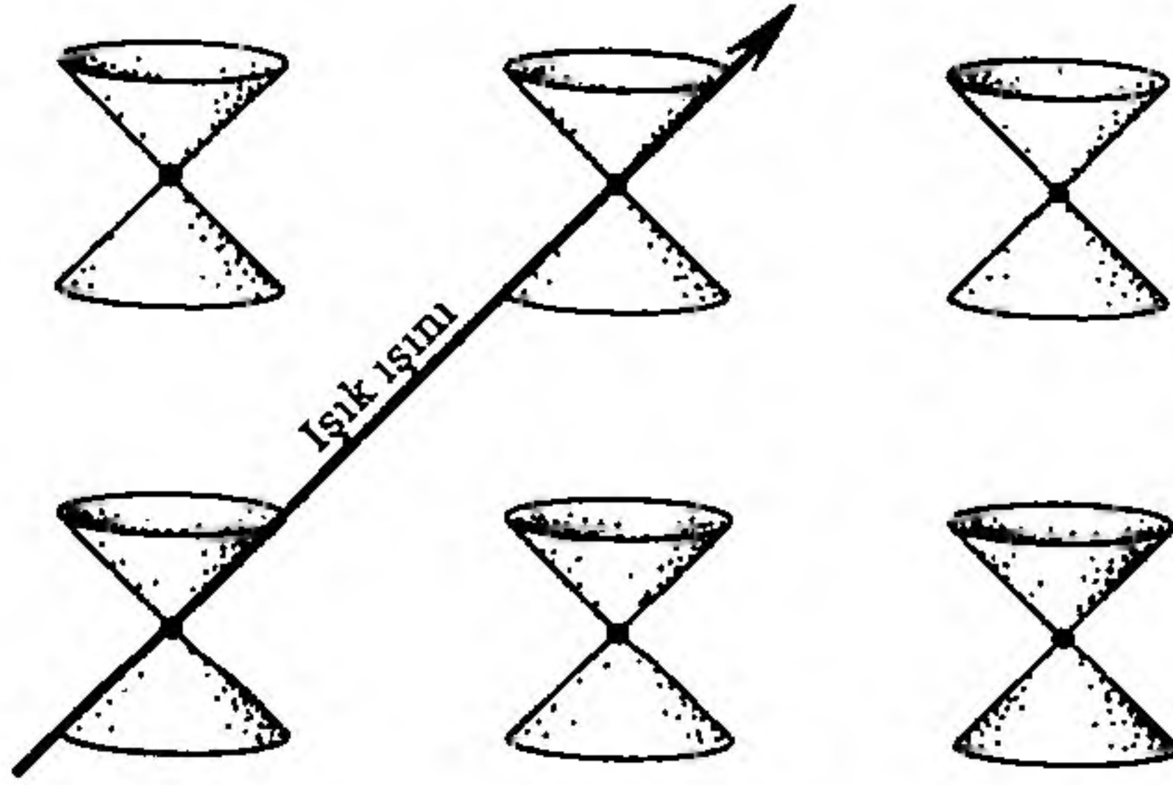
Şekil 4.2 Minkowski uzayı: Özel göreliliğin uzayzamanı. Işık konilerinin hepsi tekdüze şekilde düzenlenmiştir.
