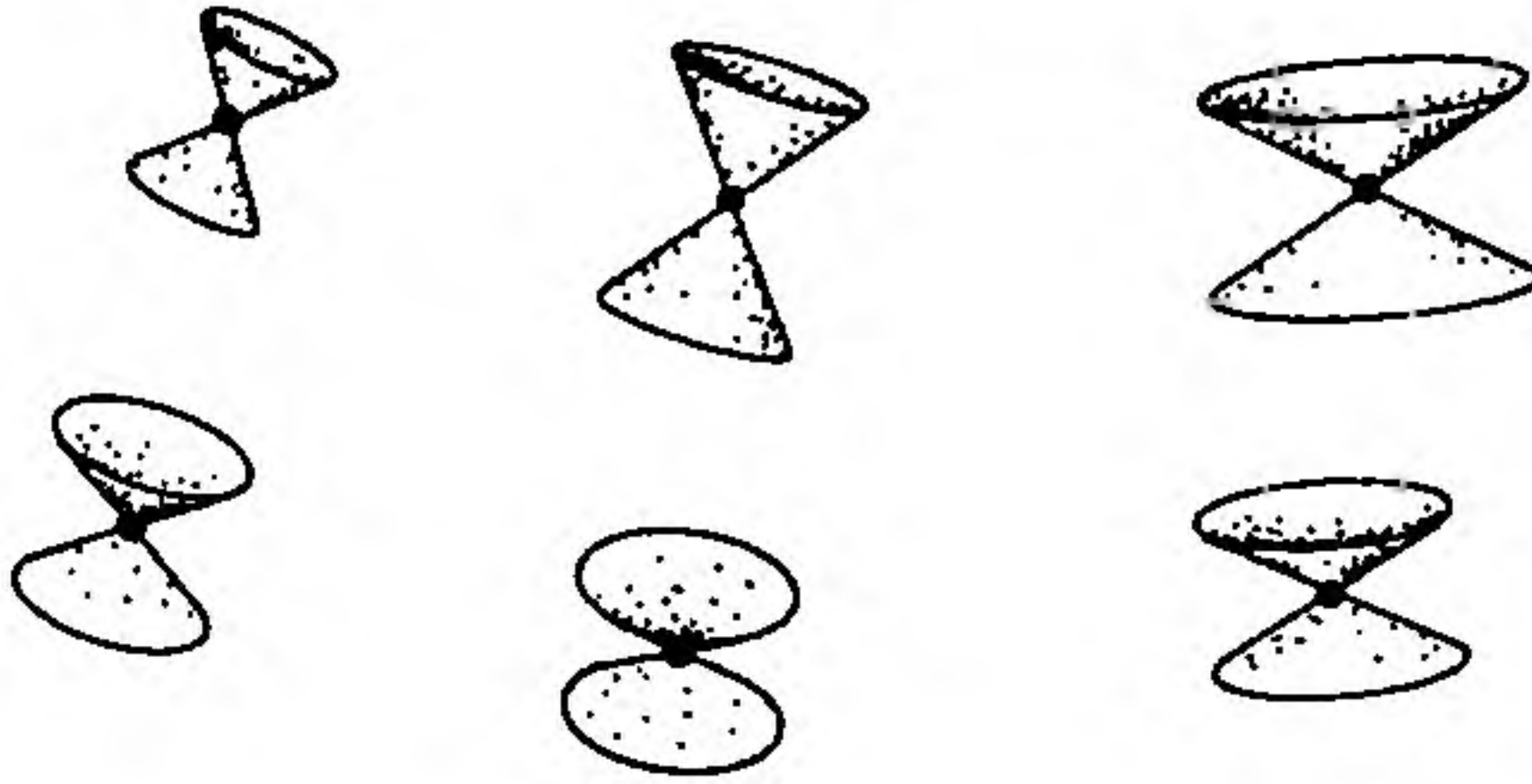
Şekil 4.3 Einstein'ın genel göreliliğindeki yan yatmış ışık konileri.
