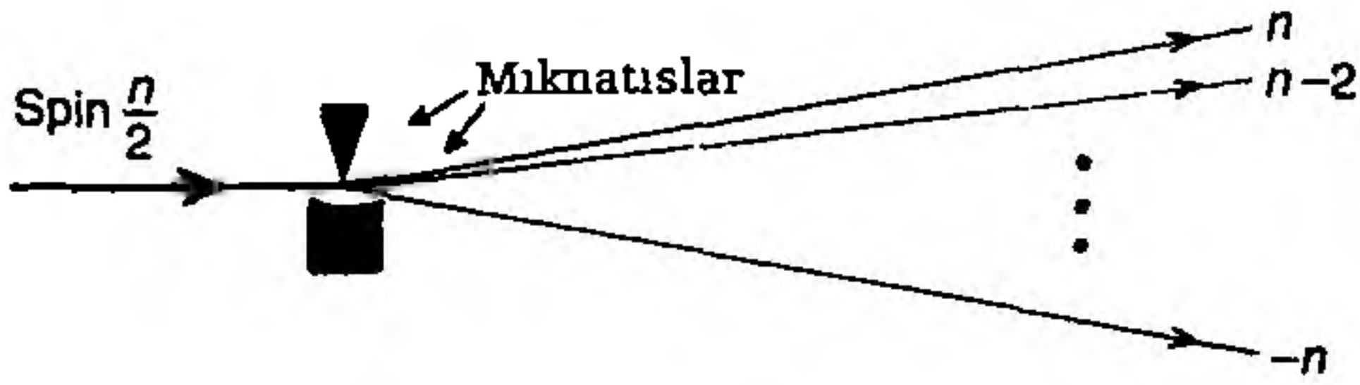
Şekil 5.20 Stern-Gerlach ölçümü. 1/2n spinde spinin ne kadarının ölçülen yönde olduğunun bulunduğuna bağlı olarak n + 1 olası sonuç vardır.
