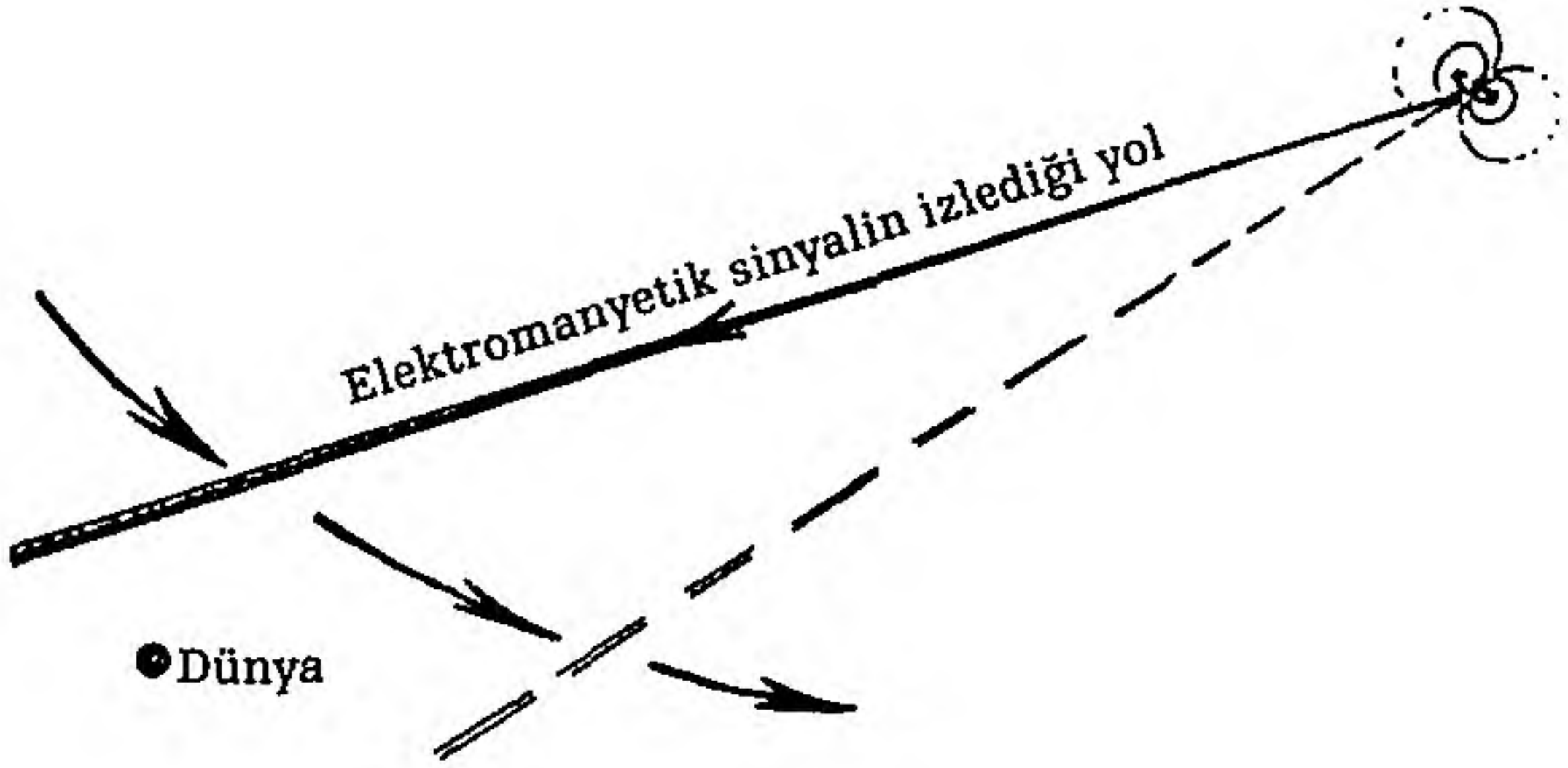
Şekil 4.10 Yakalanan yüklü parçacıklar pulsarla birlikte döne döne sallanır ve ışını dünya tarafından saniyede 17 kez alınan bir elektromanyetik sinyal yayar. Bu keskin darbeli bir radyo sinyali olarak tespit edilir.
