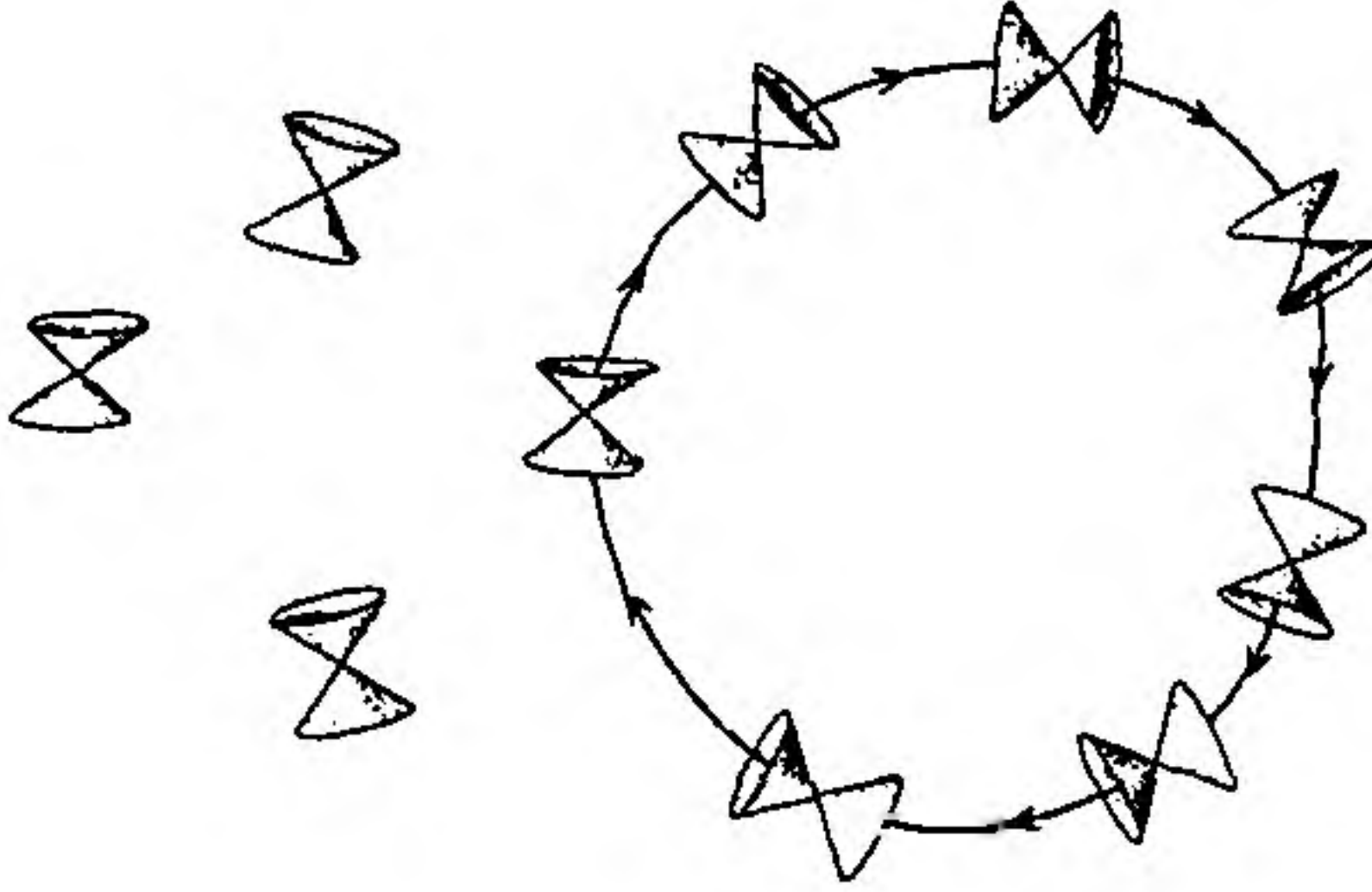
Şekil 7.15 Bir uzayzamanda yeterli şiddette ışık konisinin yan yatmasıyla kapalı zamansal çizgiler gerçekleşebilir.
