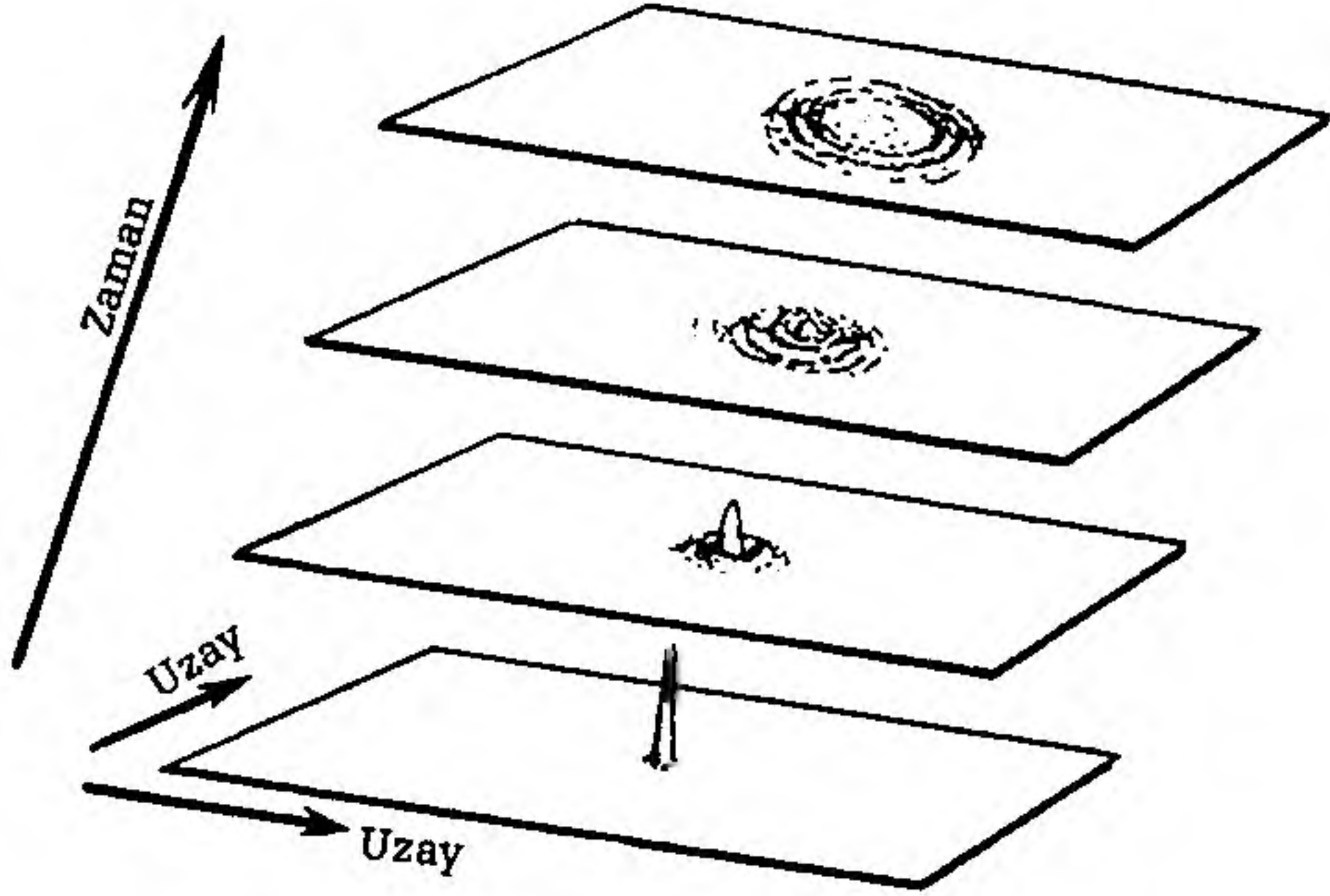
Şekil 6.1 Bir parçacığın dalga fonksiyonunun Schrödinger zaman evrimi: İlk başta esasen bir noktada yerleşmişken ardından dışa doğru her yöne yayılıyor.
