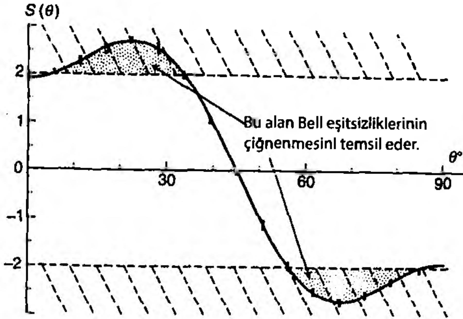
Şekil 5.7 Aspect deneyi Bell'in klasik eşitsizliklerinin çiğnenmesi yönünden kuantum kuramının beklentileriyle yakından uyuşur. Daha iyi saptayıcıların bu uyuşmayı nasıl bozacağını görmek zordur.
