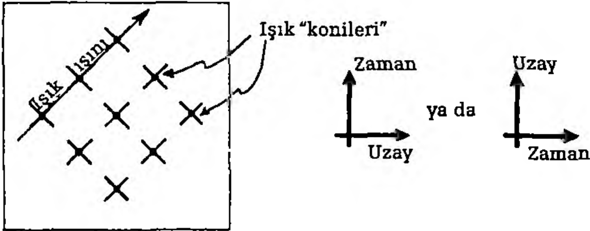
Şekil 7.16 İki boyutlu bir uzayzamanda uzay ile zaman arasında hiçbir fark yoktur; yine de tek bir kişi bile uzayın "akması" gerektiğini iddia etmez!
