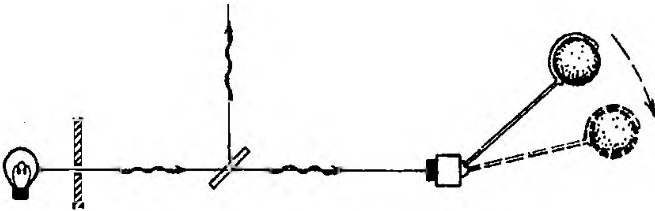
Şekil 6.4 Ölçüm kedi yerine küre şeklinde bir topağın basit hareketinden oluşabilirdi. Topak R'nin gerçekleşmesi için ne kadar büyük ya da kütleli olmak veya ne kadar uzağa hareket etmek zorundadır?
