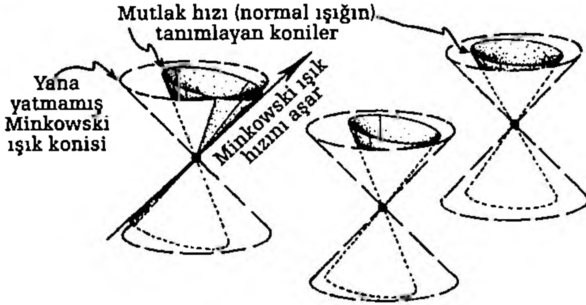
Şekil 4.4 Einstein'ın genel göreliliğine göre ışığın yayılması, Minkowski uzay çerçevesi içerisinde özel göreliliğin temel ilkesi olan sinyallerin Minkowski ışık hızından daha hızlı yayılamayacağı ilkesi çiğnenmeksizin "kıvrımlı bir ortamın" etkisi olarak düşünülemez.
