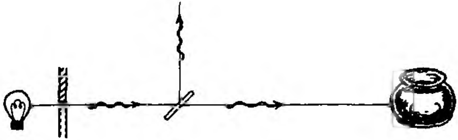
Şekil 6.7 Foton durumunun geçen kısmının bir topağı hareket ettirmek yerine sadece sıvı bir madde tarafından soğurulduğunu varsayalım.
