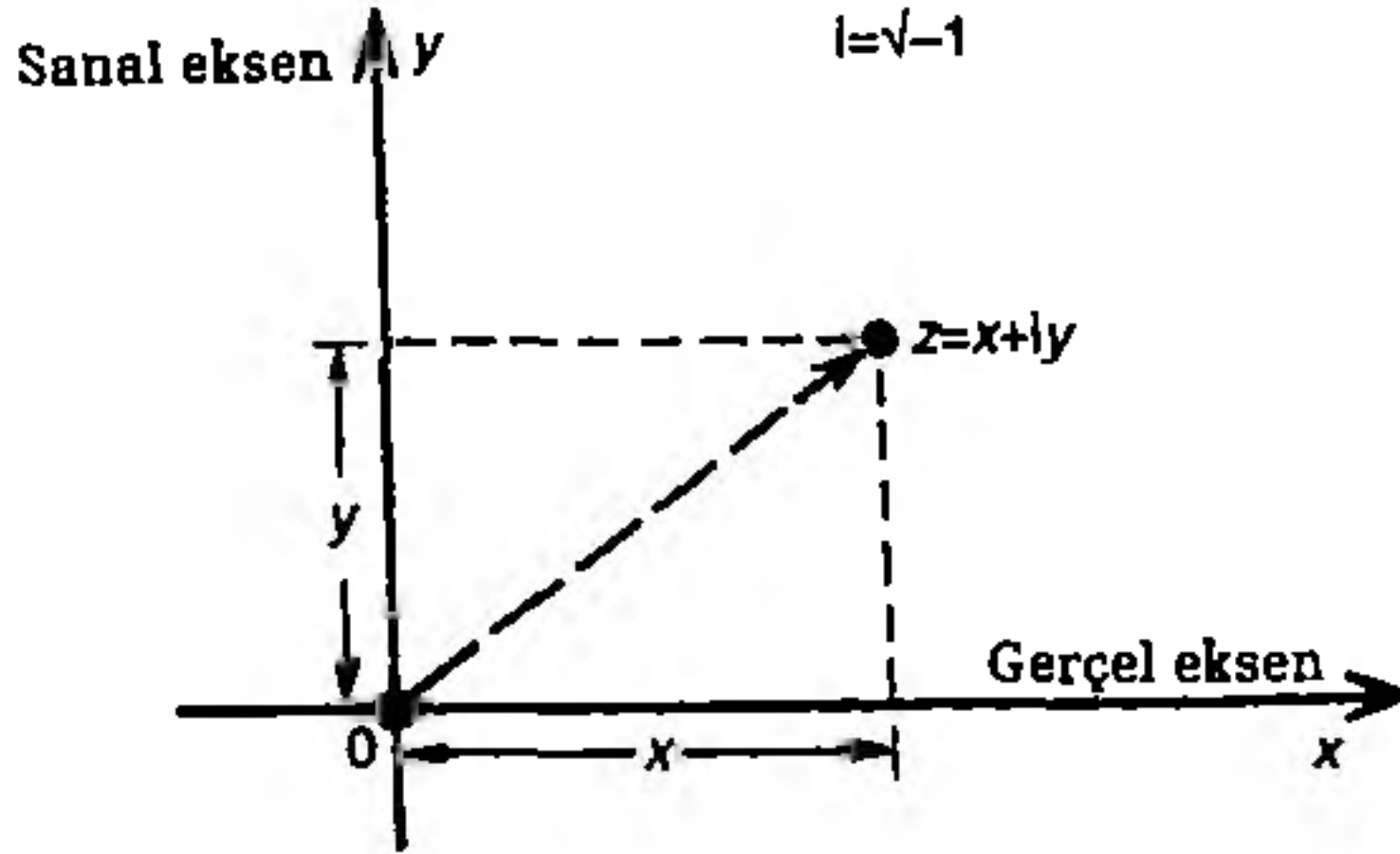
Şekil 5.16 Karmaşık bir sayının (Wessel-Argand-Gauss) karmaşık düzleminde gösterimi
