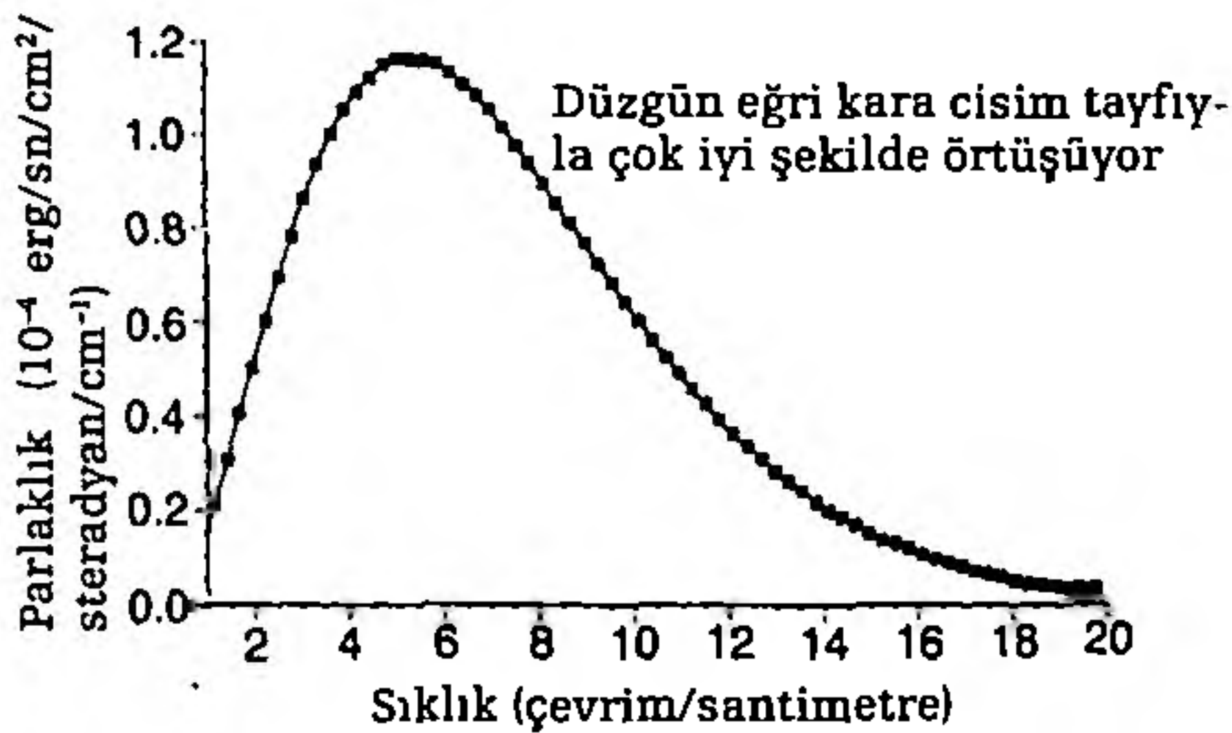
Şekil 4.12 COBE ölçümü ile Büyük Patlama ışımasının beklenen "termal" doğası arasındaki kesin örtüşme.
