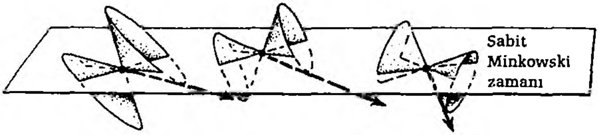
Şekil 4.5 İlkesel olarak ışık konisinin yan yatması ışık sinyallerinin Minkowski geçmişi içerisine yayılabileceği kadar uç olabilir.
