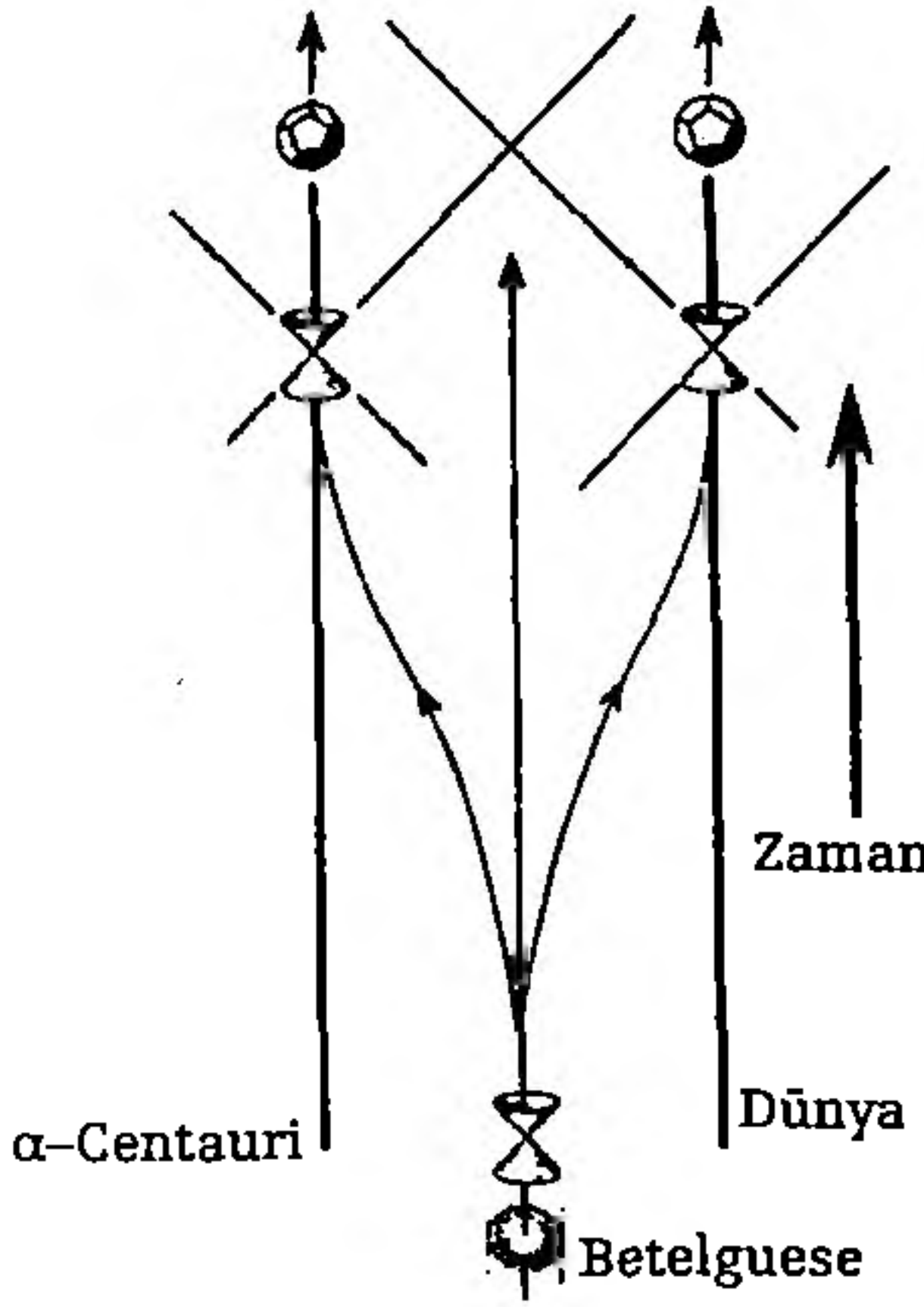
Şekil 5.5 İki dodekahedronun geçmişinin uzayzaman diyagramı. α-Centauri'ye ve dünyaya uzaysal olarak ayrılmış olaylarda ulaşırlar.
