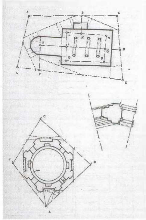
71. İstanbul Karasurlarında ölçme çalışması (1992)
