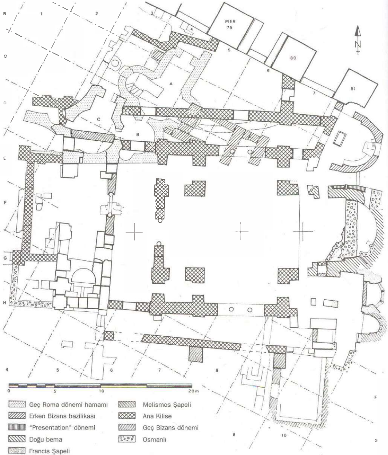
85. İstanbul Kalenderhane Camii ve çevresindeki kazıların analitik rölövesi (D.Kuban, C.Striker, 1972)
