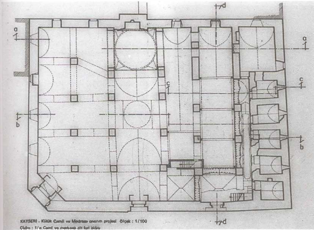
81. Planda kubbe ve tonoz izdüşümlerinin gösterilişi
