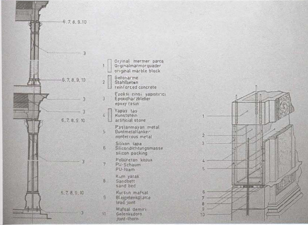
124. Efes, Celsius Kitaplığı: restorasyonda uygulanan taşıyıcı sistem şeması ve restorasyon sonrası genel görünüm (1990)
