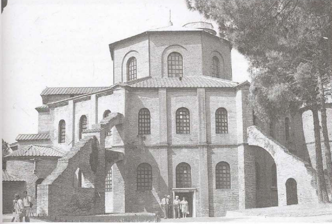
96. San Vitale Kilisesi duvarlarını destekleyen uçan payandalar (1982)
