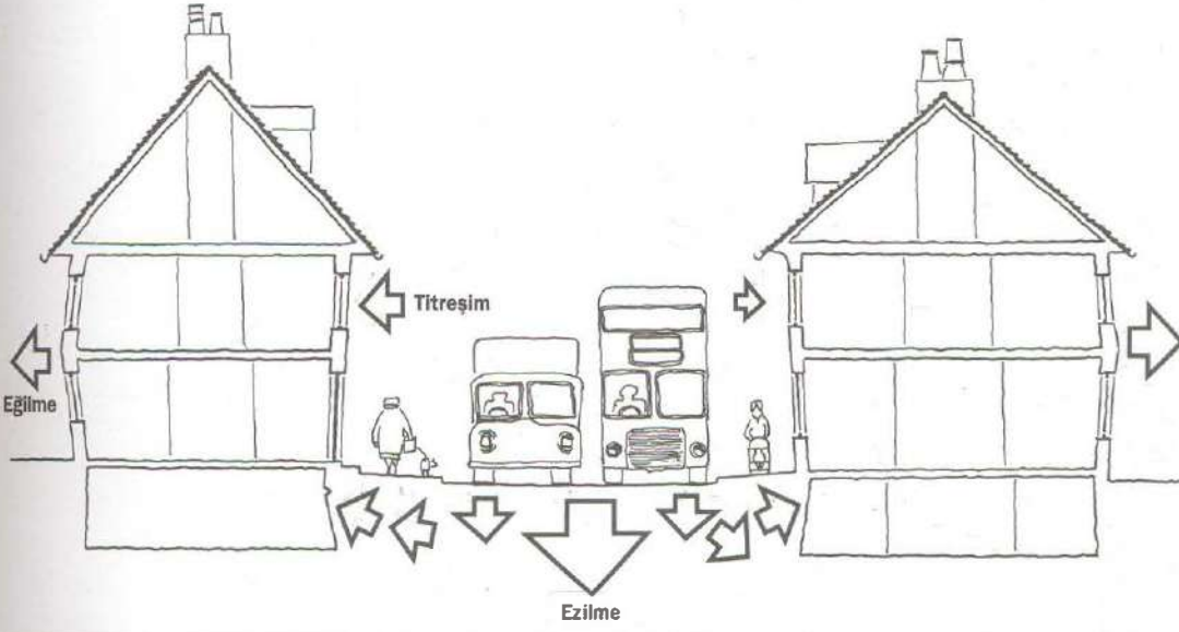
54. Ağır trafiğin çevredeki tarihi yapılara zararlı etkileri (D.Insall, 1975)
