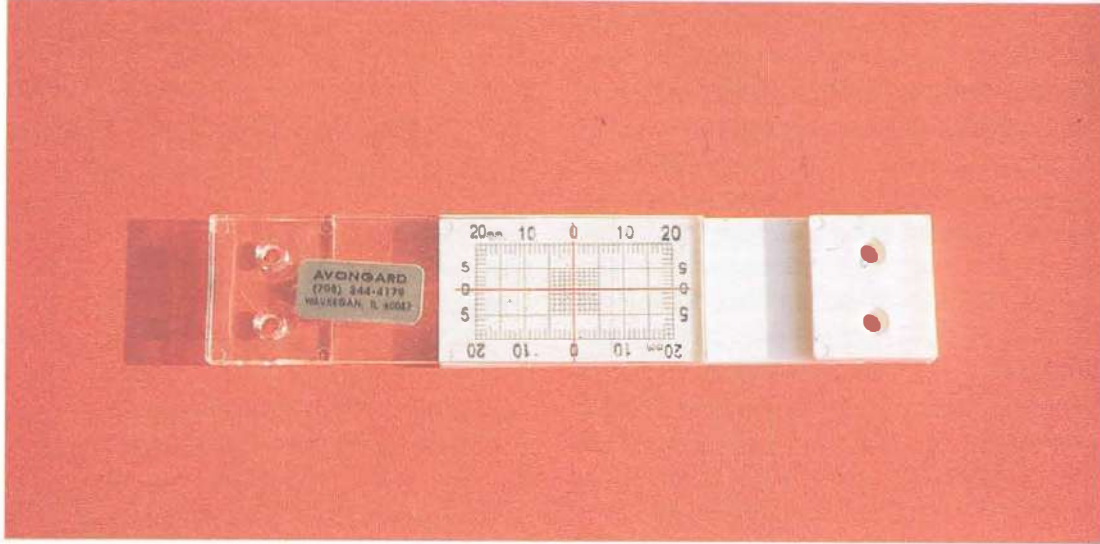
63. Çatlak monitörü
