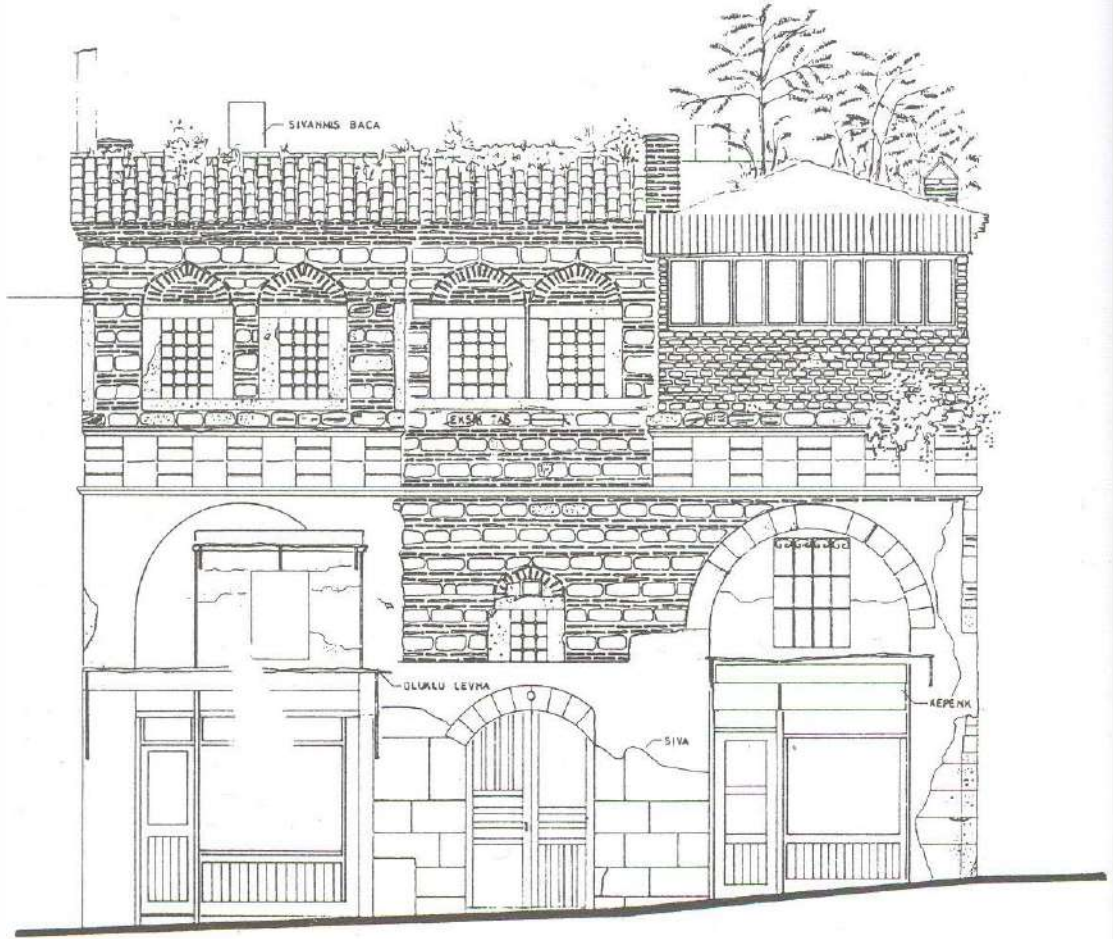
68. Eminönü, Emin Bey Hanı, kuzey cephesi rölövesi (F.Altan, 1989)
