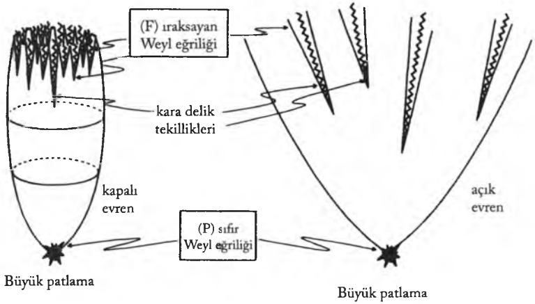
Şekil 2.5 Weyl eğrilik hipotezi: Başlangıç tekillikleri (büyük patlama), Weyl eğriliği sıfır olacak şekilde sınırlandırılmıştır. Buna karşılık, sondaki tekilliklerde, Weyl eğriliğinin ıraksayacağı bekleniyor.
