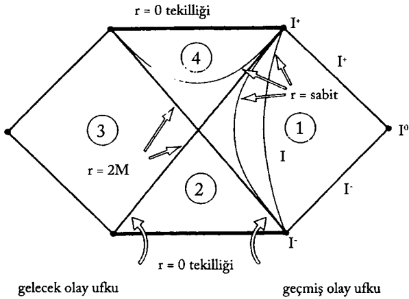
Şekil 3.4 Sonsuz zamanlı Schwarzschild karadelğine ait Carter-Penrose diyagramı
