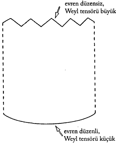
Şekil 5.13 Evrenin iki ucunu ayırdetmek amacına yönelik, Weyl tensörü hipotezi
