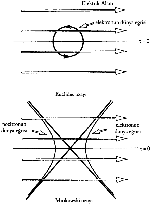
Şekil 3.11 Euclides uzayında elektron, elektrik alanında bir daire çizerek döner. Minkowski uzayında pozitif ve negatif elektrik yüklü bir çift parçacık birbirinden uzağa ivmelendirilir.
