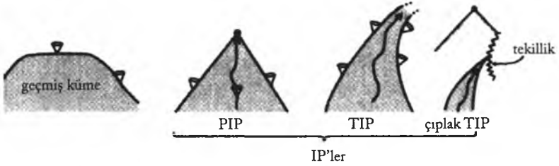
Şekil 2.2 Geçmiş-kümeler, PIP'ler ve TIP'ler
