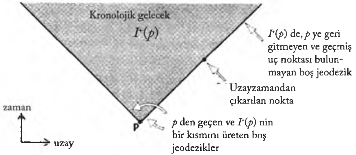
Şekil 1.1 p noktasının kronolojik geleceği
