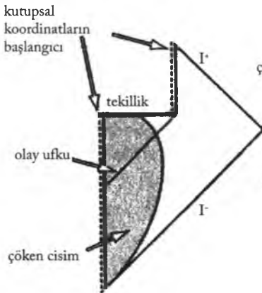
Şekil 7.5 Kara ve akdelikler için Carter-Penrose diyagramı
