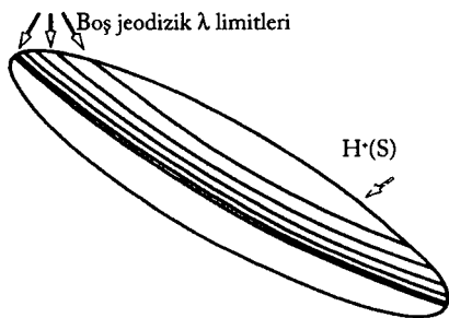
Şekil 1.12 Cauchy ufkunda, geçmiş veya gelecek uç noktaları olmayan, limit oluşan bir boş jeodezik vardır.
