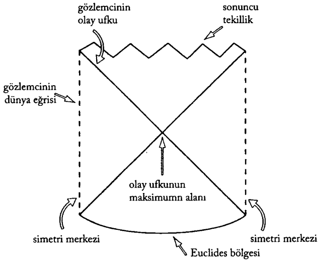
Şekil 5.12 Evren, bir gözlemci onun tamamını göremeden önce, sonundaki tekillik çökecektir.
