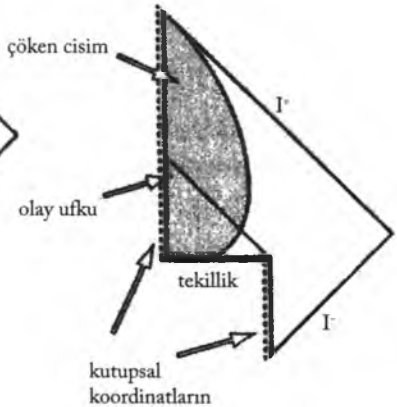
Şekil 7.5 Kara ve akdelikler için Carter-Penrose diyagramı
