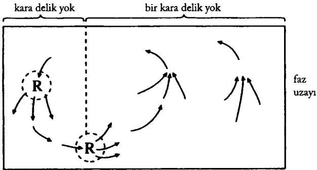
Şekil 4.4 Bir karadelik varsa, faz uzayında hacim kaybı gerçekleşir. R ile gösterilen dalga fonksiyonunun çökmesi nedeniyle, faz uzayı hacminin geri kazanılması, bunu dengeler.
