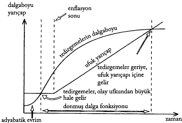
Şekil 5.10 Enflasyonda zamanın fonsiyonu olarak, dalgaboyu ve ufuk.
