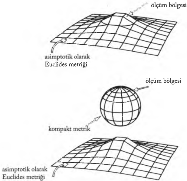
Şekil 5.2 Kozmolojik ölçümler sonlu bir bölgede yapıldığı için, iki tip asimptotik Euclides metriği dikkate alınmalıdır: bağlı olanlar (üstte) ve bağlı olmayanlar (altta).
