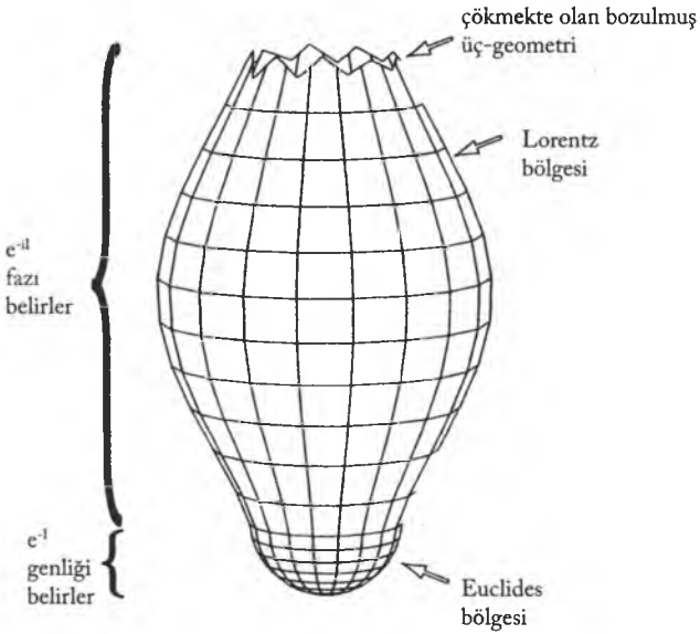
Şekil 7.4 Çökmüş olan üç-geometriye tünel sırasında; Euclides kısmı, üç-geometrinin dalga fonksiyonunun genişliğini belirtirken, Lorentz kısmı ise fazı belirler.
