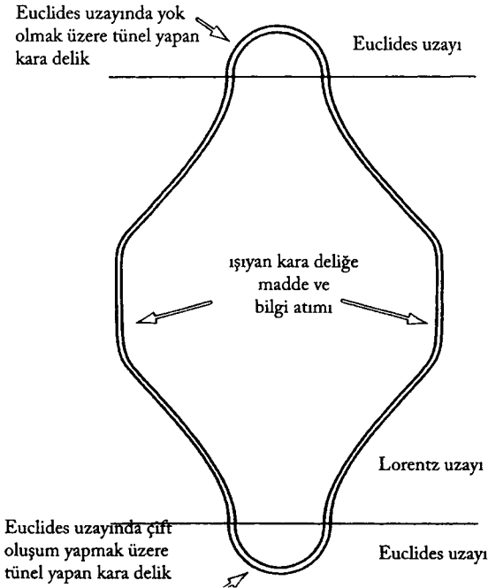
Şekil 3.16 Bir çift karadelikğin tünel olayı ile ortaya çıkması ve sonra gene tünel olayıyla yok olması
