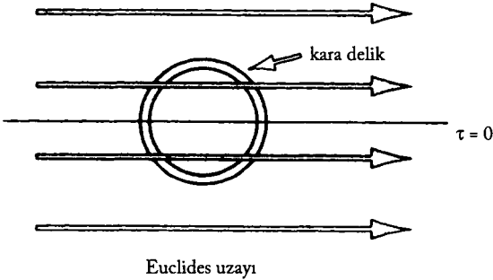
Şekil 3.14 Euclides uzayında bir çember üzerinde hareket eden yüklü karadeliğin.
