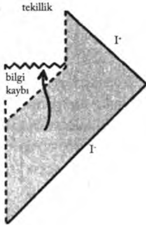
Şekil 4.3 Buharlaşan karadelik'in Carter diyagramı
