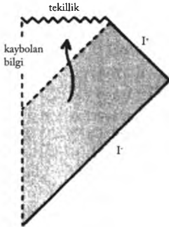
Şekil 4.2 Karadelğin çökmesine ait Carter diyagramı
