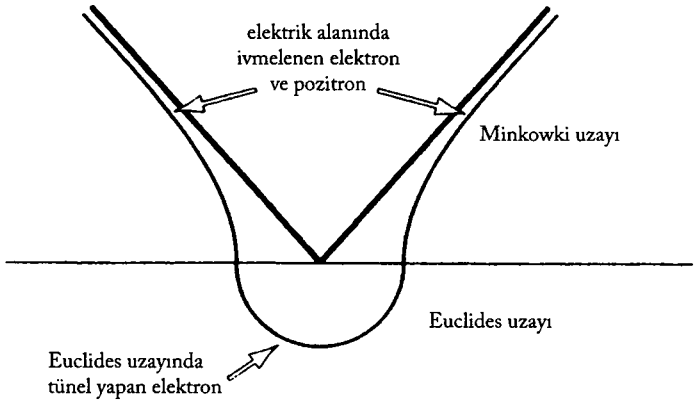
Şekil 3.12 Parçacık yaratılması, Euclides diyagramının yarısını, Minkowski diyagramının yarısına yapıştırarak belirtilir.
