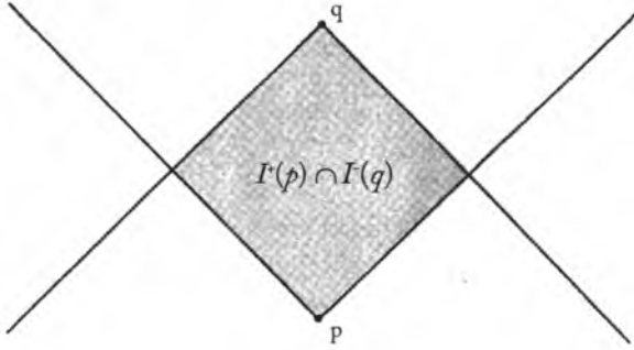
Şekil 1.5 p 'nin geleceği ile q 'nun geçmişinin kesişiminin kompakt kapanışı
