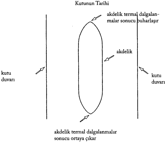
Şekil 7.3 Termal dalgalanmalarla ortaya çıkıp, kaybolan bir akdelik.
