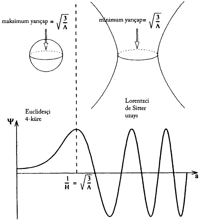
Şekil 5.6 S yarıçapının fonksiyonu olarak dalga fonksiyonu
