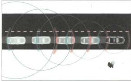
Doppler etkisi. Bir dalgalının kaynağı gözlemciye doğru hareket ettiğinde, dalgaboyları daha kısa görünür. Dalga kaynağı uzaklaştığında ise dalgaboyları daha uzundur. Bu duruma Doppler etkisi denir.
