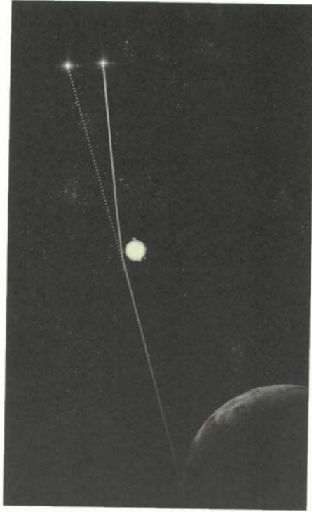
İşığın Güneş'in yakınında eğilmesi. Güneş doğrudan Dünya ve uzak bir yıldız arasında olduğunda, Güneş'in kütleçekimi alanı, o andaki konumuna bağlı olarak yıldız ışığının yönünü değiştirir.
