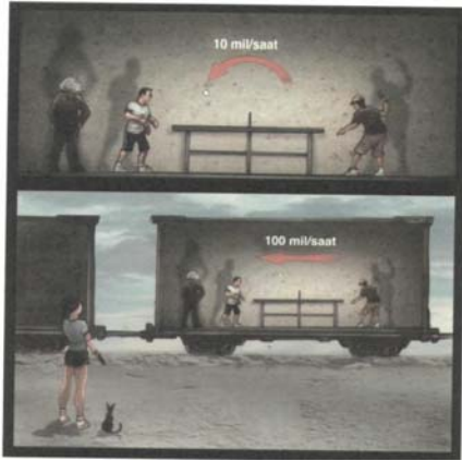
Pingpong topının farklı hızları.
