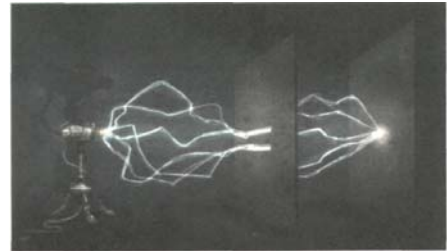
Elektron yolları.
