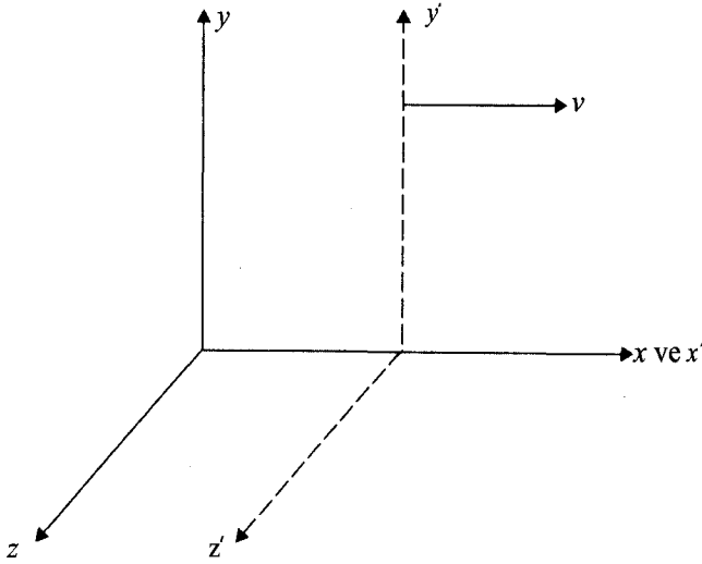
Şekil TN3.1 Görelî hareket halindeki iki uzaysal referans sistemi
