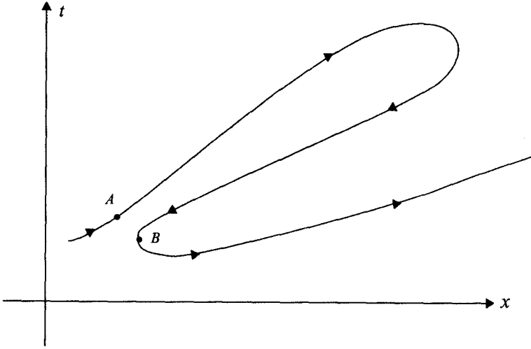
Şekil TN4.4 A noktasından B noktasına zaman içinde geriye hareket eden bir parçacığın konum-zaman eğrisi
