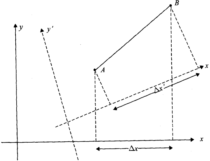
Şekil TN4.6 Döndürülmüş koordinat sistemleri
