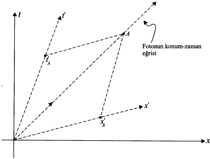
Şekil TN7.2 Fotonun dünya (konum-zaman) çizgisinin değişmezliği
