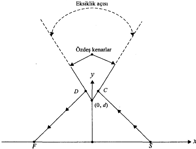
Şekil TN10.1 Uzay-zaman içinde, bir kozmik sicimin oluşturduğu eksiklik açısı
