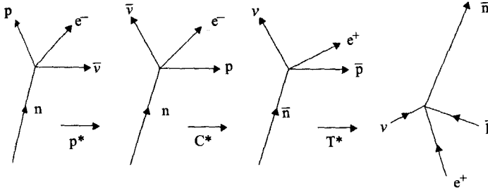
Şekil R2.1 TCP kuramı, anti nötronu öngörür.
