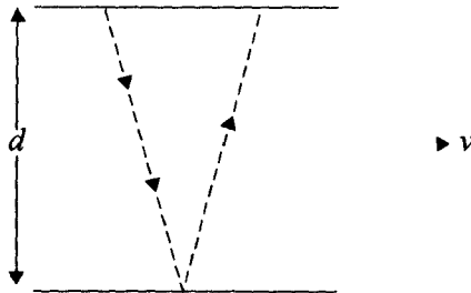
Şekil TN2.1 Foton saati
