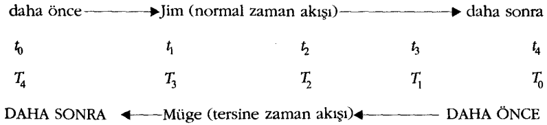
Şekil 3.1 Farklı dünyalarda saatin tersi yönünde akan karşıt zaman yönleri
