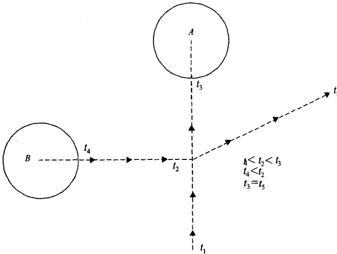
Şekil TN9.2 Bilardo toplarının dünyasında "dede torun paradoksu". A bilardo topu, tam merkezde duran zaman makinesi olan kurt deliğinin A ağzına yaklaşır ve içeri girmeden hemen önce I noktasından olaysız geçer. Top, sonra A ağzından içeri girer ve böylece I noktasından geçmek ve kendi genç hali ile çarpışmak için tam zamanında B ağzından geçmişte ortaya çıkar. Bu çarpma,
