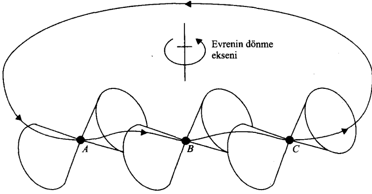
Şekil TN8.1 Döner bir evrenin yana yatmış ışık konileri. a. Evrenin dönme eksenini
