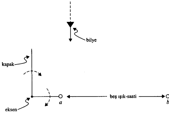
Şekil 4.1 Wheeler ve Feynman'ın paradoks makinesi
