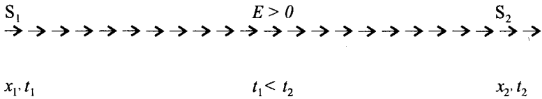
Şekil 4.2 Soğurulmadan sonra pozitif enerjili parçacığın dışarı yayılımı
