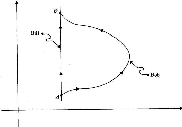
Şekil TN5.2 İvmeli ve ivmesiz hareket eden ikizlerin Dünya (konum-zaman) çizgileri
