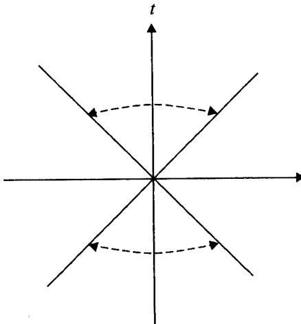
Şekil TN4.2 Fotonların konum-zaman eğrileri
