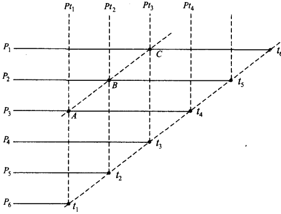
Şekil 3.5 Çok boyutlu zaman
