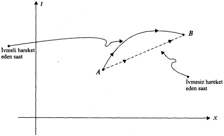
Şekil TN5.1 İki saatin konum-zaman eğrisi
