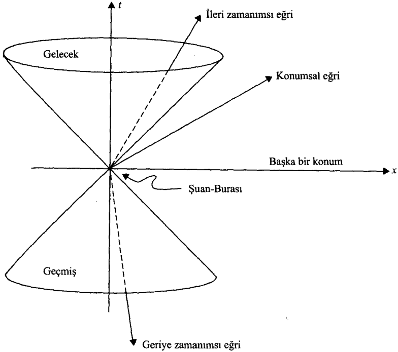
Şekil TN4.3 Konum-zaman eğrileri ve bir ışık konisi
