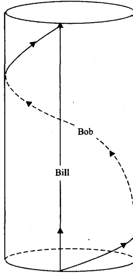
Şekil TN5.3 Silindirik bir uzay-zaman içinde ivmesiz ikiz paradoksu
