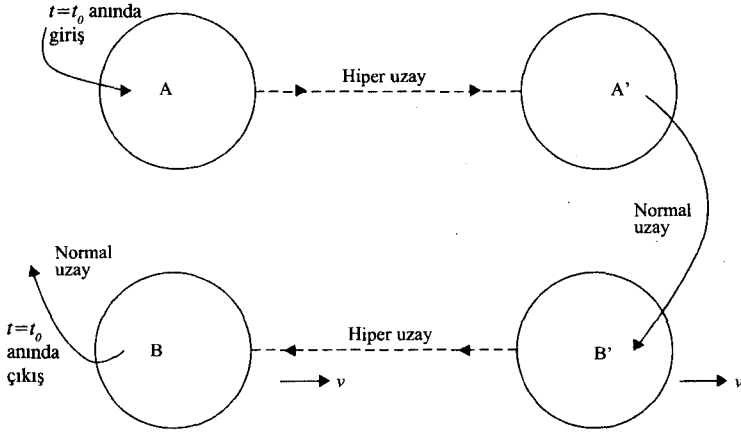
Şekil TN9.4 İki solucan delikli Roman biçimi zaman makinesi
