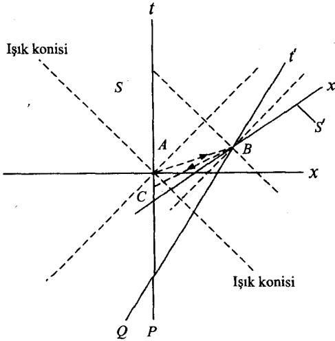
Şekil TN7.5 Bir IH nedensel paradoksu
