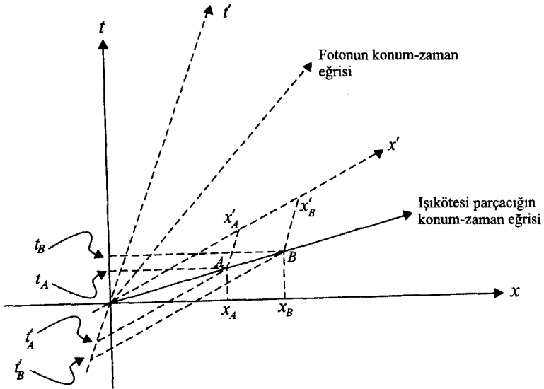
Şekil TN7.4 Işıktan daha yüksek hızlarda hareket eden parçacığın konum-zaman eğrisi
