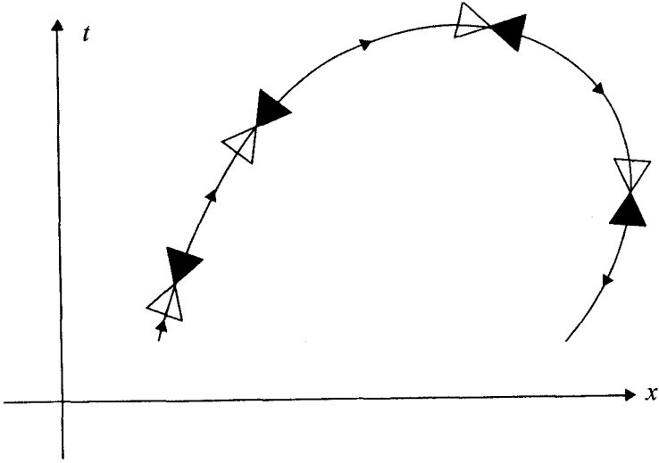
Şekil TN4.5 Eğilmiş ışık konileri. Gelecek konileri koyu renk ile gösterilmiştir.
