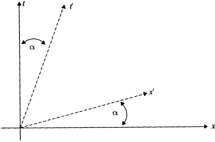
Şekil TN7.1 Göreceli hareket ile uzay-zaman koordinatlarının dönmesi
