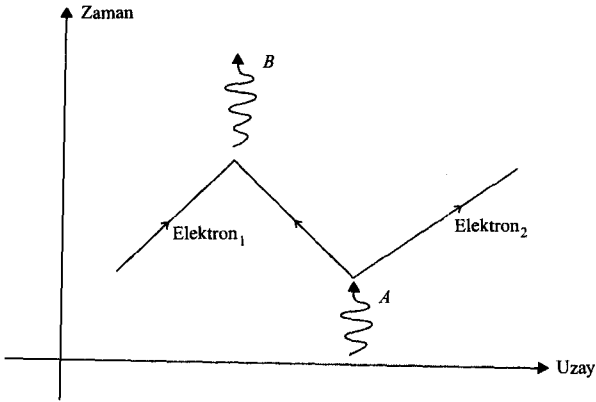
Şekil 3.3 Geçmişe zaman yolculuğu yapan anti-madde
