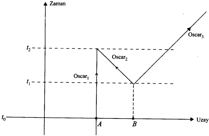
Şekil 3.2 Bir zaman gezgini ve konum-zaman eğrisi
