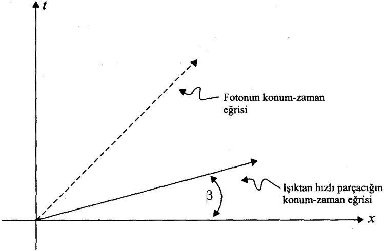
Şekil TN7.3 Işıktan hızlı bir parçacığın dünya çizgisi
