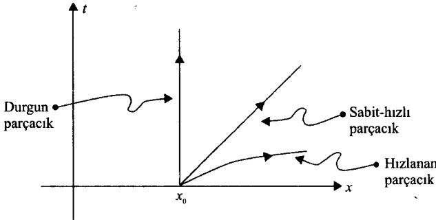
Şekil TN4.1 Üç ayrı parçacığın farklı konum-zaman eğrileri
