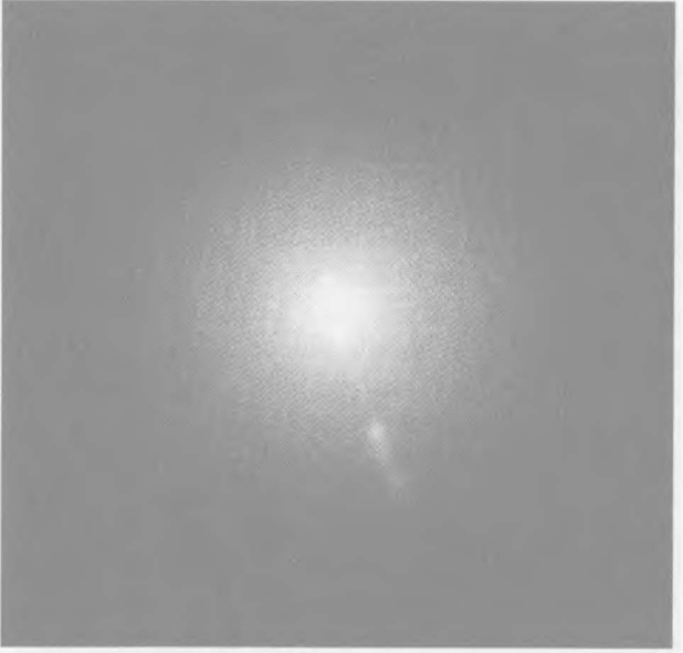
Şekil 15a. 500 ışık yılı uzaktaki M87 galaksisinin ( aynı zamanda Virgo A olarak da bilinir) görünür ışıkla çekilmiş fotoğrafı. Galaksinin merkezinden çıkan sönük, damlalara benzeyen çizgiye dikkat ediniz.
