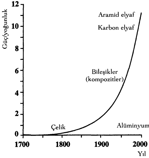
Şekil 5.1 Zamanın Bir Fonksiyonu Olarak Maddelerin Güç/Yoğunluk Oranında Gelişme ( \times 10^6 olarak)
