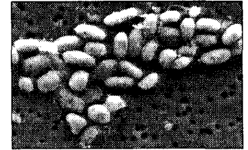
Şekil 6. GFAJ-1 bakterisinin mikroskopik görüntüsü.
