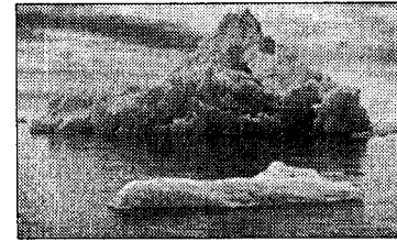
Şekil 40. Devasa boyutlardaki buzullar, sıvı suyun daha yoğun olması sayesinde yüzeyde kalırlar.
