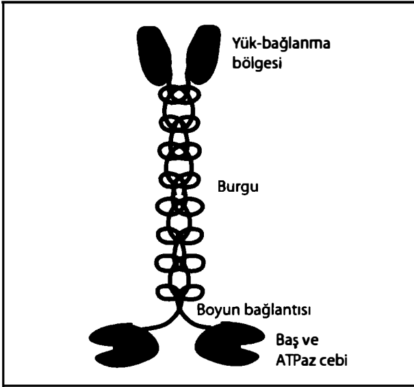
Şekil 7.4. Bir kinezin-1 molekülünün yapısı. Altta molekülün bir mikrotübül iplikçığı boyunca paytak paytak yürümekte kullandığı iki baş görülüyor. Her başta ATP'ye bağlanıp onu su kullanarak ayrıştırmaya yarayan bir cep vardır. Kısa boyumlu bir bağlayıcı iki başı bir arada tutar. Bunun üstünde yük bağlanma alanına uzanan çift kıvrımlı bir gövde bulunur.
