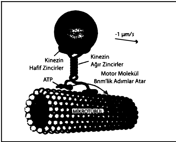
Şekil 6.8. Besinlerle dolu bir keseciği taşıyan bir kinezin moleküler motoru bir mikrotübül boyunca yürüyor. Moleküler motorun tamamının yüksekliği yalnızca yaklaşık elli nanometredir. © 1999 Robert A. Freitas Jr., www.nanomedicine.com . İzin alınarak kullanılmıştır.
