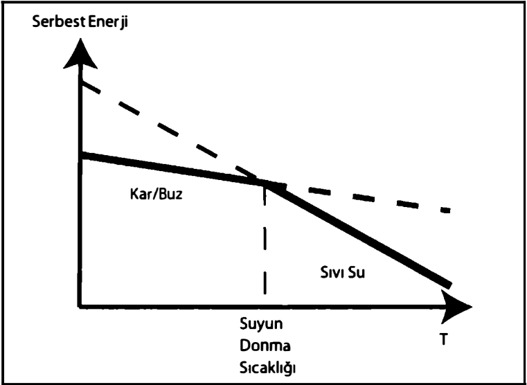
Şekil 3. 1. Sıvı haldeki suyun (siyah) ve buz ya da karın (gri) serbest enerjisinin sıcaklığa karşılık grafiği. Sıvı haldeki suyun entropisi daha yüksek olduğundan grafikte daha dik bir çizgi ile gösterilmiştir. Düşük sıcaklıklarda buz, sıvı haldeki sudan daha düşük serbest enerjiye sahiptir ve su donar. Yüksek sıcaklıkta sıvı haldeki su (yüksek entropiden ötürü) daha düşük serbest enerjiye sahiptir ve buz erir.
