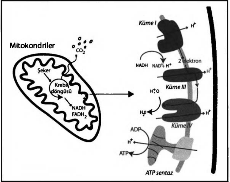
Şekil 7.10. Şeker halindeki kimyasal enerji mitokondride ATP halindeki enerjiye çevrilir. Bu, çok adımlı bir süreçtir. İlk, enerji NADH ve \text{FADH}_2 adlı moleküllere sabitlenir. Daha sonra bu moleküller, mitokondri zarındaki türlü makinelerce işlenir; bu makineler enerjiyi kullanarak hidrojen iyonlarını ( \text{H}^+ ) zarın bir yanından diğerine taşırlar. NADH küme I tarafından işlenirken \text{FADH}_2 küme II tarafından işlenir (gösterilmemiştir). Zarın bir tarafındaki hidrojen iyonu fazlalığı, ADP'yi yeniden doldurup ATP yapan ATP sentazı işletmek için kullanılır.
