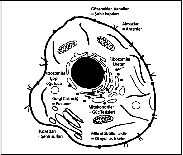
Şekil 7.1. Bir hayvan hücresinin taslağı.
