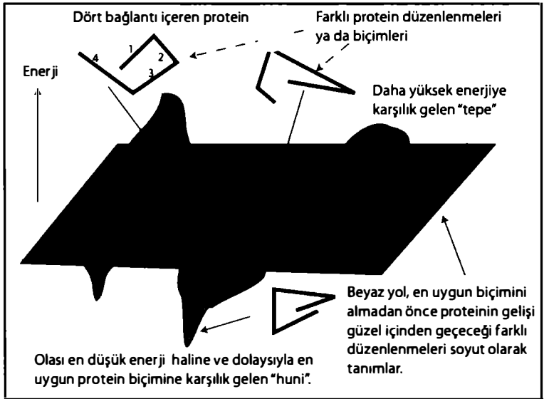
Şekil 4.4. Katlanan bir proteinin enerji yüzeyi.
