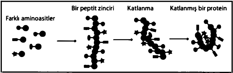
Şekil 4.3. Aminoasitler tek tip omurga ama farklı yan zincirleri olan moleküllerdir. Omurgalar bir peptit zinciri oluşturmak üzere peptit bağları ile birbirlerine eklenebilirler. Bu zincir, susevmez öğeleri (yıldızlar) merkezde ve susever olanlar dışarıda kalacak şekilde katlanarak kararlı bir yapıya ulaşana kadar moleküler fırtına tarafından itilip kakılır.
