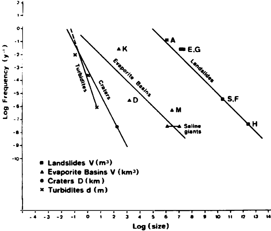
Şekil 8. Nadir olayların büyüklük/sıklık ilişkisinin 10 bazlı logaritmik bir grafikte gösterilmesi. Heyelânlar: A=Airolo, E=Elm, G=Goldau, S=Saidmarreh, F=Flims, H=Heart Mountain; Buharlaşma havzaları: K=Karaboğaz (Hazar Denizi), D=Ölü Deniz (İsrail ve Ürdün), M=Akdeniz (Mesiniyen Olayı).
