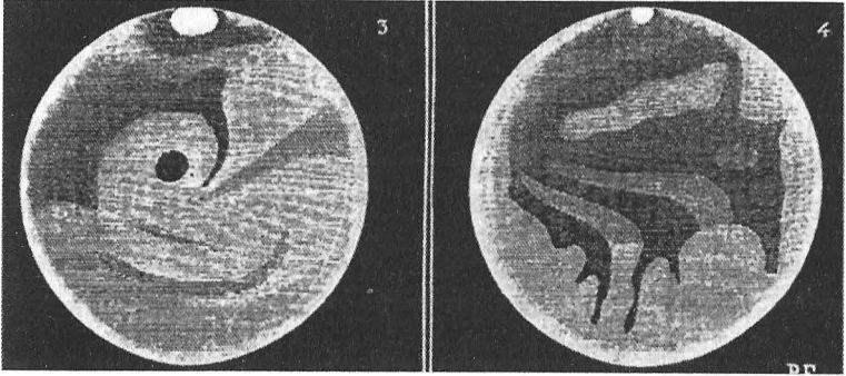
18 - Mars gezegeninin, 1877 yılı karşı-konumu sırasında, Camille Flammarion ve Giovanni Schiaparelli tarafından çizilen krokileri. (soldaki Flammarion'a, sağdaki Schiaparelli'ye ait). Kanal mitinin ortaya çıkmasına neden olan özellikle Schiaparelli'nin krokileridir. (C.Flammarion, L'Astronomie populaire "Güncel Gökbilim", Paris, 1880, s. 476)
