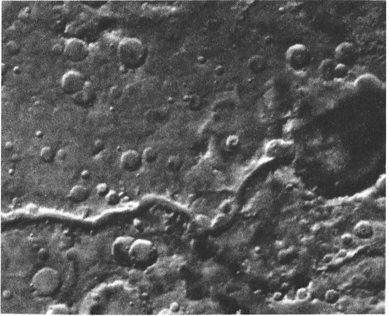
6.13- Geleceğin Mars sondaları, fosil içermeleri en fazla olası, akarsu ve göl çökelti alanlarına ineceklerdir. Gusev krateri (sağda) ideal bir alandır: Kraterlerle dolu eski platonun içinden kıvrılarak geçen derin Ma'adim Vallis vadisinin suları buraya boşalmıştır(Fotoğraf NASA/JPL/Caltech).
