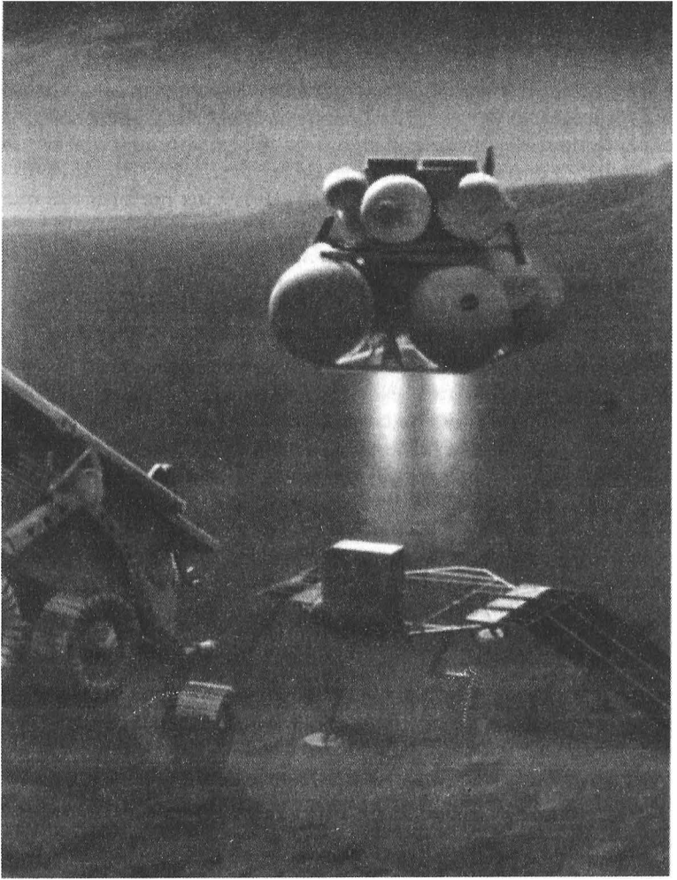
§6.12- Marsın keşfinde bir sonraki aşama: Örneklerin otomatik olarak dünyaya getirilmesidir. Öngörülen tarih 2007-2008 yıllarıdır. Yüz kadar küçük kaya ve yer örneği, bir kazıcı ile donatılmış arazi arabası (yakın planda solda) tarafından toplanacaktır. Yük, sondanın yörüngeye çıkma katına teslim edilince, dünyaya dönüş yolculuğu başlayacaktır. (Pat Rawling, NASA.)
