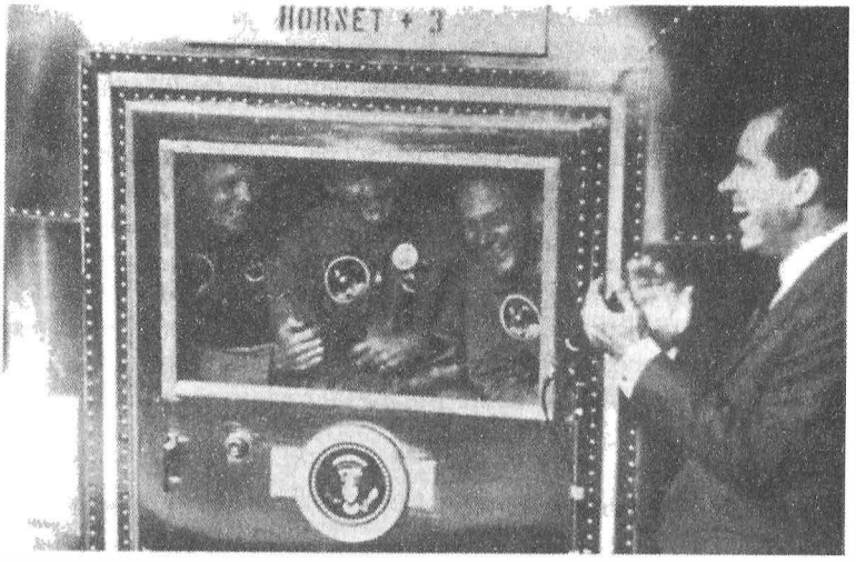
3.3.- Apollo II astronotları Ay'dan dönüşlerinde iki hafta boyunca, Ay'dan hiçbir yabancı bakteri taşımadıklarını doğrulayacak bir süre, karantinada tutuldular. Bu fotoğrafta Başkan Nixon, Armstrong'u, Collins'i ve Aldrin'i, Houston Laboratuvarı'na götürülmelerinden önce, camın arkasından tebrik ediyor. (Fotoğraf NASA)
