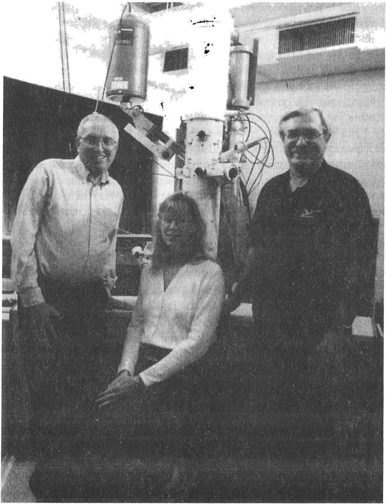
4.7- ALH 84001 göktaşında biyolojik bir etkinliğin yaşandığı varsayımını ortaya çıkaran üç araştırmacı. Soldan sağa: David McKay, Kathie Thomas-Keptra ve Everett Gibson. Arkalarında görünense, otuz bin kez büyültme ile minerallerin incelenmesini sağlayan transmisyonlu elektronik mikroskop (TEM). (Fotoğraf NASA/JSC)
