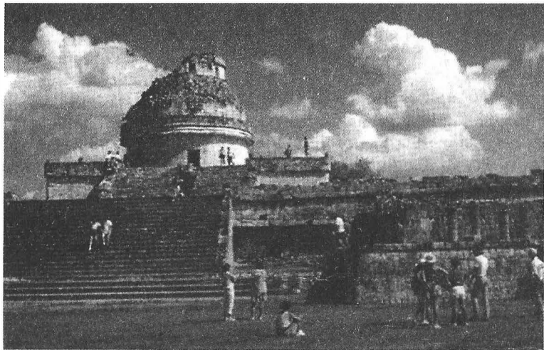
1.1- Meksika'da, Chichen Itza harabelerindeki Maya gözlemevi. Yıldızların gözlemlenmesi, birçok uygarlığı, evrende yaşam sürdüren diğer dünyaların varlığı hakkında kendi kendilerine soru sormaya itti. (Fotoğraf yazara aittir.)
