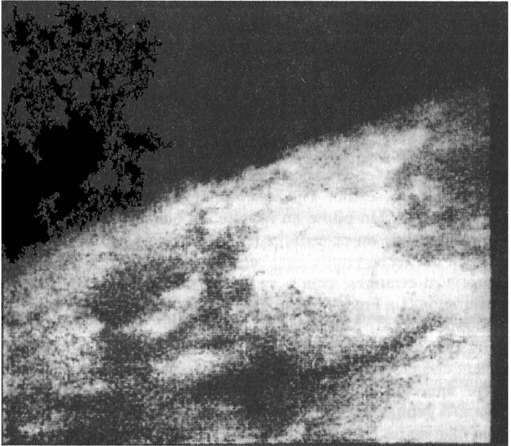
2.5.- Bir uzay gemisinden çekilen ilk Mars fotoğrafı. 15 Temmuz 1965'te Mariner-4, Elysium dağ kolunun çapraz fotoğrafını çekerek, yirmi iki görüntü alma salvosunu başlattı. Alan genişliği 350 kilometredir. Yuvarlak gölgeler kraterleri göstermektedir. (NASA/NSSDC)
