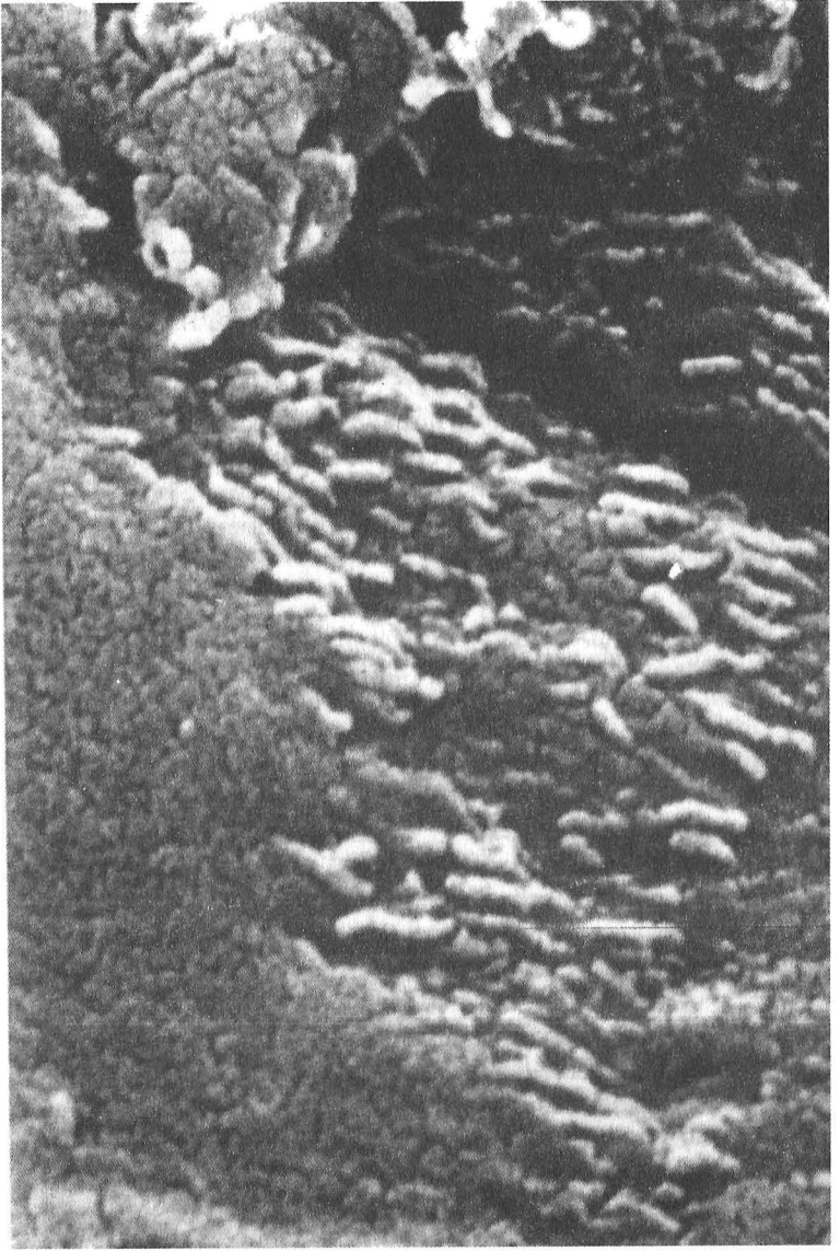
4.9- Mars göktaşı ALH 84001'in mikroskop altında görünüşü. Yumurta biçiminde küçük şekiller, et kurtları gibi karbonat mineralinin yüzeyine çıkıyor. Fosil mezarlığı mı? Ya da organik olmayan mineralin sopamsı aşınması mı? (Fotoğraf NASA/JPL)
