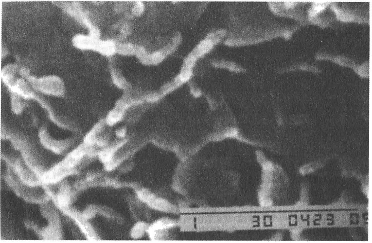
5.6- Sicily Volkanı killeri, mikroskop altında, fosilleşmiş küçük bakteriler olarak bilinen solucan biçiminde yapılar sergilerler. Bunlar Marslı mikrofosil oldukları tahmin edilen şekillerle aynı boyda ve biçimdedir. Sağda alttaki ölçü cetveli 1 mikrometre boyundadır. (Fotoğraf NASA, Robert Folk'a teşekkür ederiz.)
