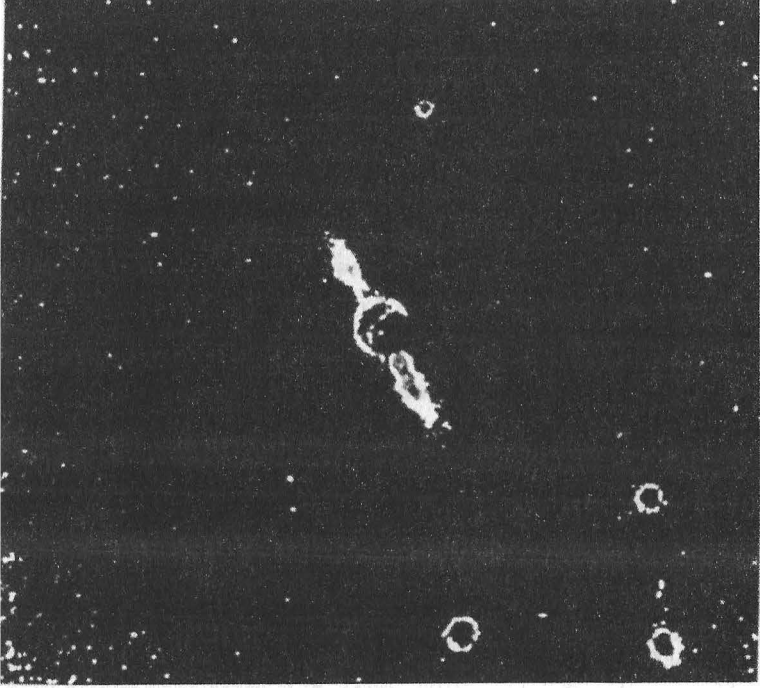
8.4- Beta Pictoris yıldızı bir toz diskiyle çevrili durumda (solda yukarda ve sağda aşağıda "parıldayan kulaklar" görülüyor.) Gözlem alanının merkezinde yer alıyor. Şili Campanas gözlemevinde Carnegie Enstitüsü'nün teleskobuyla elde edilen bu fotoğraf, Güneş dışında başka yıldızların da gezegen sistemlerini barındırabileceğinin ilk kanıtlarındandır. (Carnegie Enstitüsü, fotoğrafın işlenmesi JPL ve Arizona Üniversitesi, Lunar ve Planetary Enstitüsü koleksiyonu.)
