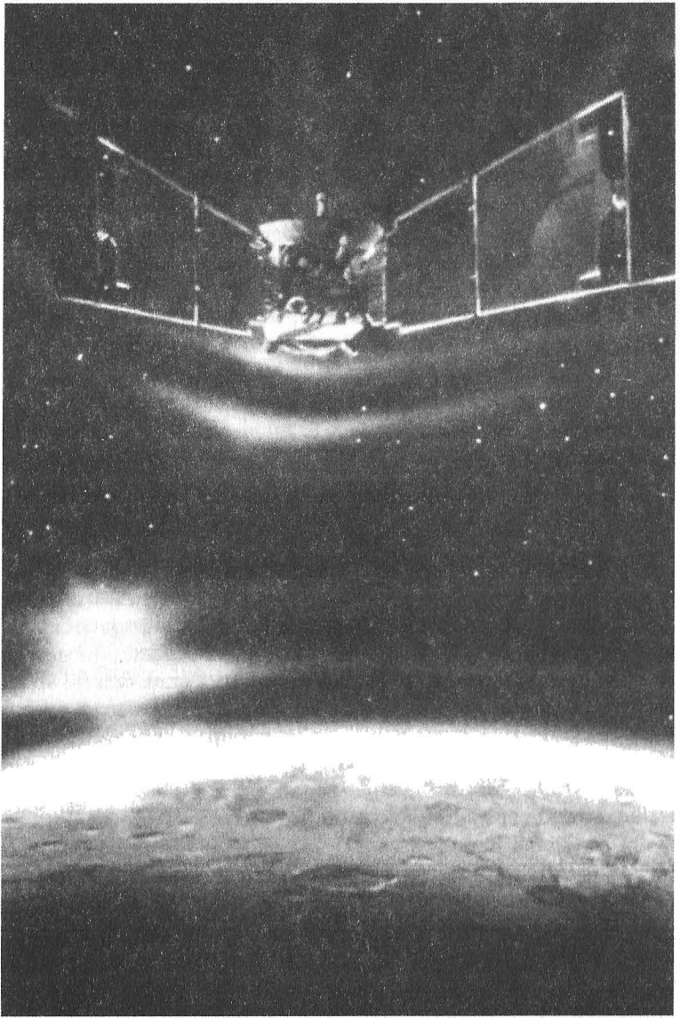
6.10- Global Surveyor sondasının Mars yörüngesindeyken sanatçı taafından yorumlanması. Uzay gemisi güneş panolarını hava freni olarak kullanıyor: Hız azalması ona, propergol yakıtı kullanmadan “kendiliğinden” yörüngesini düzeltmeyi sağlıyor. (Pat Rawling, NASA.)
