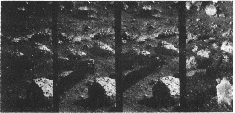
3.9.- Kapaklı bir küreği bulunan uzaktan kumandalı kol, Mars'ta iş başında. Kolun örneği yerden aldıktan sonra bıraktığı taze iz kolaylıkla fark ediliyor. (Fotoğraf, Viking NASA\JPL.)
