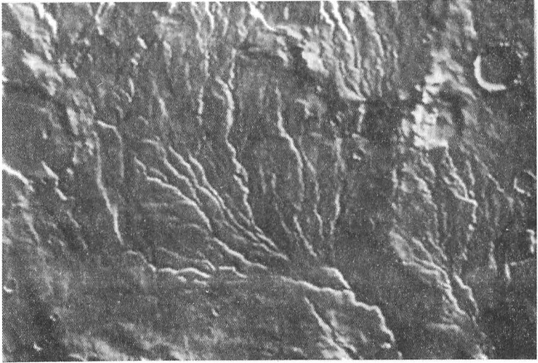
2.13.- Mars'ın güney yarımküresinde birçok su yolu yüksek volkanik platolardan aşağı iner. Bu fotoğrafta vadiler, bir yaprağın damarları gibi, fotoğrafın sağ alt köşesine doğru yöneliyor. Bu çok eski erozyon yağmur sularının yüzeyde sel gibi akması ya da erimiş yeraltı suyunun yeryüzüne çıkarak yüzeyi çökertmesi sonucunda oluşmuştur. (Fotograf Viking, NASA, Ay ve Gezegenler Enstitüsü'nden Brian Fessler'in değerlendirmesi.)
