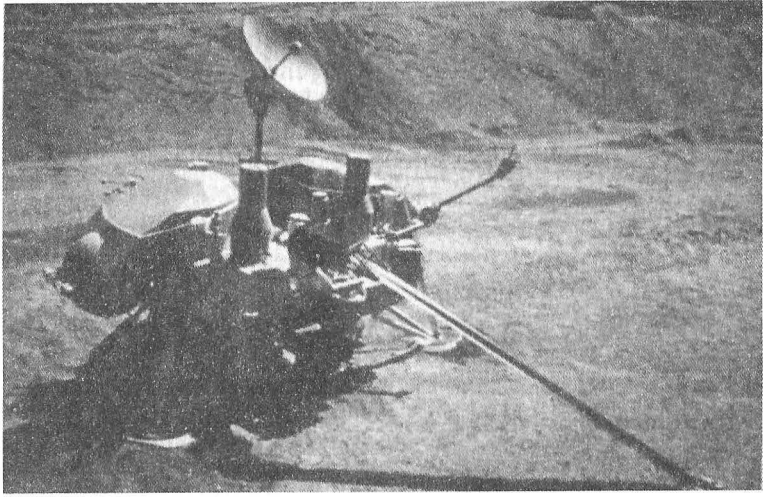
3.6.- Dünya üstünde fotoğrafı çekilen Viking sondası. Solda yakıt depolarının bulunduğu kapak. Merkezde yüzey örneğini almakla ve onu arka bölümdeki, iki görüntü alma çıkmasının ortasında yer alan dağıtım hunisine koymakla görevli teleskopik kol. En üstte Dünya ile iletişim anteni. Sağda, meteoloji aletlerinin direği. (Foto NASA).
