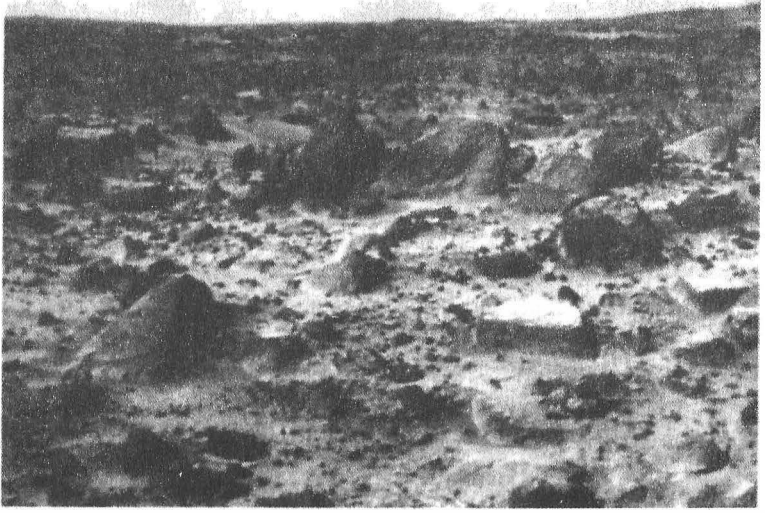
6.8- Rock Garden (Kayalar bahçesi). Bu büyük kayaların oluşturduğu yığıntı Sojourner'ın başlıca hedefiydi ve otomobil oraya Ağustos ayı sonunda ulaştı. Yakın planda, solda, köpekbalığı yüzgecine benzeyen kayanın adı Shark. Sağında açık renk tozla kaplı olanının adı Flat Top. İkinci plandaki kayalar güçlü bir akıntının etkisiyle sıralanmış gibiler. (Fotoğraf NASA/JPL/ Caltech.)
