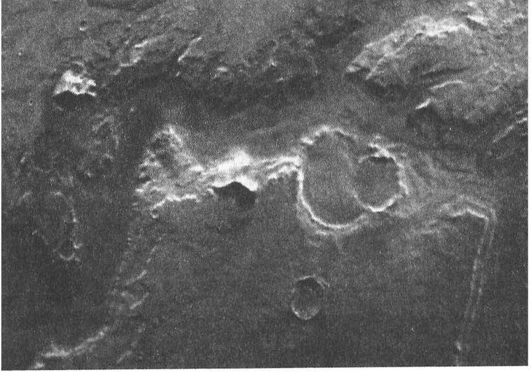
2.14. Mars'ta bir sel baskını kanalı. 972 kilometre uzunluğunda ve binlerce metre genişliğindeki Reull Vallis, bir yeraltı buzunun çözülmesiyle oluşan çamur ve su fırtınasını yönlendirmiş olmalı. Vadinin kenarları sayısız teras izi (özellikle sağda aşağıda) ve büyük bir olasılıkla da kum kumulları olan koyu çözelti plajları (yukarda solda) göstermektedir. (Fotograf Viking, NASA/JPL.)
