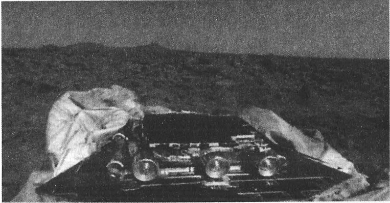
6.4- Pathfinder sondası 4 Temmuz 1998'de Mars yüzeyinde görünüyor. Platformun üstünde duran Sojourner kızıl gezegene inme emirini bekliyor. Daha önce çıkırıklar hava yastıklarını sarmak ve çevreyi düzenlemek için harekete geçecekler. Ufukta ikiz Twin Peaks tepeleri yeralıyor. (Fotoğraf NASA/ Caltech.)
