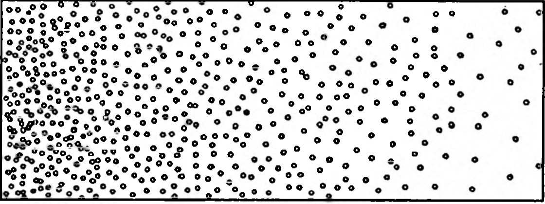
Şekil 4. Konsantrasyonu değişen bir çözeltide soldan sağa difüzyom.
