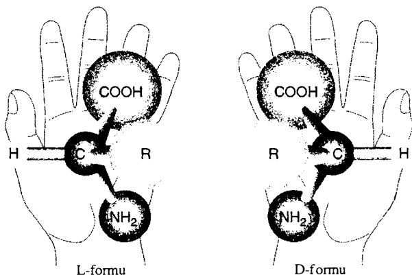
Şekil 1. Kiral cisimlerle ilgili el analojisi. Bir cisim, ayna görüntüsü kendi üzerine aynen yerleştirilemiyorsa kiraldir.
