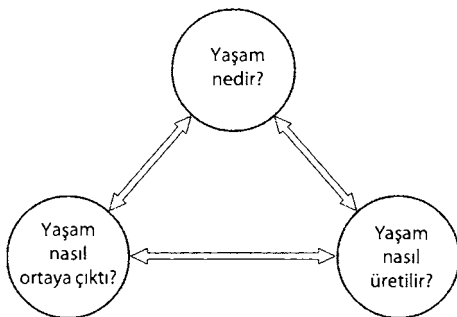
Şekil 5. Biyolojide bütüncü anlayışı yöneten üç temel soru.
