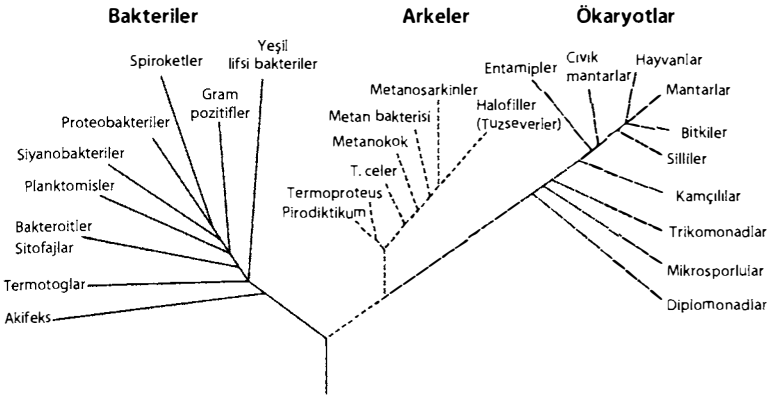
Şekil 4. Yaşamın üç âlemini –Bakteriler, Arkeler ve Ökaryotlar– gösteren, ribozomal RNA dizilim analizine dayalı yaşam ağacı.
