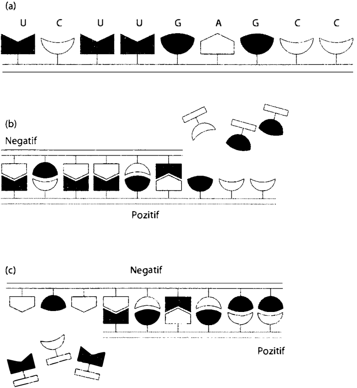
Şekil 3. (a) A, U, G ve C nükleotid yapıtaşlarının bir diziliminden oluşan RNA molekülünün şematik temsili. (b) RNA zincirinin kendisinin tamamlayıcı bir kopyasının oluşturulmasını tetiklediği sürecin temsili şeması. (c) Tamamlayıcı RNA kopyasının, orijinal RNA'nın kopyasının oluşumunu tetiklediği (negatiften pozitif) sürecin şematik gösterimi.
