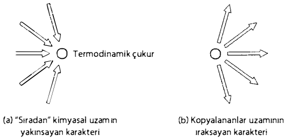
Şekil 7. "Sıradan" kimyasal uzamdaki (yakınsayan) ve kopyalananların uzamındaki (ıraksayan) dallanma örüntülerinin şematik gösterimi.
