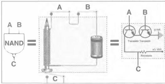
Görsel 2.6: NAND kapısı A ve B bitlerini girdiler olarak alır ve A=B=1 ise C=0 , değilse C=1 kuralına göre, C bitini çıktı olarak verir. Pek çok fiziksel sistem NAND kapısı olarak kullanılabilir. Ortadaki örnekte, anahtarlar 0=açık ve 1=kapalı olacak şekilde bitler olarak yorumlanabilir ve A ile B anahtarlarının ikisi de kapalıyken bir elektromıknatıs C anahtarını açar. En sağdaki örnekte, voltajlar (elektiriksel potansiyel) 1=5 volt ve 0=0 volt olacak şekilde ayarlanmıştır, A ve B kablolarının ikisi de beş voltta iken iki transistör elektrik iletir ve C kablosu yaklaşık sıfır volta düşer.
