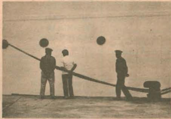
SEMH YOLACAN
