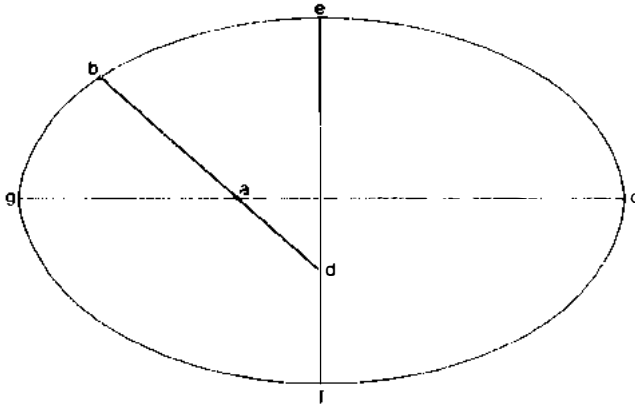
Şekil 4.1 Elipsin elipsograf ile çizimi. dab elipsografı, a , gc doğru parçasını ve d de ef doğru parçasını takip edecek biçimde hareket eder. Elipsografın bd uzunluğu elipsin büyük çapının yarısına, ab uzunluğu da küçük çapının yarısına eşittir.
