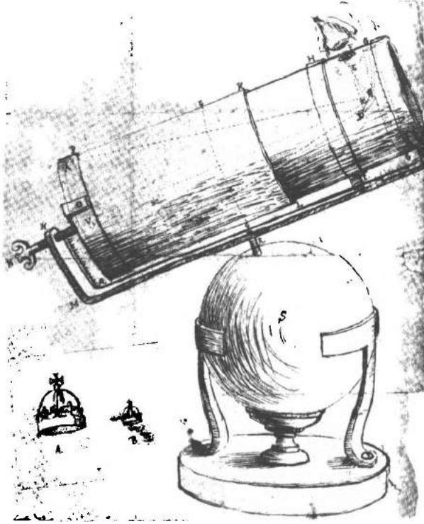
Şekil 6.9. Newton'ın teleskobunun Kraliyet Derneği tarafından yapılmış çizimi. Çizimdeki iki taç aynı cisim; tacın üzerindeki süslemelerin, 300 fit [yaklaşık 91 metre] uzaklıktan Newton'ın telekobuyla (A) ve 25 inç [yaklaşık 63 santimetre] uzunluğundaki bir mercekli teleskopla görünüşü (B). (Kraliyet Derneğinin izniyle.)
