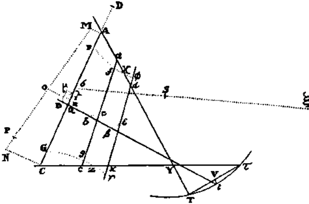
Şekil 10.9. Peş peşe yakınsamalarla bir kuyruklu yıldızın yörüngesinin hesaplanması.
