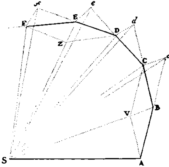
Şekil 10.1 Daha önce De motu 'da yer aldığı biçimiyle Principia 'nın 1. Önermesinin çizimi. Merkezci kuvvet B, C, D ve E'ye "aynı anda büyük bir itmeyle" etki ederek cismi doğrusal yolundan döndürür.
