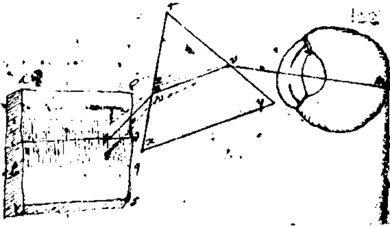
Şekil 5.4. Işığın farklı kırılabilirliğine ilişkin Newton'ın ortaya koyduğu ilk görüş. (Cambridge Üniversitesi Kütüphanesi Kurul Üyelerinin İzniyle)
