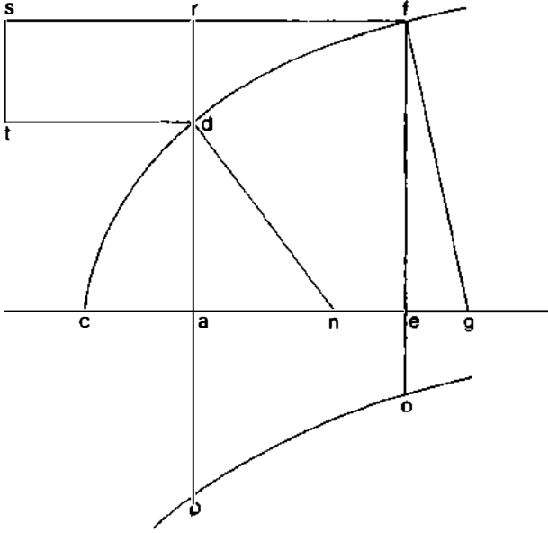
Şekil 4.10. Kalkülüsün temel teoremi.
