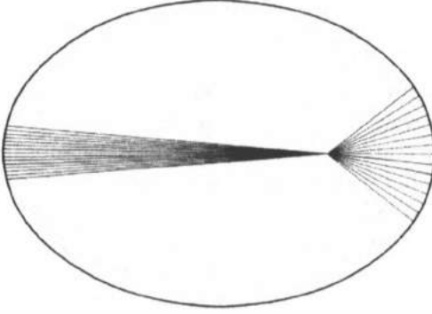
Şekil 1.3. Kepler'in, yarıçap vektörü tarafından taranan alanın zamanla orantılı olduğunu söyleyen ikinci yasası. Elipsin dışmerkezliği (odaklar arasındaki uzaklığın büyük eksen uzunluğuna oranı) bir hayli abartılmıştır.
