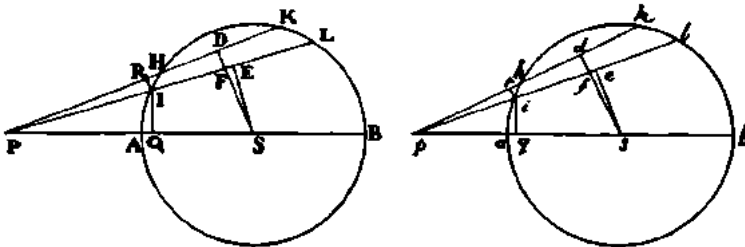
Şekil 10.4. Homojen bir küresel kabuğun dışındaki bir parçacığa uyguladığı çekim.
