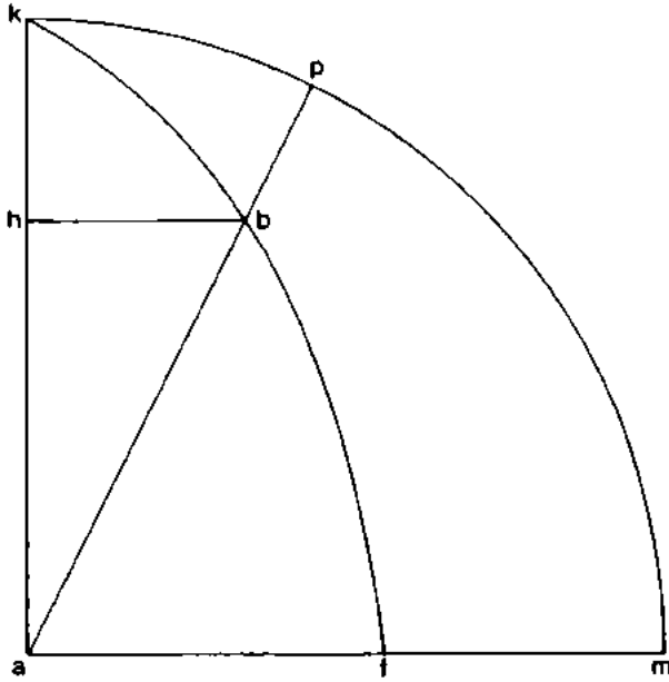
Şekil 4.16. ap yarıçapının döndürülmesi ve hb doğru parçasının hareketiyle oluşturulan kbf eğrisi.
