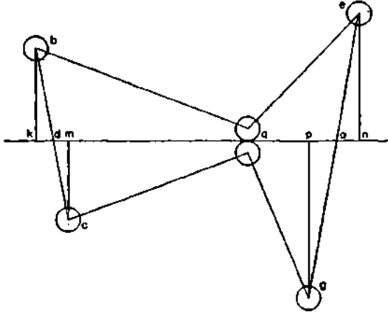
Şekil 5.1. Tamamen esnek iki cismin belli bir açı yaparak çarpışması. (Westfall, Force in Newton's Physics [Newton Fiziğinde Kuvvet])
