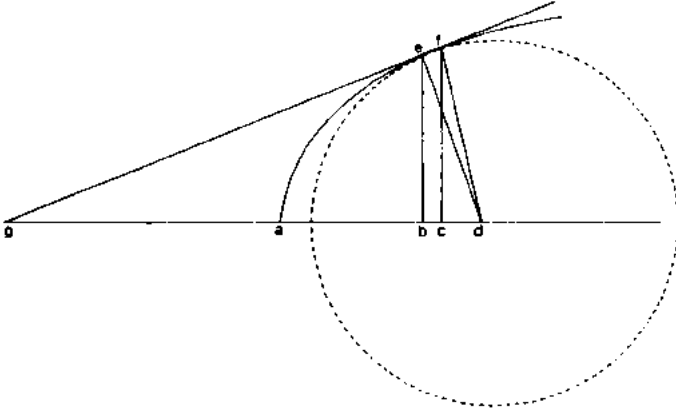
Şekil 4.14. Teğetlere yeni yaklaşım.
