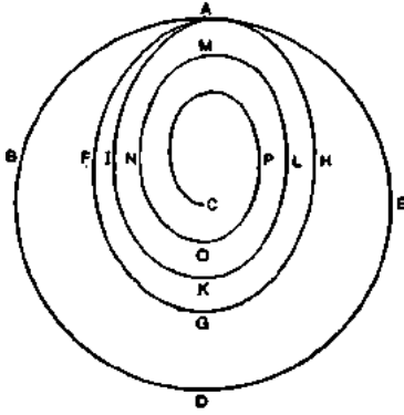
Şekil 9.4. AFGH dirençle karşılaşmayan bir cismin izlediği yoldur. İçteki AIKL-MNOPC sarmalı cismin dirençle karşılaştığı bir ortamdaki yolunu gösteriyor. (Westfall, Force in Newton's Physics 'ten.)
