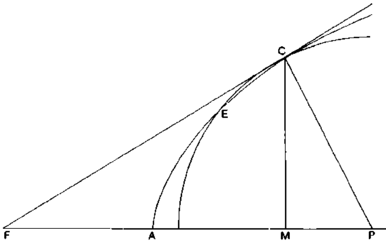
Şekil 1.6. Descartes'ın teğetleri bulma yöntemi. E ve C noktaları tek bir noktada birleştiğinde iki kökü bularak MP normal tabanının uzunluğunu buldu, aslında AEC parabolüne C noktasında teğet olan bir çemberin AM eksenı üzerindeki merkezi olan P noktasının geometrik yerini bulmuş oldu. Parabole C noktasındaki teğet elbette PC normaline diktir.
