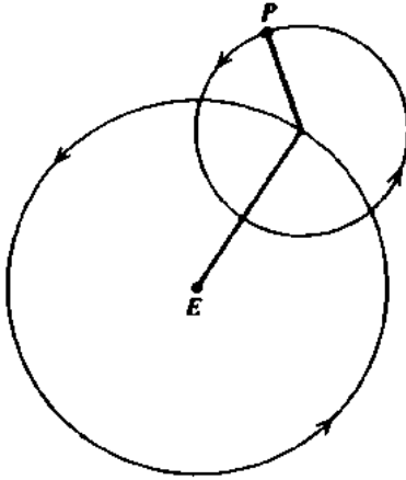
Şekil 1.1. Ptolemaios sistemi gezegenlerin geriye doğru olan görünür hareketlerini açıklamak için merkezi bir taşıyıcı çember üzerinde bulunan bir ilmekten yararlanır.
