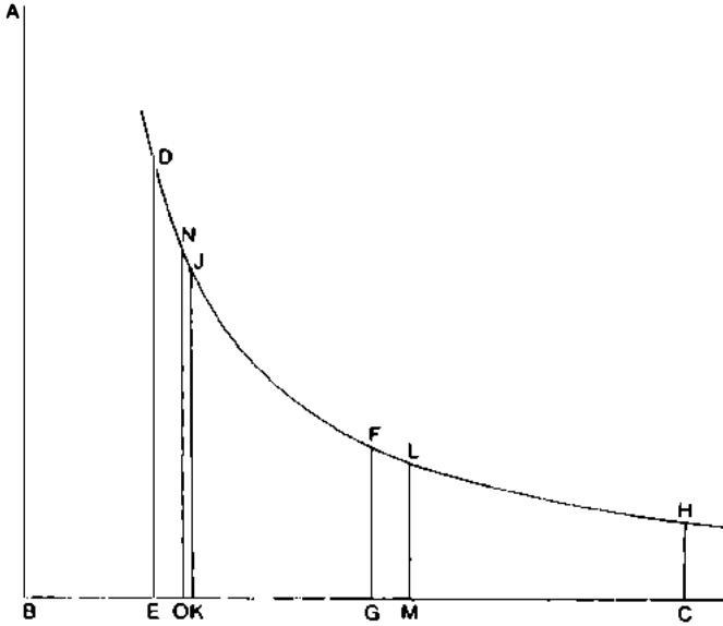
Şekil 1.9. Gregory DEGF ile FGCH alanlarını alanları birbirine eşit sonsuz küçük dilimler aracılığıyla karşılaştırdı.
