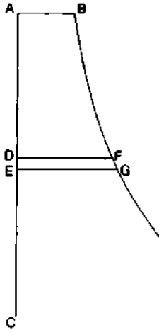
Şekil 10.6. Uzaklığın fonksiyonu olarak değişen bir kuvvetin etkisi altındaki dikey hareketin genel olarak ele alınışı.
