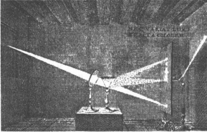
Şekil 15.2. Fransızca ikinci Optique baskısı için Newton tarafından çizilen experimentum crucis . Aşağıdaki resim, baskıda kullanılan halidir. (Oxford, New College yönetiminin izniyle.)
