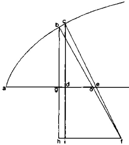
Şekil 4.4. Newton'ın eğrilik merkezi \ell in konumunu saptama yöntemi.
