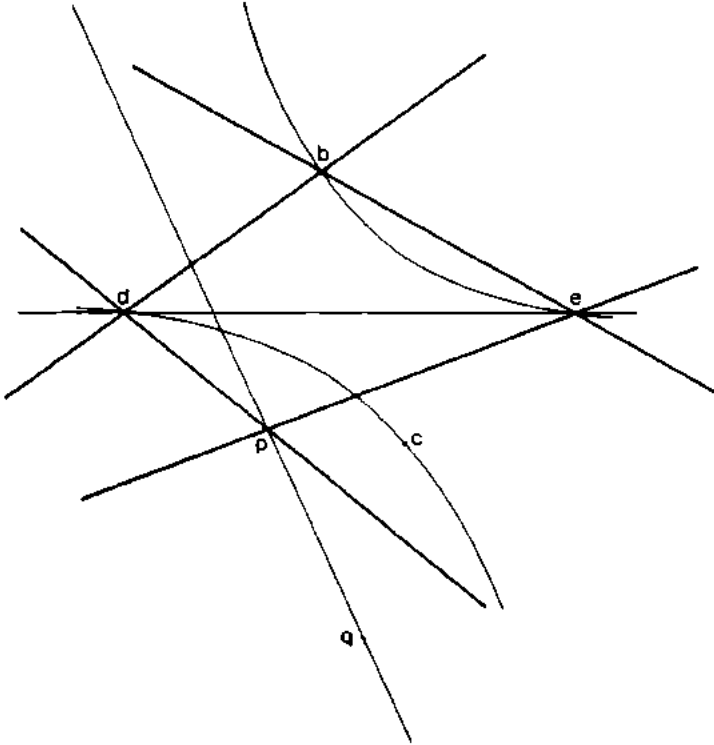
Şekil 6.2. Newton'ın eğrilerin çizilmesine ilişkin sistematik yöntemi. Büyüklükleri sabit bdp ve bep açıları d ve e noktaları etrafında döner. p kesişim noktası pq doğrultmanını çizerken, b kesişim noktası da , be , dc eğrilerini, yani d 'den e 'ye bir konik (bu örnekte bir hiperbol) çizer.
