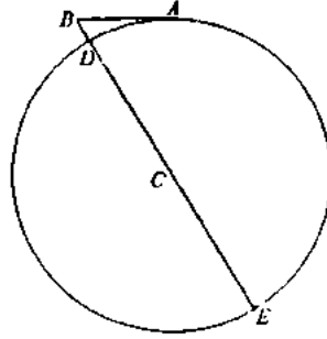
Şekil 5.3. Dairesel hareket yapan bir cismin kuvvetinin teğetten sapmasından yararlanılarak hesaplanması.
