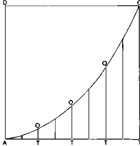
Şekil 1.11. Wallis'in ATOD karesiyle parabolün altında kalan AOT alanı arasındaki orana ilişkin gösterimi.
