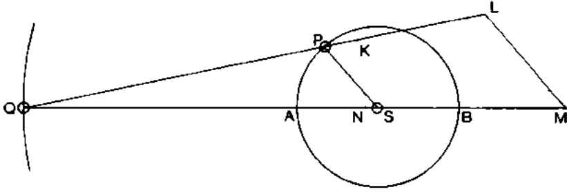
Şekil 10.5. Bunun gibi bir şekil günümüze ulaşmamıştır. Metinden hareketle, LXVI. Önerme-deki şekil örnek alınarak çizilmiştir.
