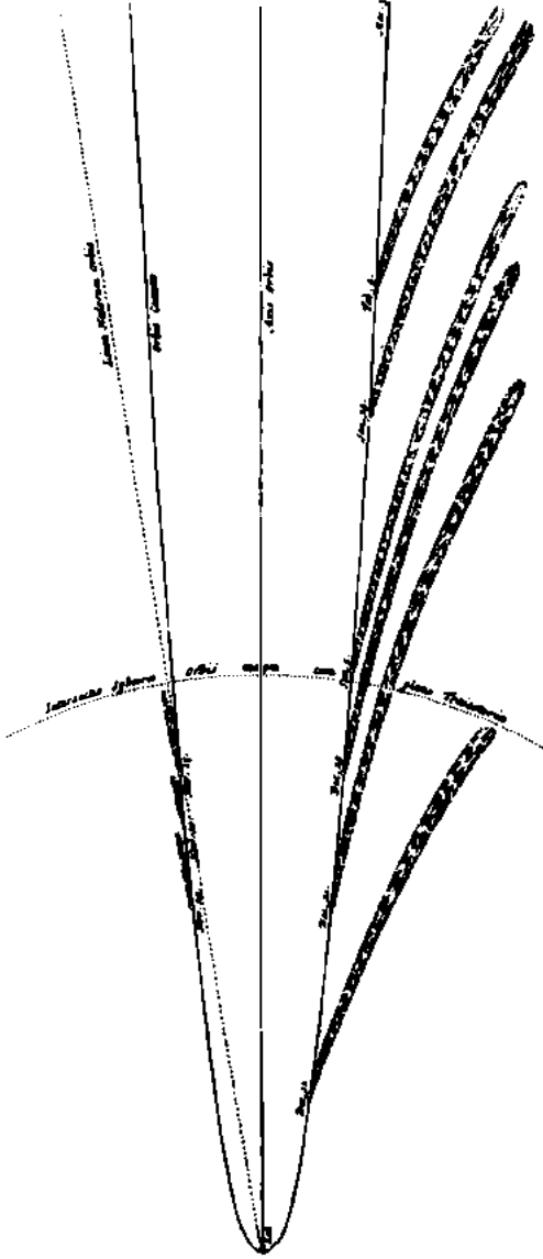
Şekil 10.10 1680-1681'in büyük kuyruklu yıldızının konik yörüngesi. ( Principia 'nın ilk baskısındaki diyagramdan alınma.)
