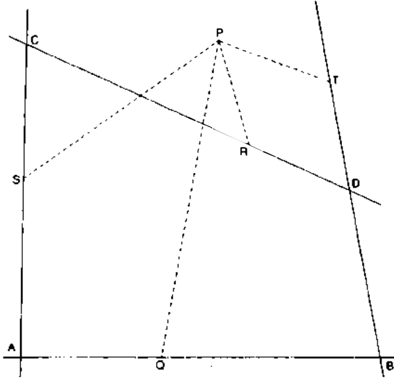
Şekil 1.4. Dört parça problemi. AB , BD , CD ve AC doğru parçaları şekildeki gibi verilmiş olsun. Bu dört doğru parçasına her biri kesiştiği doğru parçasıyla her zaman aynı açıyı yapan PQ , PR , PS ve PT doğru parçalarının çizilebileceği P noktalarının geometrik yerini bulun, öyle ki PQ \cdot PR , PS \cdot PT ile daima belli bir oranda olsun. Geometrik yer, verilen dört doğru parçasının dört kesişim noktasından ( A , B , C , D ) geçen bir koniktir.
