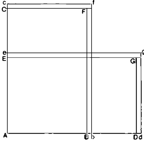
Şekil 6.8. Başlangıç veya oranlar kavramı.
