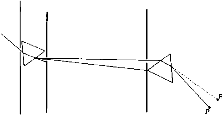
Şekil 6.5. Experimentum crucis .
