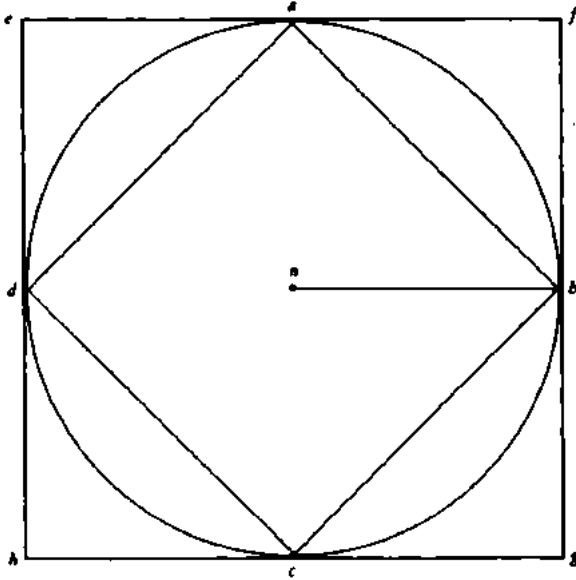
Şekil 5.2. Dairesel bir hareket yapan bir cismin kuvvetinin çarpmadan elde edilmesi.
