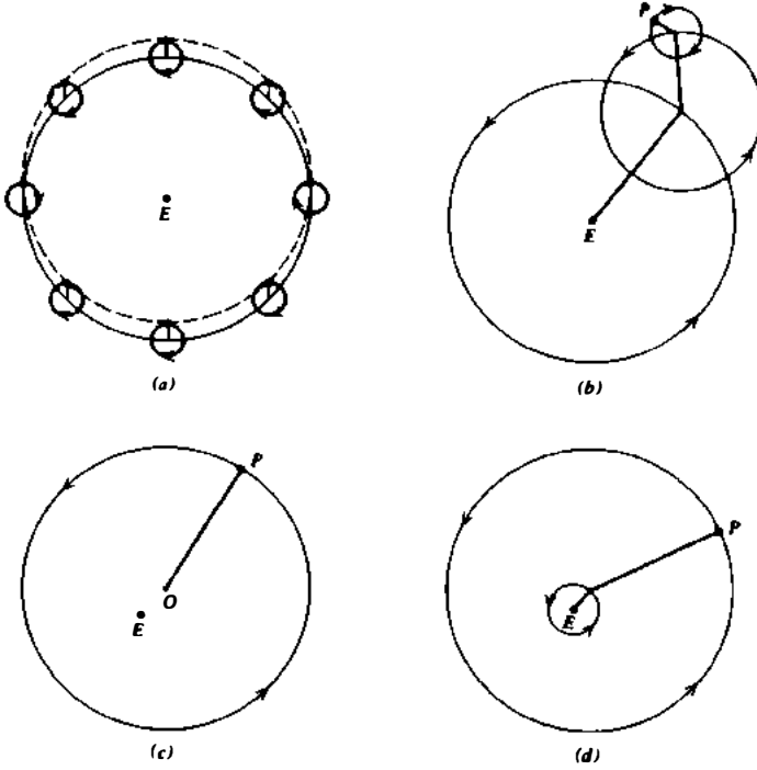
Şekil 1.2. Ptolemaios sistemindeki çeşitli düzenekler. A taşıyıcı çember ile dönüş süresi aynı olan daha küçük bir ilmeğin ortaya çıkardığı sonucu gösteriyor; B, asıl taşıyıcı çemberin üzerindeki bir ilmeği; C, eşmerkezli olmayan çemberleri ve D de bir taşıyıcı çember üzerindeki eşmerkezli olmayan çemberi gösteriyor. Küçük ilmeklerin büyüklükleri ve merkezden kaçıklığın miktarı taşıyıcı çemberin büyüklüğüne göre bir hayli abartılmıştır.
