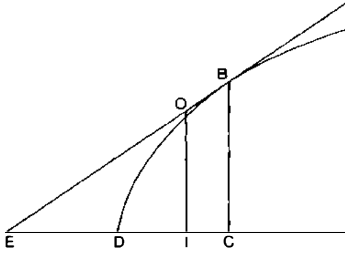
Şekil 1.7. Fermat'ın teğetleri bulma yöntemi.
