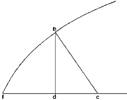
Şekil 4.3. dc normalaltının uzunluğunu saptamak için Newton'ın kullandığı yöntem.
