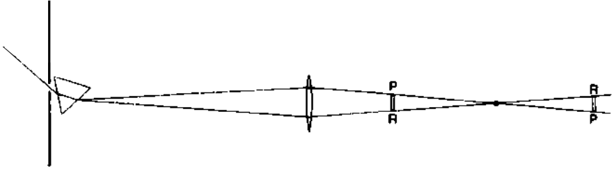
Şekil 6.6. Bir mercek yardımıyla beyaz ışığın yeniden oluşturulması.
