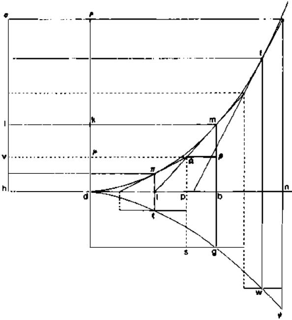
Şekil 4.13 Kalkülüsün temel teoremi.
