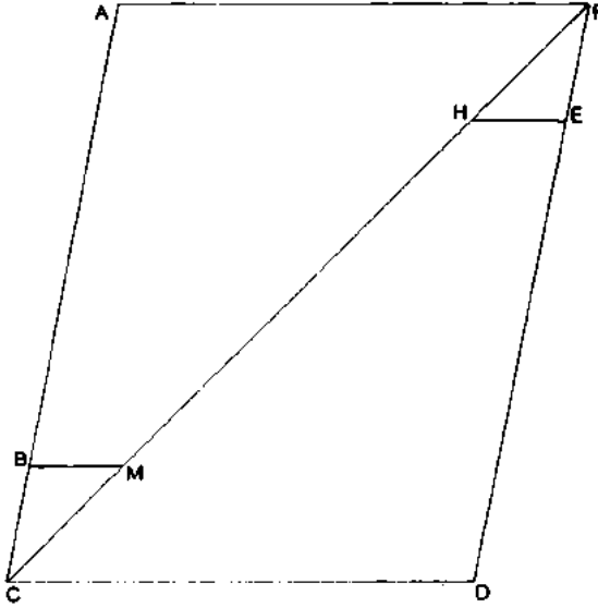
Şekil 1.8. Cavalieri'nin sonsuz küçükler yoluyla bir üçgenin alanını hesaplaması. Şema iki üçgendeki sonsuz sayıda doğru parçası çiftinden yalnızca birini gösteriyor.
