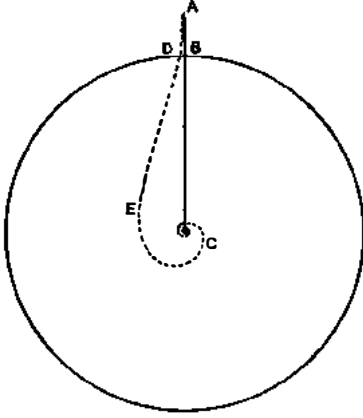
Şekil 9.3. Newton'ın dönen bir yerküre üzerine düşen bir cismin izlediği yola ilişkin çizimi. (Westfall, Force in Newton's Physics 'ten [Newton Fiziğinde Kuvvet]).
