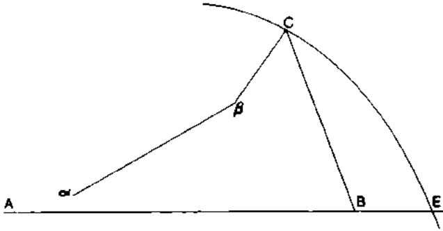
Şekil 6.3. Kübik eğrinin AB , BC koordinatlarının \alpha\beta , \beta C farklı koordinatlarına dönüştürülerek indirgenmesi.
