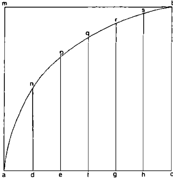
Şekil 4.5. Alanları hesaplamak için sonsuz küçüklerin ve sonsuz serilerin kullanılması.
