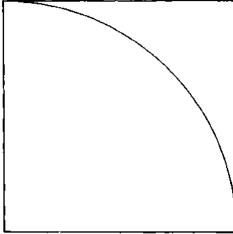
Şekil 1.12. Wallis'in tablosu karenin alanının, p ve n 'in 0'dan 10'a kadar değerleri için y = (1 - x^{1/p})^n eğrisinin altında kalan alana oranını gösteriyordu. Şema; p = 1/2 , n = 1/2 için yarıçapı 1 olan bir dairenin denklemini gösteriyor, Wallis p ve n 'nin integral değerlerini tablosuna yerleştirerek bu denklemden \pi 'nin (daha doğrusu 4/\pi 'nin) değeri için sonsuz bir seri oluşturdu.
