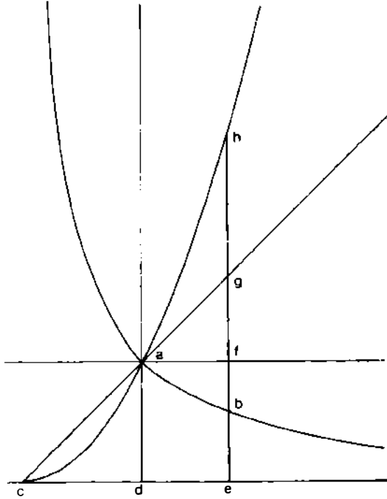
Şekil 4.7. Newton'ın hiperbolü bir dizi benzer eğri kullanarak dış değer bulma (ekstrapolasyon) yöntemiyle karelemesi.
