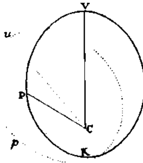
Şekil 10.7: C’den en uzak mesafeye tekrar yükselmesi için 360^{\circ} ’den fazlasına gerek duyan p cismi up yolunda eliptik bir yörünge çiziyor; bu yörünge C odağı etrafında tezdüze dönerken p cismi bu yörünge üzerinde ilerler.
