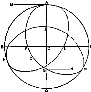
Şekil 9.5. Sabit bir kütleçekim kuvveti altında düşen bir cismin izlediği yol. (Westfall, Force in Newton's Physics 'ten.)
