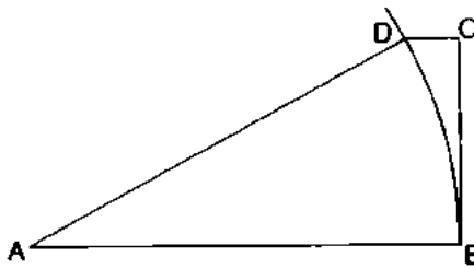
Şekil 10.2. Kesintisiz bir kuvvet tarafından meydana getirilen merkezci ivme.
