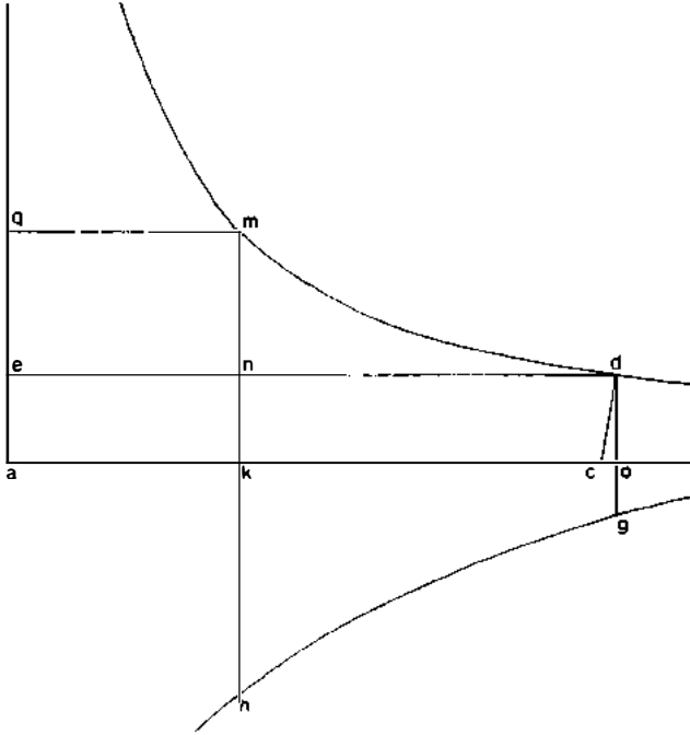
Şekil 4.11. Kalkülüsün temel teoremi.
