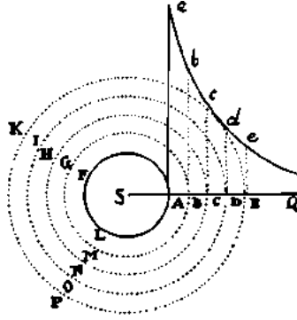
Şekil 10.8 Bir vorteksin dinamiği.
