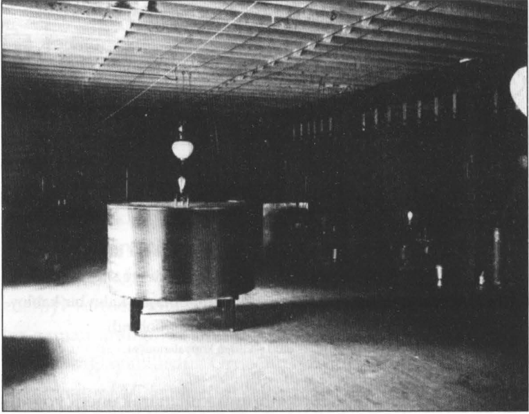
ŞEKİL 10.4. Tesla'nın 1894 civarında Beşinci Cadde'nin güneyindeki laboratuvarında kullandığı rezonans transformatörünün alıcı bobini.
