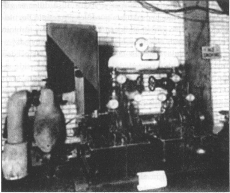
ŞEKİL 16.2. Tesla'nın 1912'de New York'taki Edison Waterside İstasyonu'nda gösterdiği türbin testi teçhizatı. İki motoru bağlayan açık renkli torsiyon yayını görebilirsiniz.
