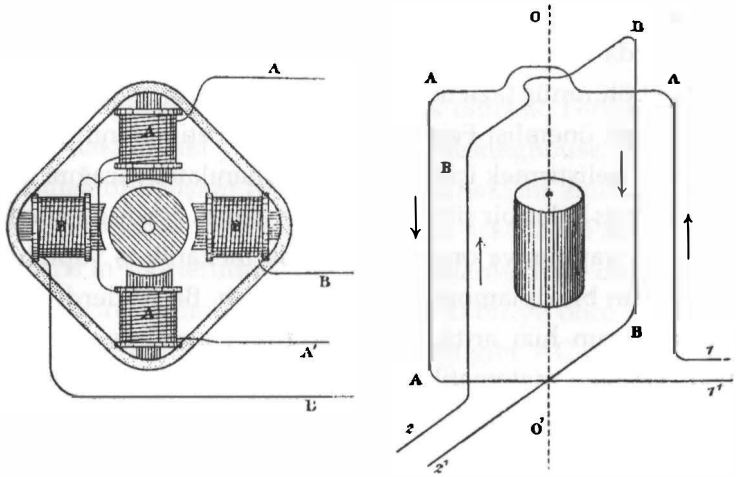
ŞEKİL 5.1. Ferraris'in AC motoru, 1885 civarı.
