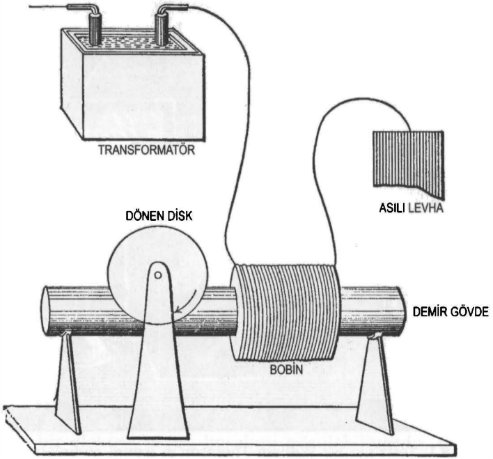
ŞEKİL 8.2. Tesla'nın 1892'de Londra konferansında gösterdiği tek telli motoru.
