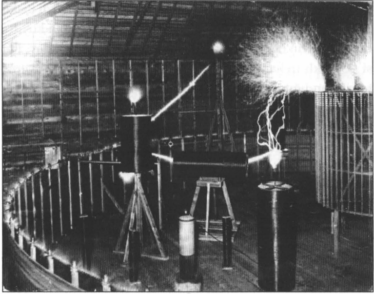
ŞEKİL 13.7. Birkaç ikincil bobiniyle büyütücü verici, dairesel duvardaki birincil bobinlerden enerji alıyor. İki ikincil bobin de farklı sayılarda sarıma sahip olduğundan, toprağa gönderilen ve Tesla'nın alıcısına iletilen iki farklı dalga boyu üretiyordu.
