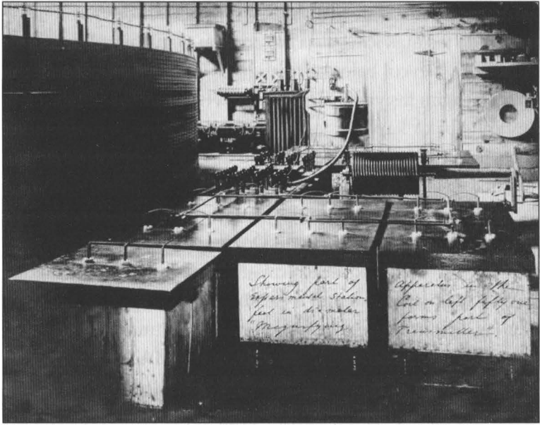
ŞEKİL 13.3. Deney istasyonunun içi. Büyütücü vericinin birincil bobinine elektrik sağlayan bileşenler görülüyor.
