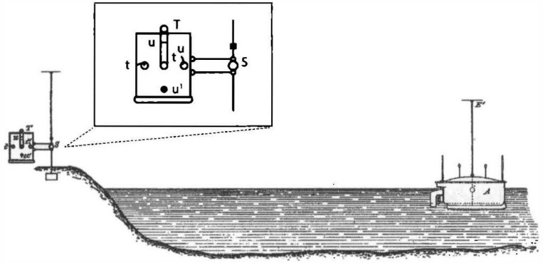
ŞEKİL 12.5. Tesla'nın telsiz kontrollü teknesini ve vericisini gösteren çizim.
