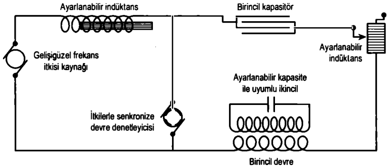
ŞEKİL 10.3. Tesla'nın Beşinci Cadde'nin güneyindeki laboratuvarında lambalarına kablosuz güç iletmek için kullandığı devre, 1894 civarı.
