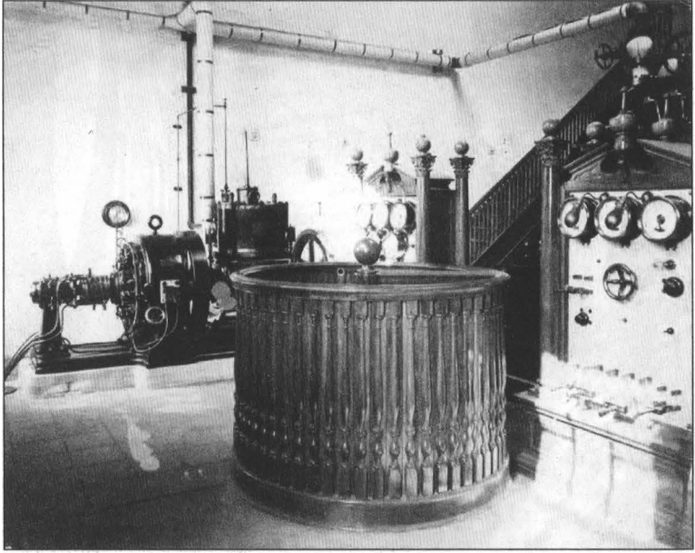
ŞEKİL 14.3. Wardenclyffe’teki makine ve dinamo dairesi, cıvalı şalter ve kontrol panelleri üzerindeki süslü ahşap işçiliğini gösteriyor.
