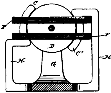
ŞEKİL 3.4. Tesla'nın 1882'de Strasbourg'da yaptığı AC motorunun çizimi.
