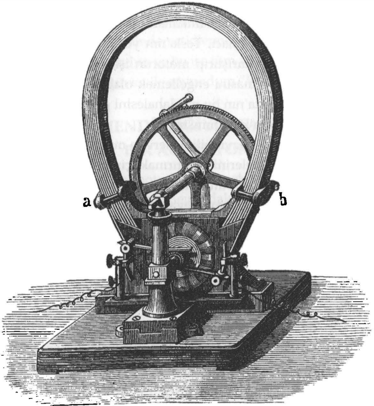
ŞEKİL 2.6. Sınıfta gösterilen Gramme jeneratörü.
