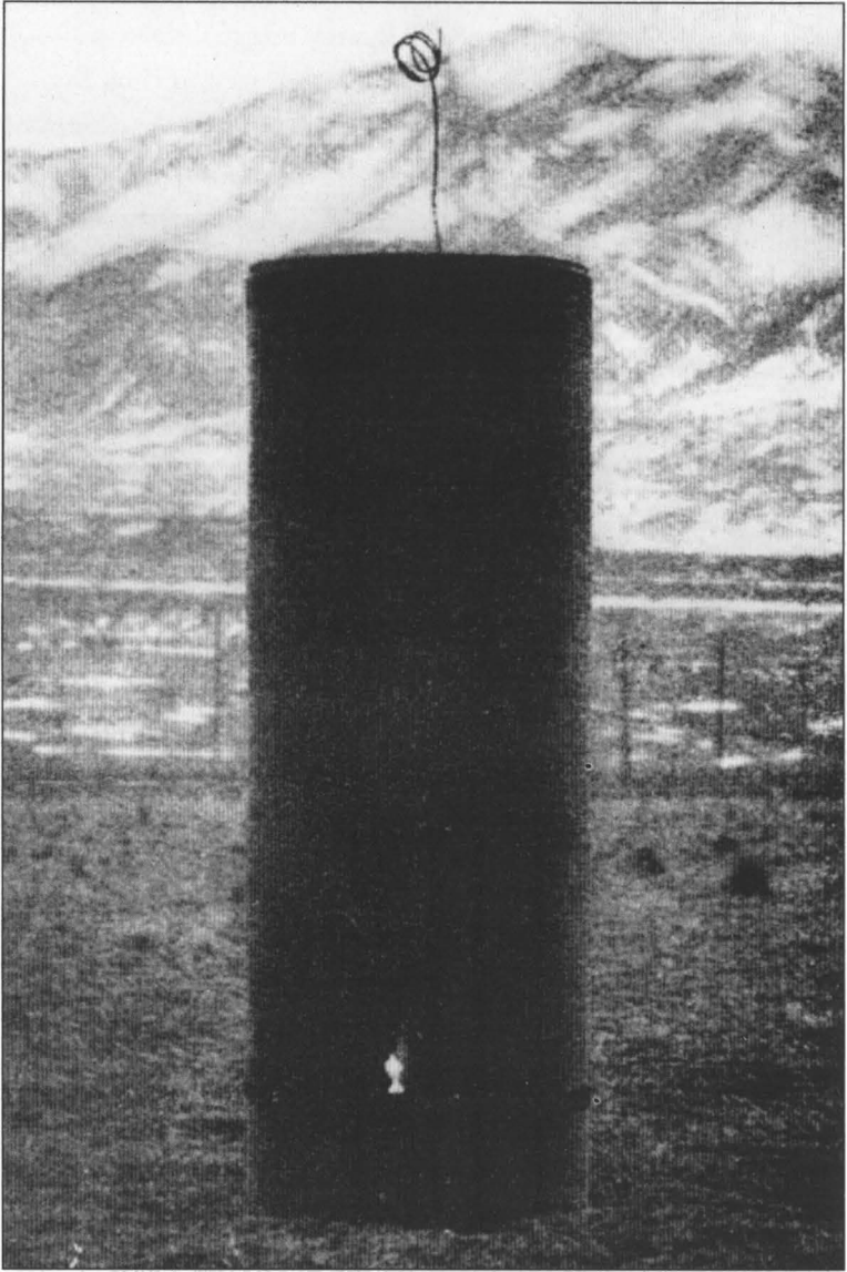
ŞEKİL 13.9. “Elektrik enerjisinin kablosuz iletimini gösteren deney” Burada Tesla alt ucu toprağa bağlı, üst ucu ise serbest olan bir bobini laboratuvarın dışına koyuyordu. Lamba bobinin alt ucunun etrafına sarılmış üç sarım telle yanıyordu. Levha XXVI, CSN, 340. NTM'den.
