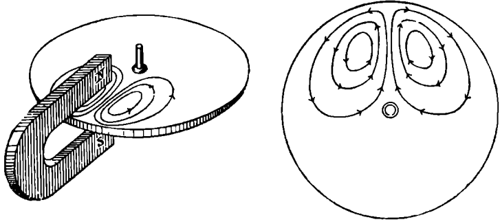
ŞEKİL 2.8. Manyetik alanda dönen bir diskin girdap akımları.
