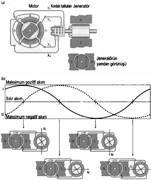
ŞEKİL 4.3. Tesla'nın AC motoru, 1887.
