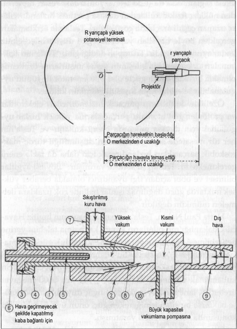
ŞEKİL 16.6. Tesla'nın ışın silahından aşırı yüklü civa parçacıkları fırlatmak için kullanmayı planladığı projektörün çizimleri.
