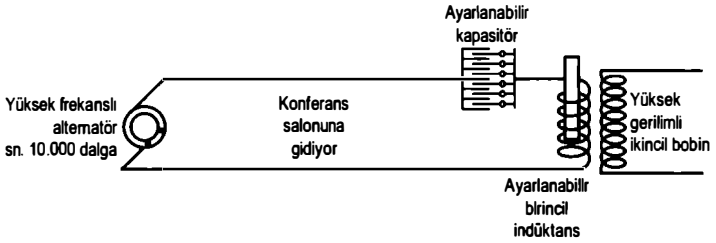
ŞEKİL 7.1. Tesla'nın 1891'de Columbia Üniversitesi'ndeki konferansında kullandığı devre. Osilasyon transformatörü veya Tesla bobini sağ taraftaki kapasitör, indüktans ve transformatörden oluşuyordu.
