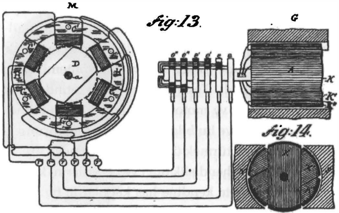
ŞEKİL 3.3. Tesla'nın patentindeki çizimde, sistemdeki jeneratörün üç ayrı alternatif akım ürettiği, bunların motora altı ayrı telle iletildiği görülüyor.
