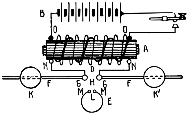
ŞEKİL 6.1. Hertz'in elektromanyetik dalgaları incelemek için kullandığı teçhizatın çizimi.
