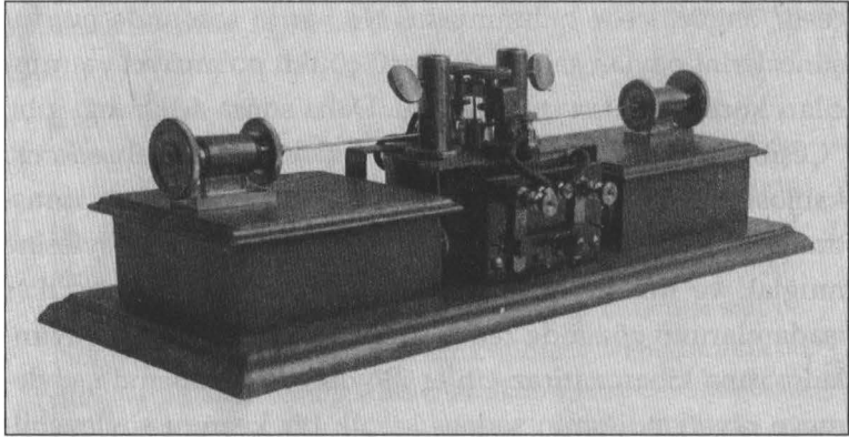
ŞEKİL 10.1. Tesla'nın 1890'ların ortalarında elektromanyetik dalgaları tespit etmekte kullandığı alıcı.
