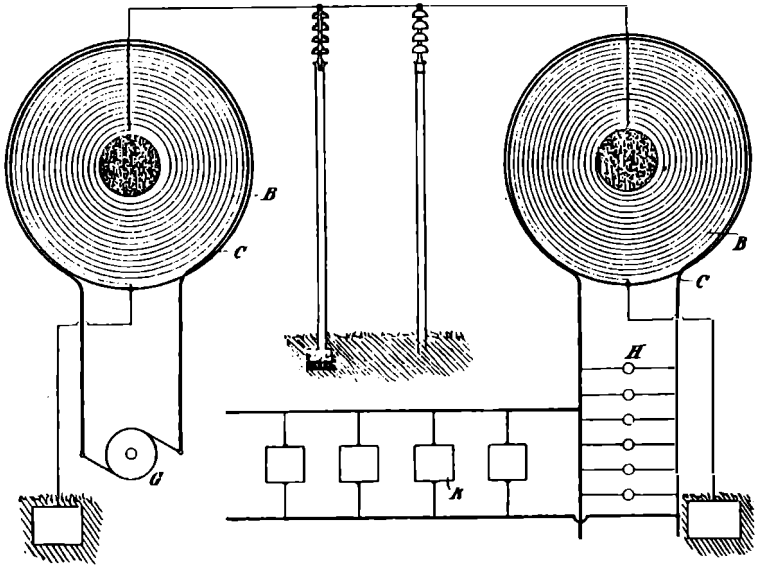
ŞEKİL 12.9. NT, "Electrical Transformer," US Patent 593,138 (başvuru: 20 Mart 1897, onay: 2 Kasım 1897).
