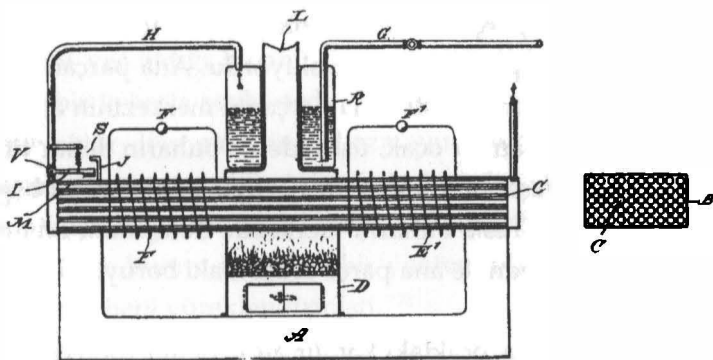
ŞEKİL 4.2. Tesla'nın piromanyetik jeneratörü, 1886-1887.
