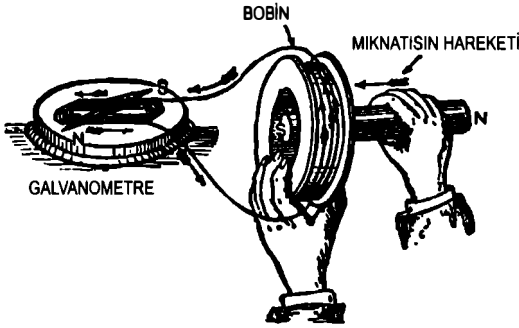
ŞEKİL 2.1. Faraday'ın elektromanyetik indüksiyon kanunu.
