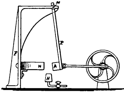
ŞEKİL 4.1. Tesla'nın 1886'daki termoelektrik motoru.
