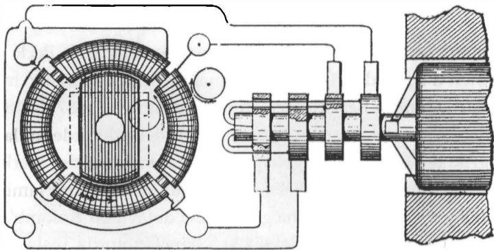
ŞEKİL 4.5. Tesla'nın 1887 sonbaharında AC motor deneyleri için kullandığı temel deney düzeneği.
