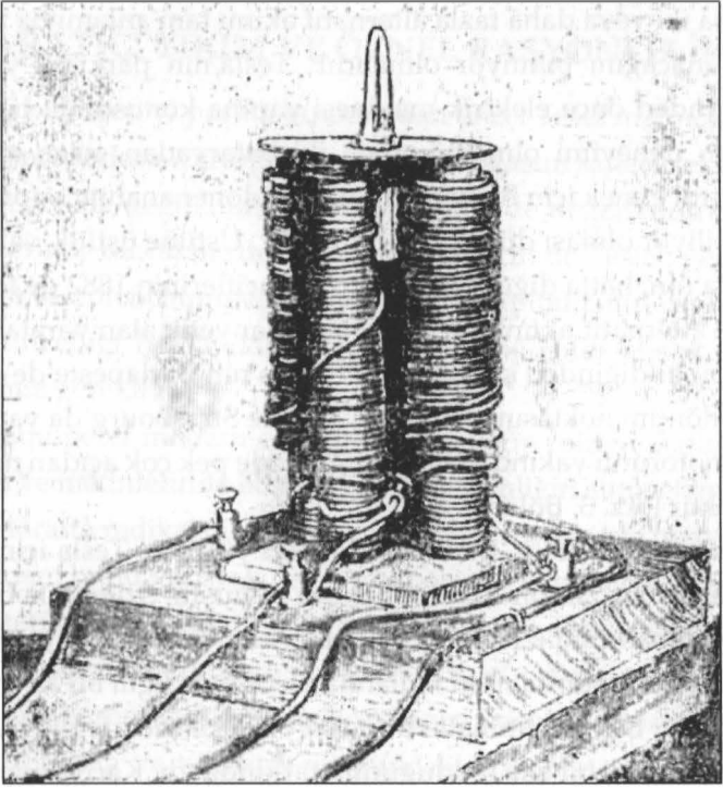
ŞEKİL 2.9. Baily'nin elektrik motoru, 1879.
