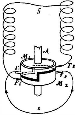
ŞEKİL 2.3. Hippolyte Pixii'nin 1832 yılına ait ilk komütatörü ile manyetosu.
