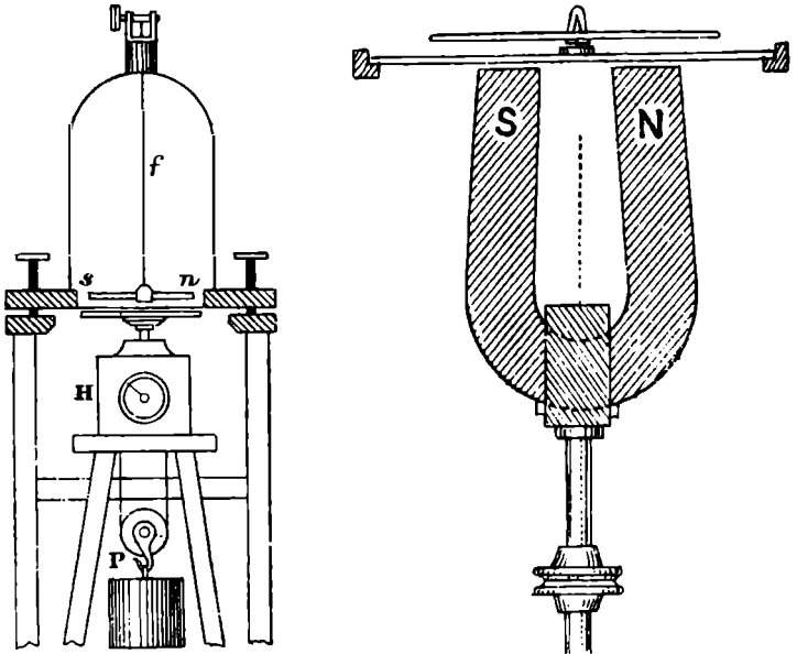
ŞEKİL 2.7. Arago'nun dönen diski (solda) ile Babbage ve Herschel'in yaptığı değişik versiyon (sağda).
