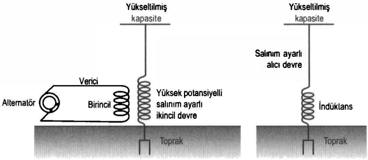
ŞEKİL 7.3. Tesla'nın verici ile alıcısını nasıl toprakladığını gösteren şekil. 1916'da yaptığı açıklamada Tesla 1891'den beri böyle düzenekler kullandığını belirtmiştir. Vericinin kapasitesini yükseltmek için büyük bir teneke kutu kullanmıştır.
