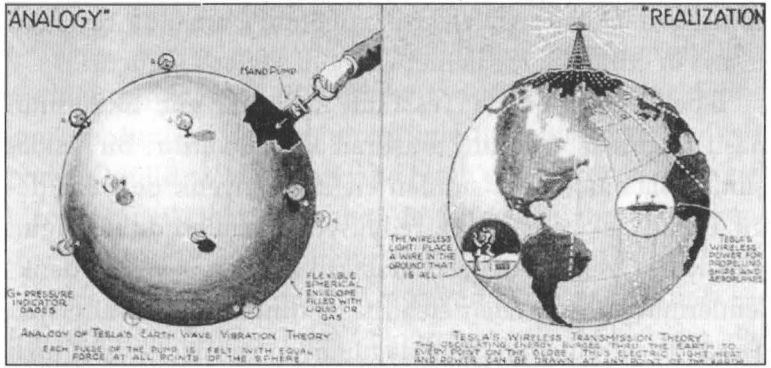
ŞEKİL 15.5. Tesla'nın Dünya'nın sıkışmaz akışkanla dolu olduğuna yönelik vizyonu.
