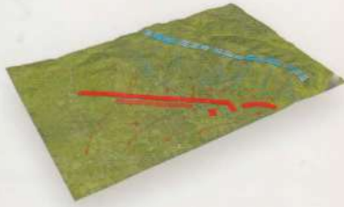
3 boyutlu harekât haritaları
