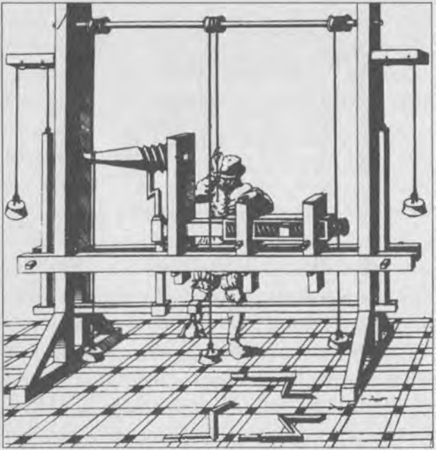
Jacques Besson'un vida kesici makinesi, 1579.
