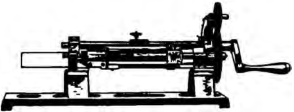
Jesse Ramsden'in duyarlı vida kesici tornası, 1777.
