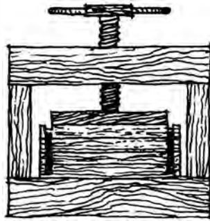
Heron'un doğrudan vidalı presi.
