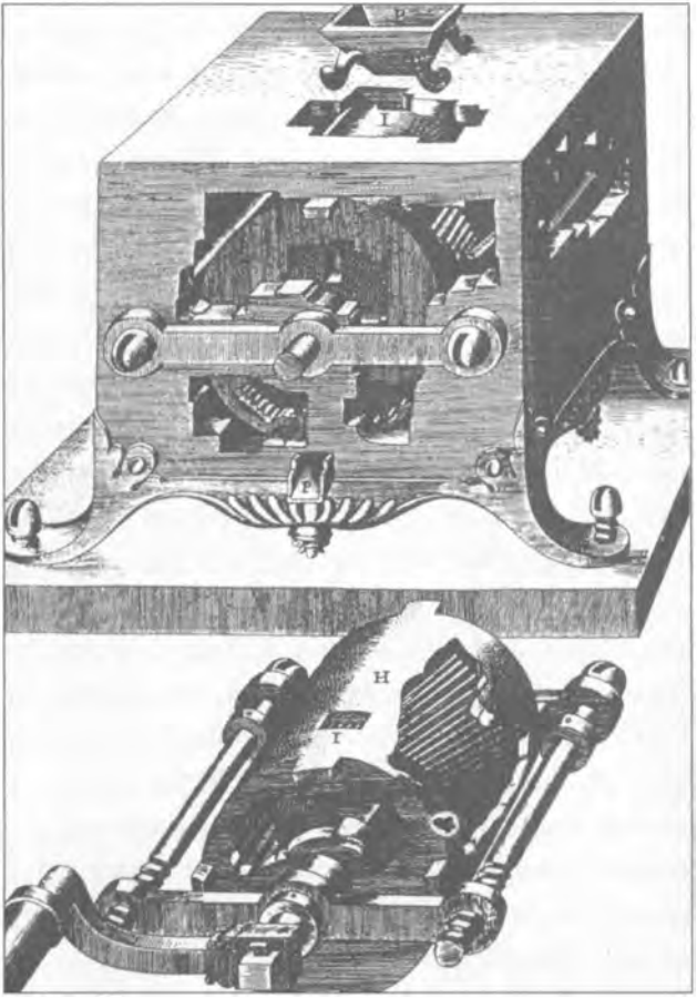
Agostino Ramelli'nin Le diverse et artificiose machine yapıtından, taşınabilir un öğütücüsü, 1588.
