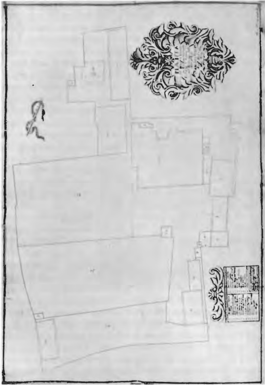
Resim 138. Venedik Sarayı ve müştemilâtının 1746 senesine ait planı (Venier'in 15 Eylül 1746 tarihli dispaccio'suna ekli: 40. 47. F 200)
