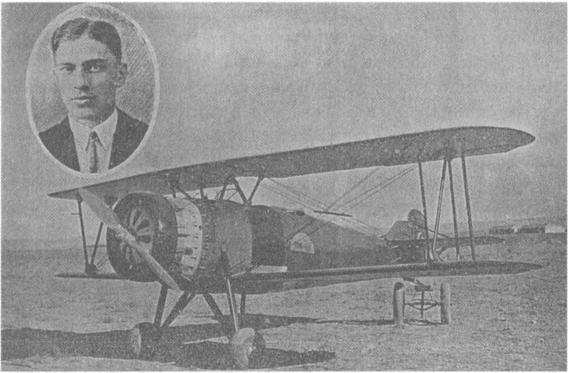
M.M.V.1 tip Selahaddin keşif tayyaresi ve konstrüktörü Müh. Selahaddin Reşit.
