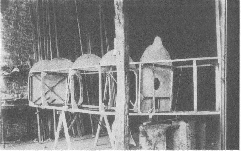
Gövde bölmeleri hazırlıkları...
