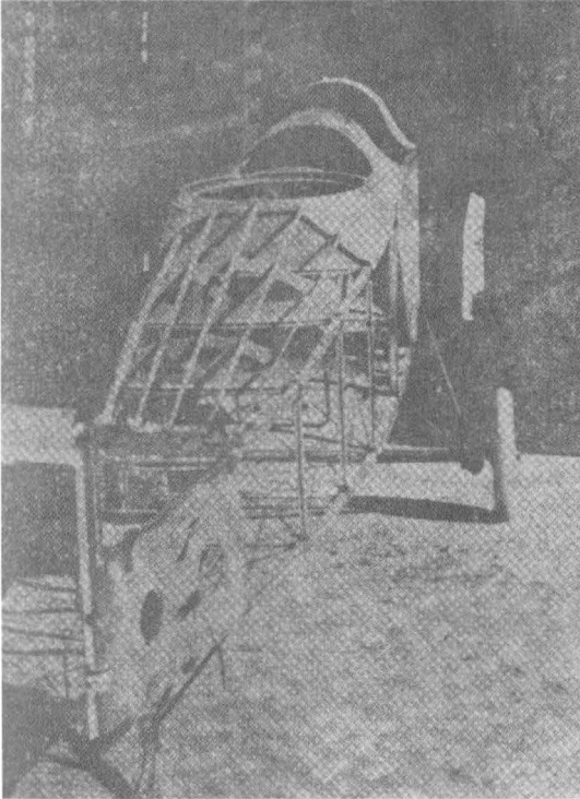
Vecihi K VI tip tayyarenin bezlenmemiş halindeki inşasının ikmali
