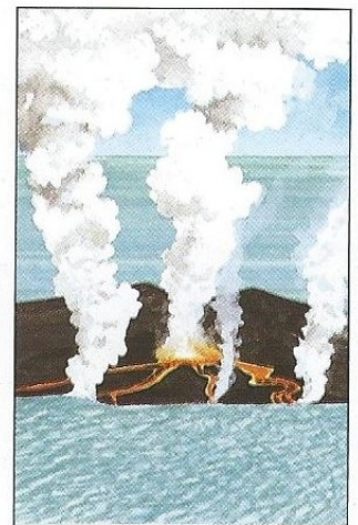
Yanardağ yeterince yükseldikten ve ağzı deniz yüzeyinin üstünde kaldıktan sonra, lav püskürmeleri ve akıntıları birkaç ay daha sürdü ve sonunda ada bugünkü büyüklüğüne erişti.
