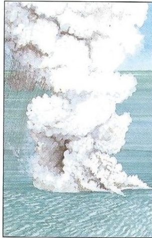
Yanardağ, birkaç hafta boyunca, deniz tabanından yüzeye doğru yükselmesini sürdürmüştü. Deniz yüzeyinden dumanlar yükselince, balıkçılar tarafından fark edildi.
