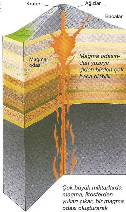
Bir yanardağ kesiti
