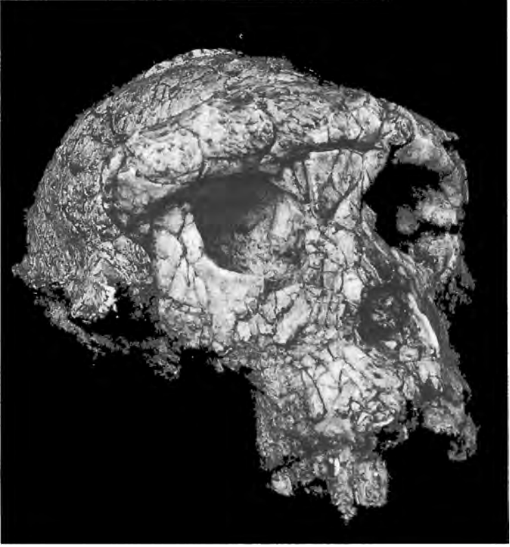
Preparasyon sonrası Sahelanthropus tchadensis kafatası.
