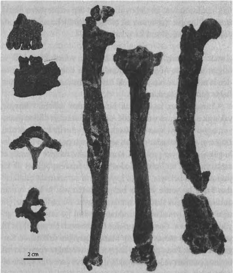
"Udo" Danuvius guggenmosi 'nin önemli kemikleri: Üstçene, altçene, omur, dirsek kemiği, kaval kemiği, uyluk kemiği.
