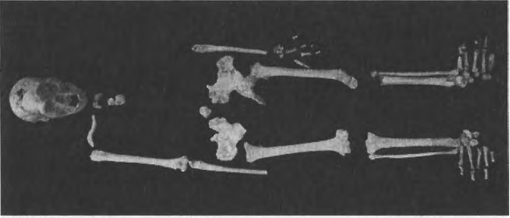
"Hobbit" adıyla bilinen Homo floresiensis 'in LB 1 iskeleti.
