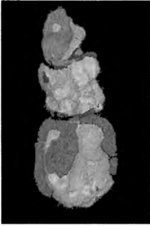
"El Graeco"nın aşınmış dişleri. Diş arayüzleri kayıp, ayrıca dişler iç içe geçmiş.
