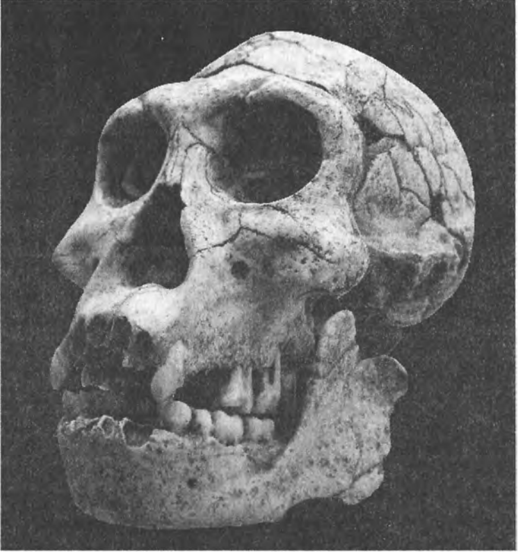
Gürcistan Dmanisi'de keşfedilen tarih öncesi insan Homo georgicus 'un kafatası.
