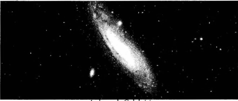
Andromeda Galaksisi
