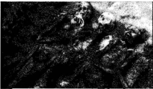
İkinci Dünya Savaşı'ndan kalma bir toplu mezar
