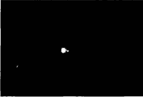
Dünya ve ayın 183 milyon kilometre uzaklıktan görünümü (Messenger uzay aracı tarafından çekilmiştir.)
