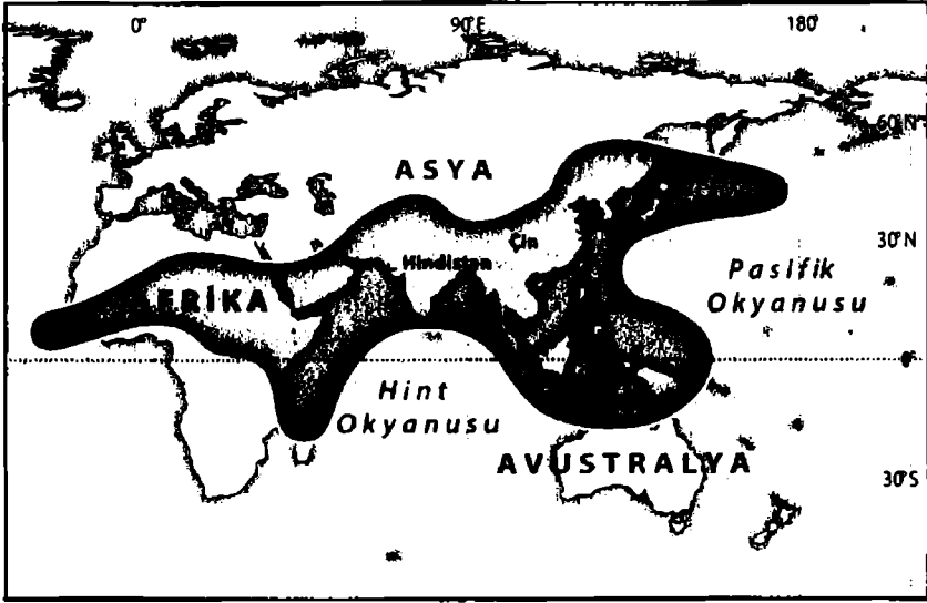
Şekil 7.2 Doğu Yarımküre’de Muson İklim Kuşağı
