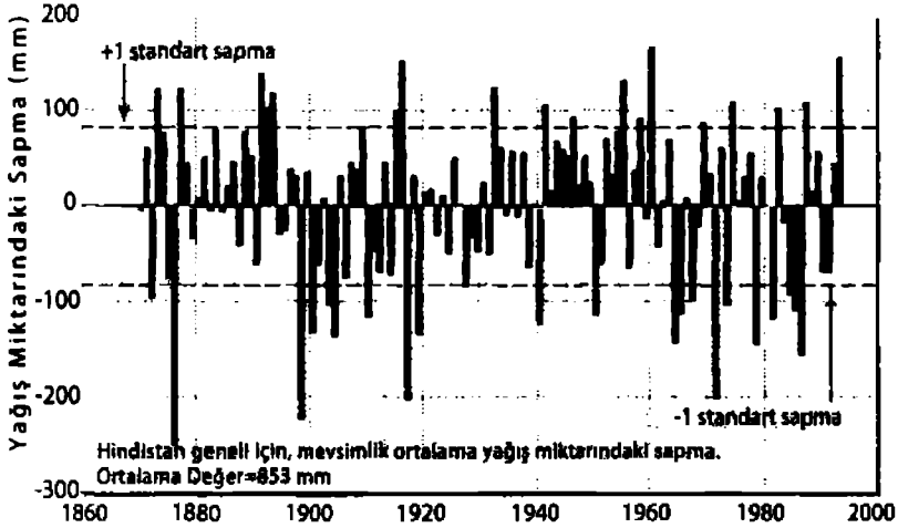
Şekil 8.3 ENSO ve Hindistan Geneli Yağış Miktarındaki Sapmalar
