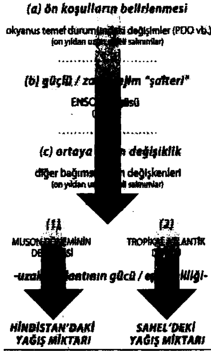
Şekil 8.2 ENSO / Uzak Bağlantı Düzeninin İki Hali
