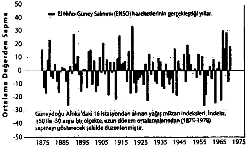
Şekil 8.4 ENSO ve Güneydoğu Afrika'da Yağış Miktarı
