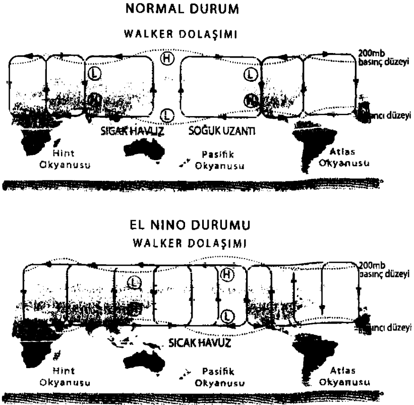
Şekil 7.1 Sıcak Havuz'un Doğuya Kaymasına Bağlı El Niño Hareketi
