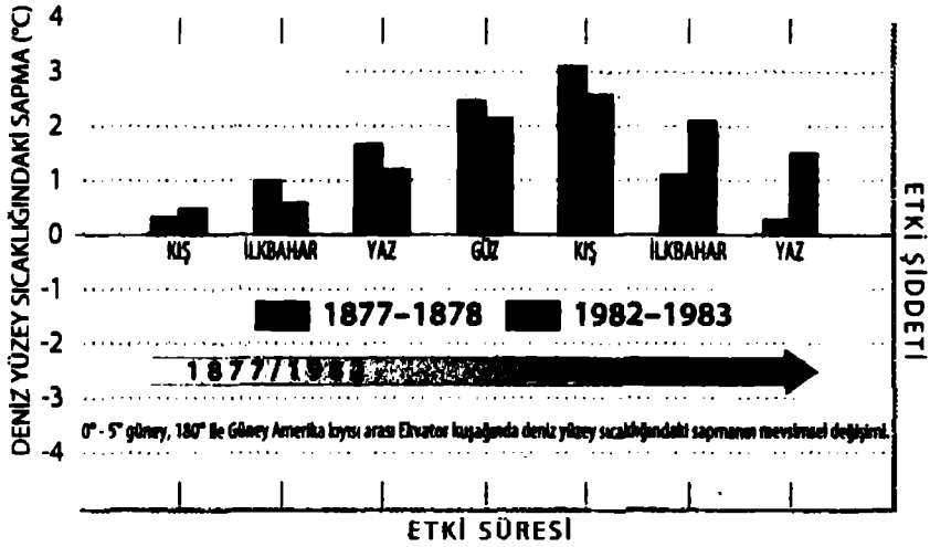
Şekil P2: 1877-78 ve 1982-83 El Niño Hareketleri Arasındaki Karşılaştırma
