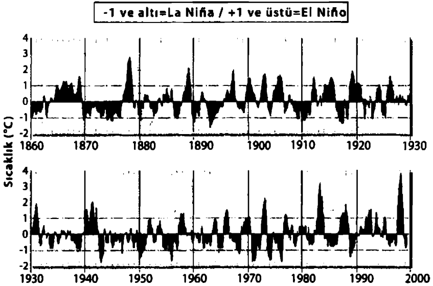
Şekil 7.5 ENSO'nun Salınım Genliğindeki Değişim
