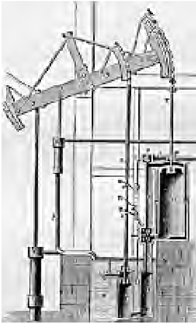
James Watt’ın Buhar Makinası Resim 1-a
