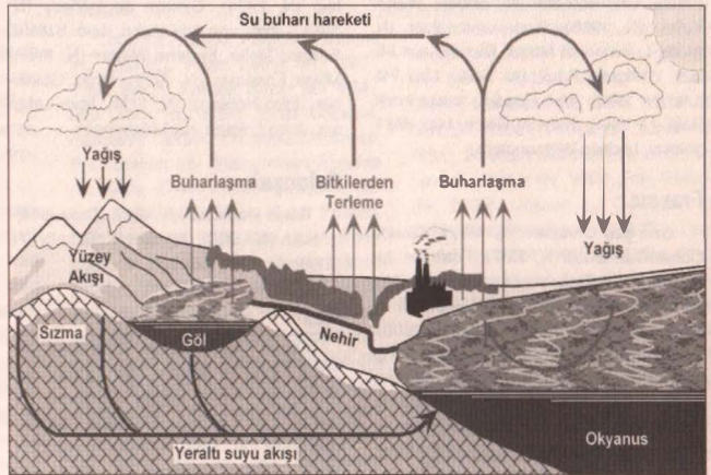
Şekil 1. Dünyadaki su döngüsünün şematik gösterimi.
