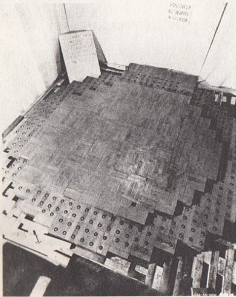
Chicago Pile 1 reaktörünün yapısı. (ABD Enerji Bakanlığı arşivi)
