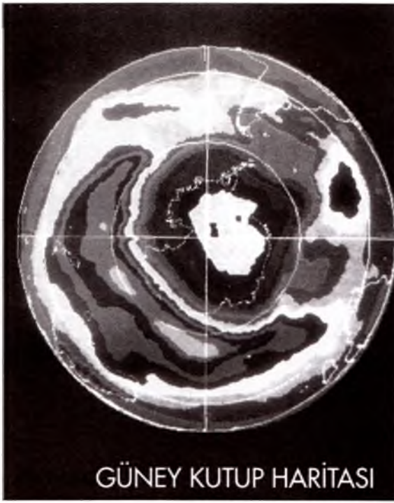
Şek.3-4. Güney kutbunun üzerindeki ozon deliği.
