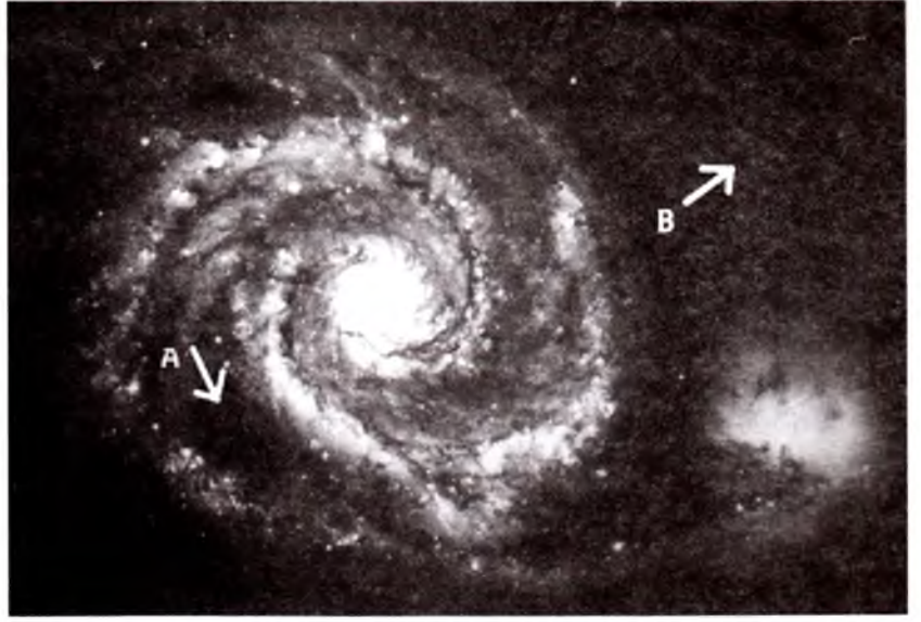
Şek.2-35. Spiral galaksi.
