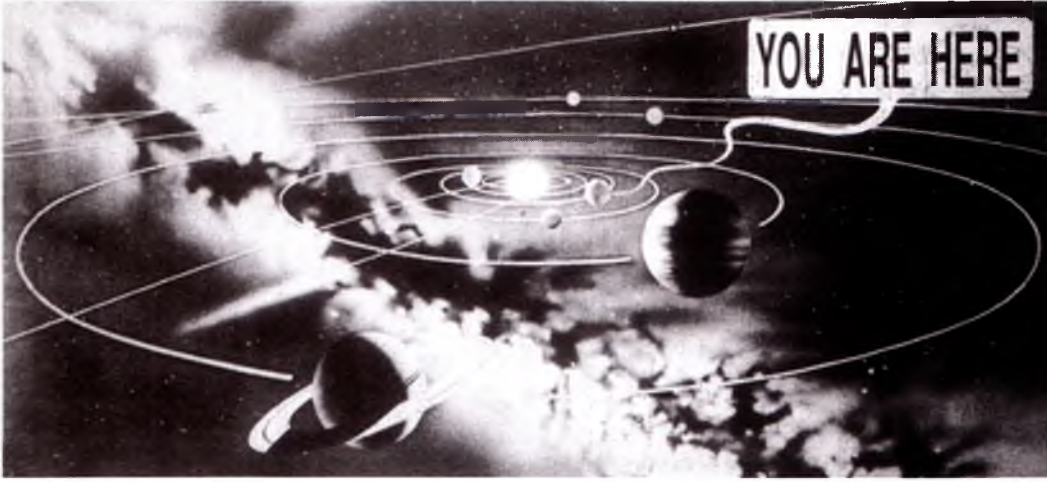
Şek.2-33. Güneş sisteminde Dünyanın yeri.
