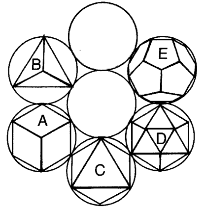
Şek.6-15. Plato'nun beş Cismi.
