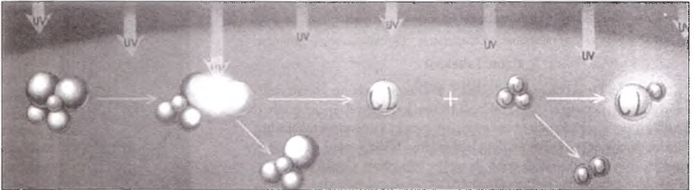
Şek.3-5. Moleküllerde ozon reaksiyonu.
