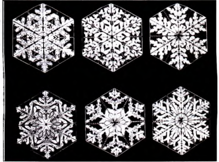
Şek.6-46 Buz kristalleri, veya kar taneleri.
