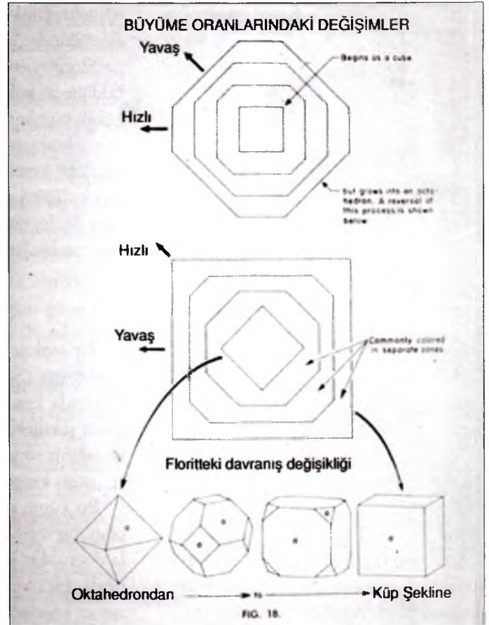
Şek.6-36. Bir florit kristali.
