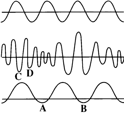
Şek.2-29. Sinüs dalga örnekleri.
