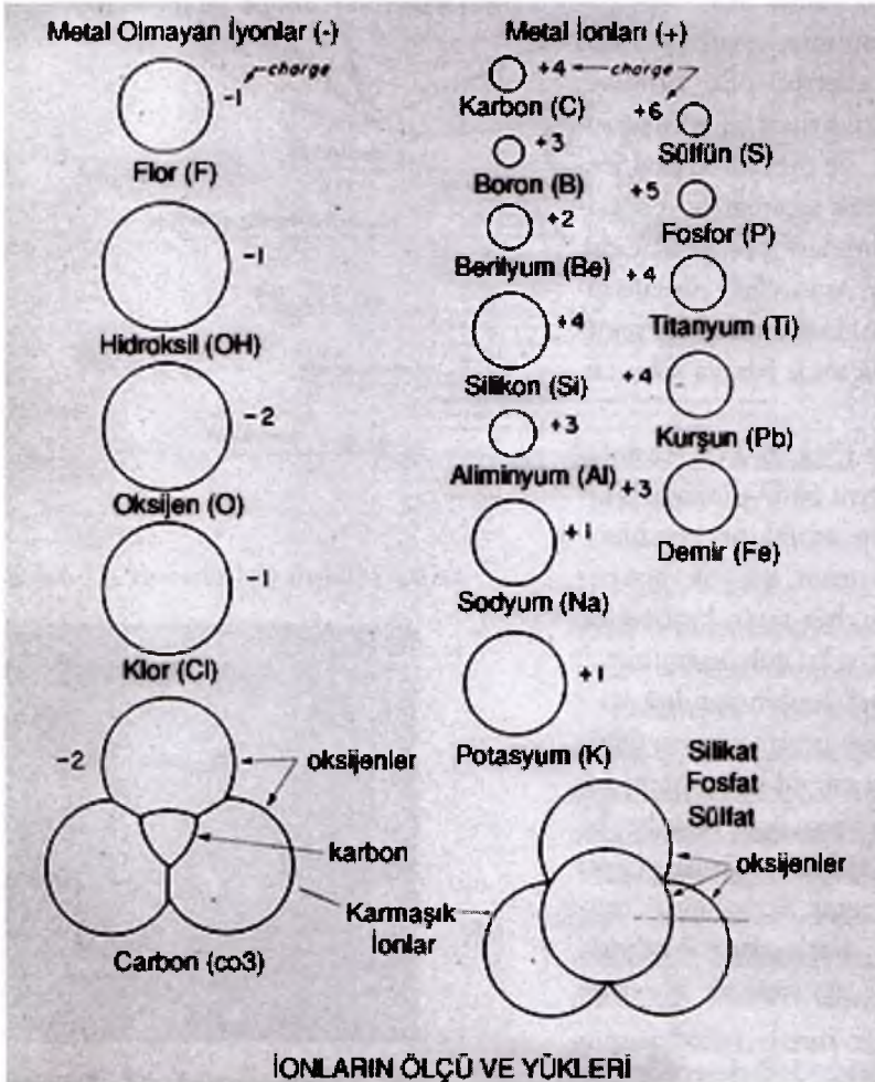
Şek.6-30. İyonların ölçü ve yükleri.
