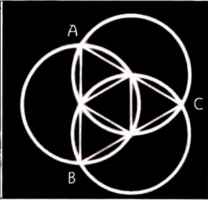
Şek.5-37 Üç kürenin içindeki küçük ve büyük tetrahedronlar.
