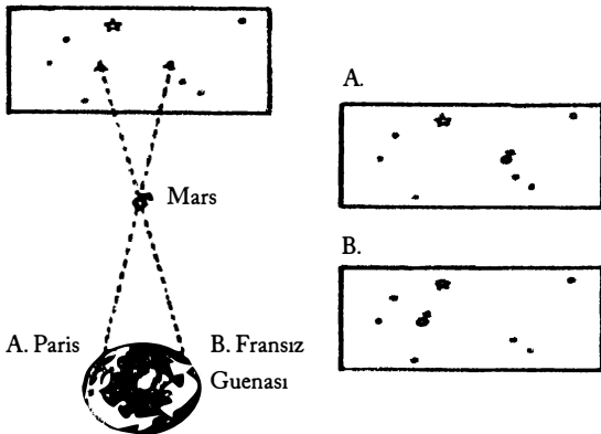
Şekil 2a. Paralaks (Mars'ın)
