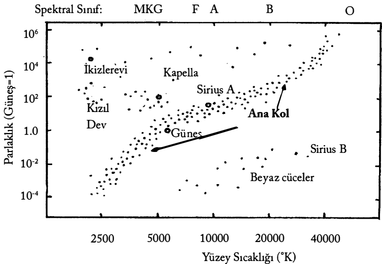
Şekil 7 H-R Diyagramı
