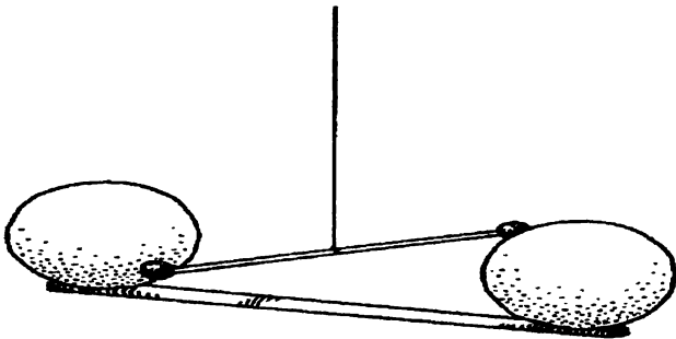
Cavendish Deneyi
