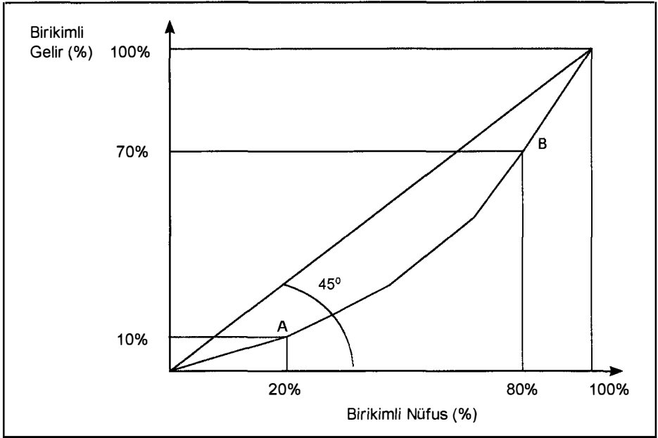
Şekil-2.2: Bir Gelir Dağılımına Ait Lorenz Eğrisi
