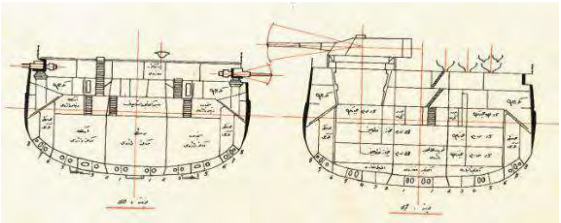
Yavuz'a ait çeşitli teknik resimler (Baş, 2008, s.285)
