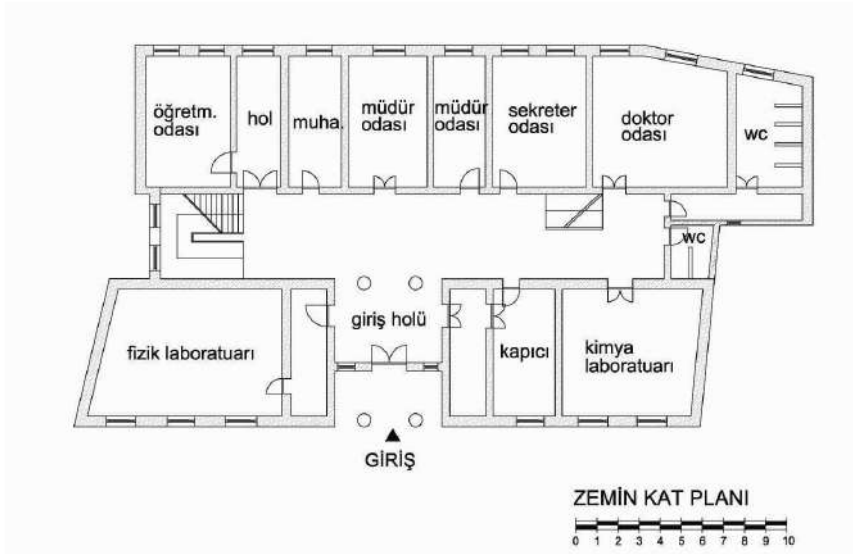
Resim 25. Zoğrafyon Rum Erkek Lisesi'nin zemin kat planı (Karlı, 2006, 41)
