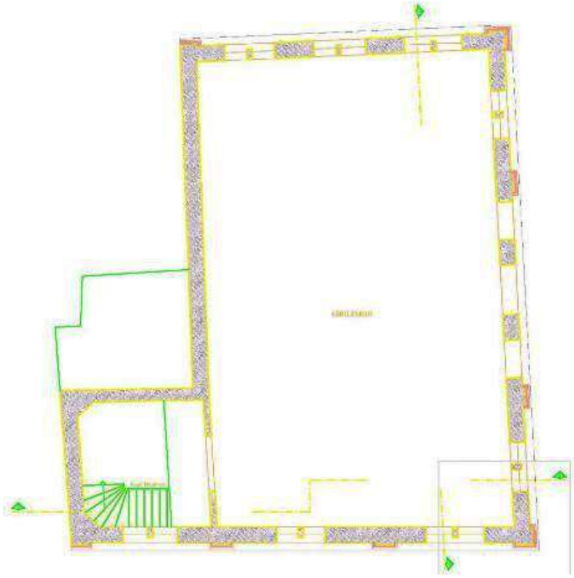
Resim 19. İkinci normal kat planı (MİMSA Mimarlık, 2012)
