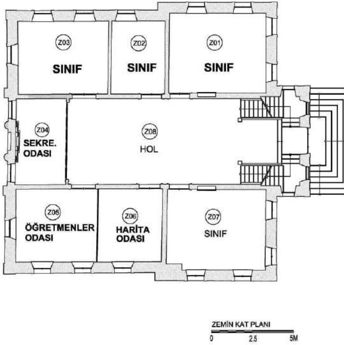
Resim 21. Ioakimion Rum Kız Lisesi'nin zemin kat planı (Karşlı, 2006, 69)
