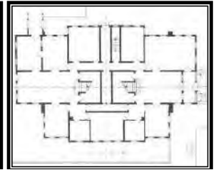
Resim. 6. Hatice Sultan Yalısı 20. yüzyılbaşı ve rölöve planları (Eldem, 1993)
