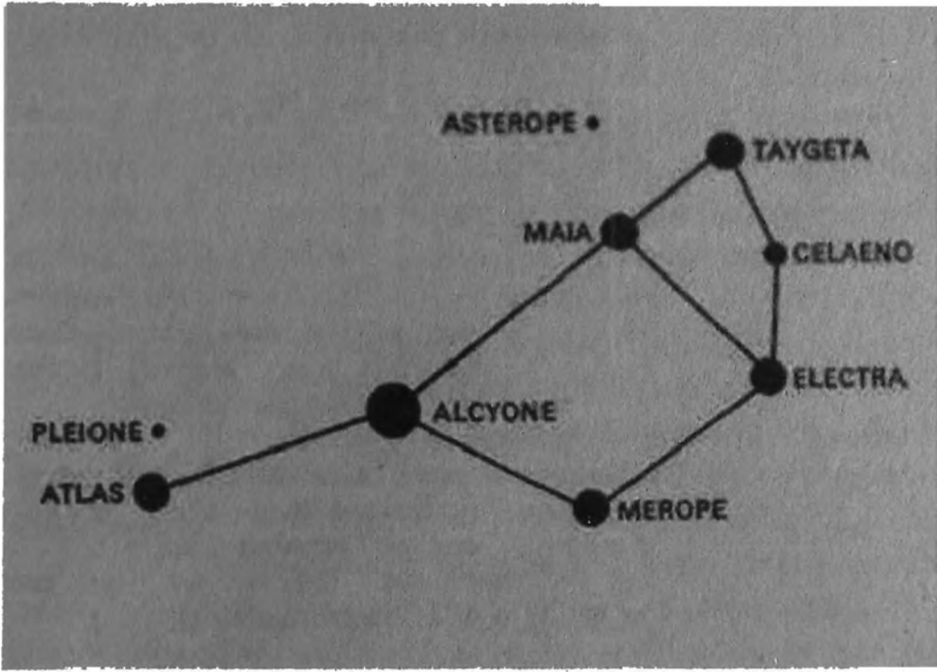
Resim99: Ülker Takımyıldızı
