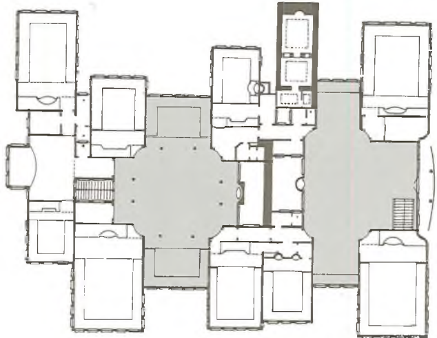
54 İstanbul Bebek - Köçeoğlu Yalısı- Birinci kat planı, (Eldem'den)
