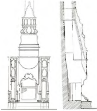
81 Ocak - Topkapı Sarayı - (Zeren'den)
