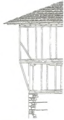
108 Safranbolu - taşırtma
