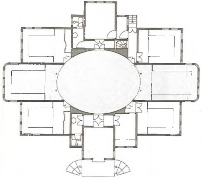
47 İstanbul - Nispetiye Köşkü - 19. Yüzyıl - Plan (Eldem'den)
