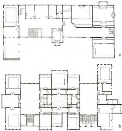
92 Harem ve Selamlık
