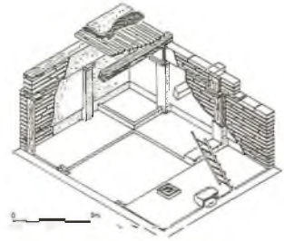
2 Çatalhöyük -Yapı tekniği- Rökonstrüksiyon - M.Ö. 7. Bin (Mellaart'dan)
