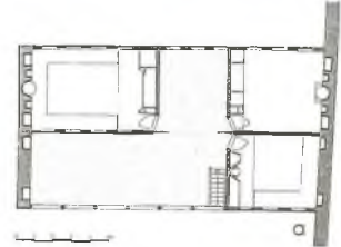
30 İstanbul - Fatih Köşkü - Topkapı Sarayı, 15. Yüzyıl - Plan
