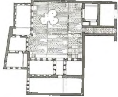
103 Diyarbakır - Hacı Hidir Mahallesinde ev - Harem planı - (Erginbaş'tan)
