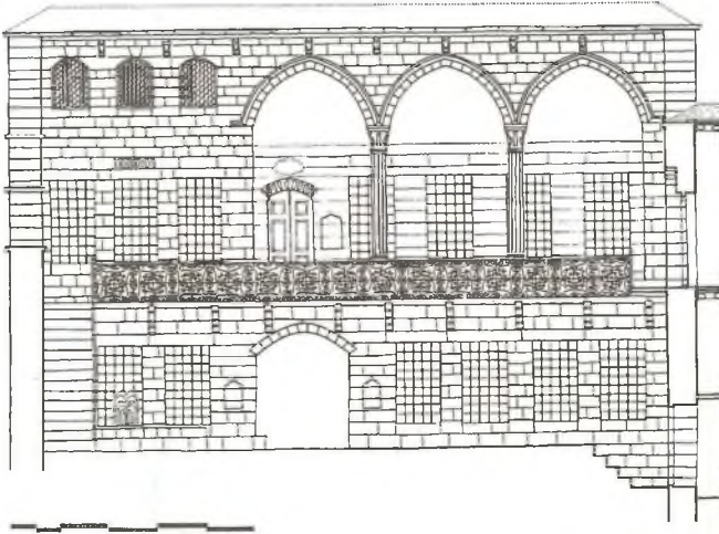
102 Diyarbakır - Hacı Hidir Mahallesinde Ev - Avlunun güney cephesi - (Erginbaş'tan)
