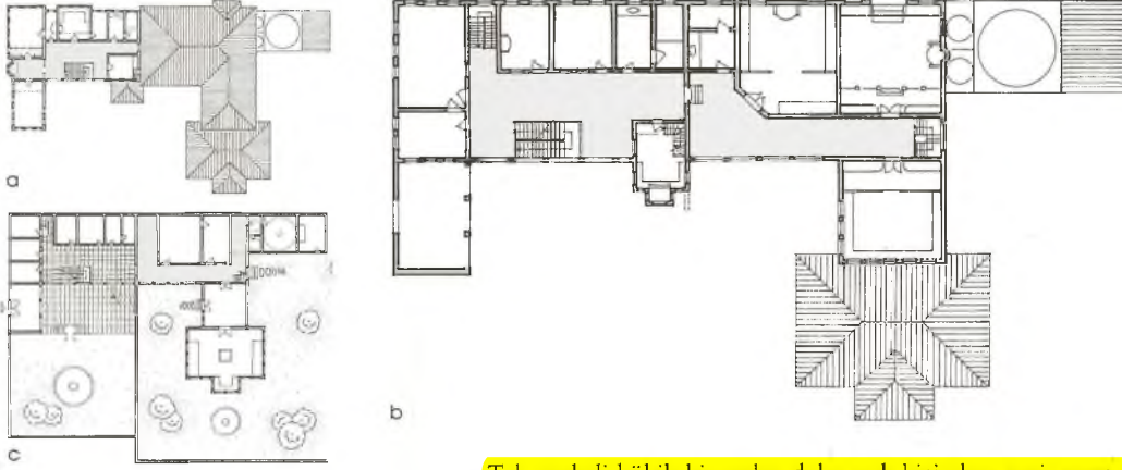
26 Vezir Köprü - Ev - 18. Yüzyıl - Planlar (Şahabeddin'den)
