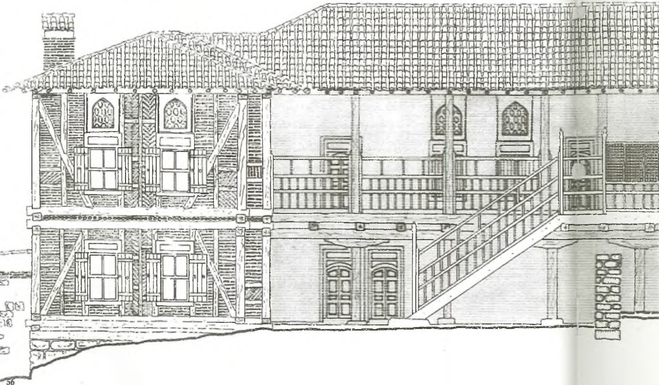
27 Vezir Köprü - Ev - 18. Yüzyıl - Hayat Cephesi (Şahabeddin'in etüdünden yararlanılarak Şirin Akıncı tarafından çizilmiştir)
