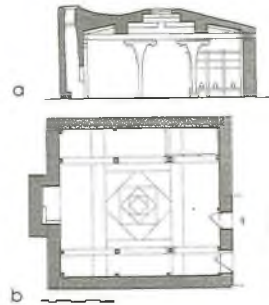
73 Şarkışla - Cem Evi - (G.Akın'dan)
