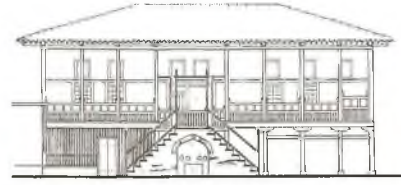
100 Bursa - Halıcı İzzet Evi - Hayat cephesi
