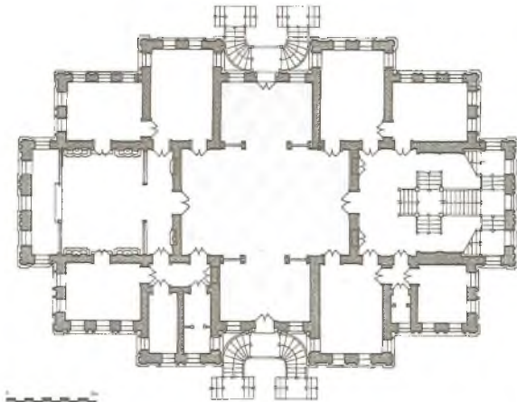
55 İstanbul - Yıldız Sarayı Mabeyn Köşkü - Giriş katı - 1865
