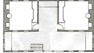
22 Mudanya - Halilağa Evi - 1640 - Plan (Eldem'den)
