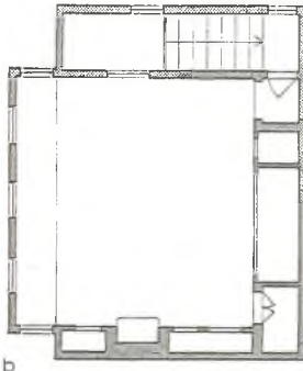
66 Gebze - Tek Odalı ev - 19. Yüzyıl - (Arseven'den)
