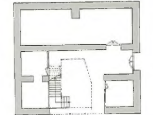
49 Safranbolu - Saraçlar Evi - 20. Yüzyıl başı - Planlar (Günay'dan)
