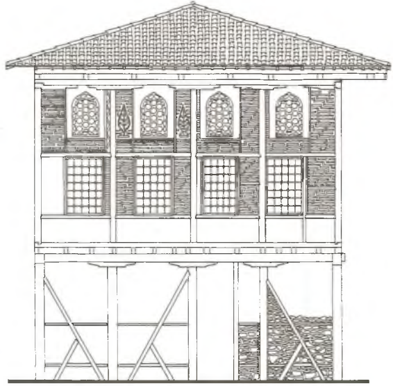
106 Mudanya - Hasan Ağa Evi - Ahşap strüktür
