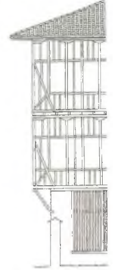
109 Safranbolu - ahşap çatlı
