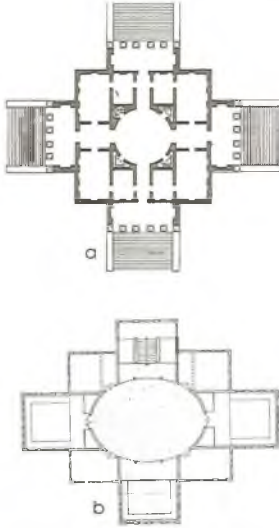
62 İtalya'da ve Türkiye'de merkezi planlı Köşk yorumu
