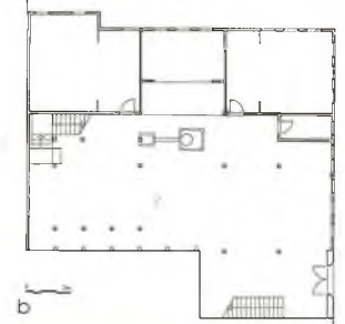
44 İstanbul Bebek - Kavarıyan Evi - 18. Yüzyıl - Planlar
