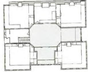
48 Ankara - Değirmenci Ahmet Ağa Evi - 19. Yüzyıl - kat planı, hamamla birlikte (Eldem'den)
