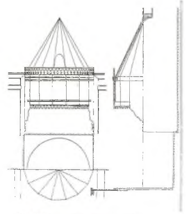
80 Yaygın ocak tipi - plan - kesit ve görünüşü - (Eser'den)
