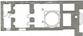
94 İstanbul - Zarif Mustafa Paşa Yalısı - Hamam
