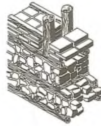
3 Beycesultan -Yapı tekniği- M.Ö. 4. Bin (Naumann'dan)
