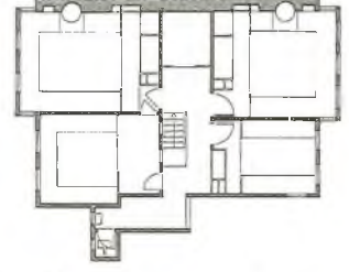
43 Gebze - Kadri Usta Evi - 19. Yüzyıl - Birinci kat planı (Eldem'den)
