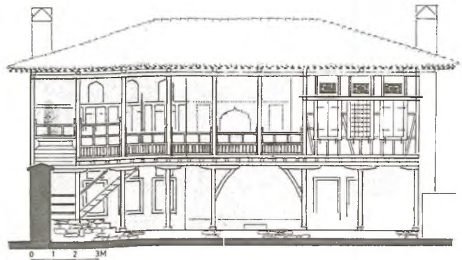
97 Cephe de ahşap strüktür (Eldem'den)
