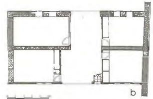
31 Yenişehir - Şemaki Evi a- Birinci kat b- Zemin kat
