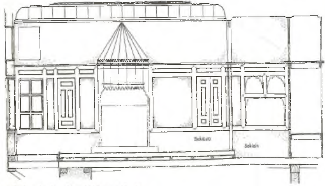
68 Safranbolu - Ocaklı ev - Kesit
