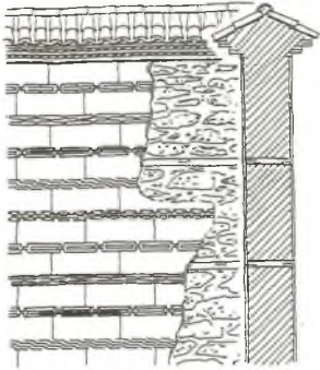
Bahçe duvarı (Eldem'den)
