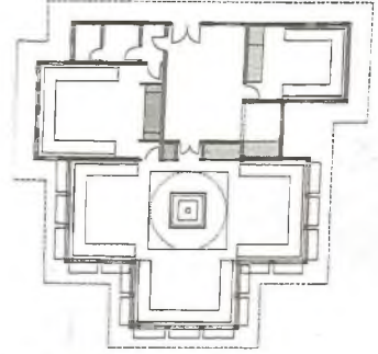
58 İstanbul - Anadoluhisarı - Amcazade Hüseyin Paşa Yalısı, Divanhane - 1700 civarı - plan
