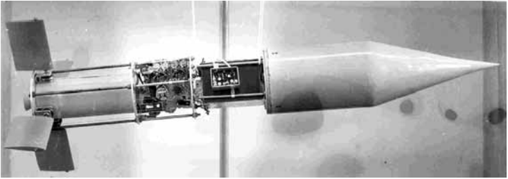
Elektronik Güzüm Sistemi (Roket sadece gösteri içindir, gerçek değildir, ancak arkasındaki dört kumanda kanatçığı, gerçek ORDOT'un önündeki kanatçıklardır)
