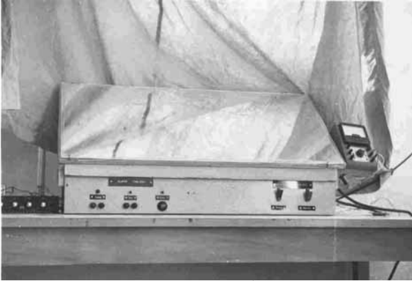
Roket Motoru Deneme Odası (Duvarın arkasında itki ölçüm gerecine bağlı olan roket aynalar aracılığıyla görülmekte)
