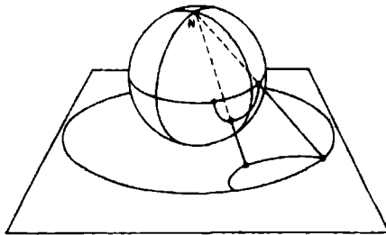
Şekil 6: Poincaré'nin disk modeli 5
