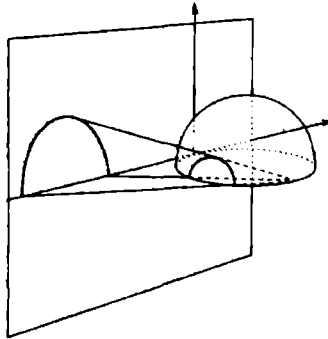
Şekil 7: Poincaré yarım-düzlem modeli 6
