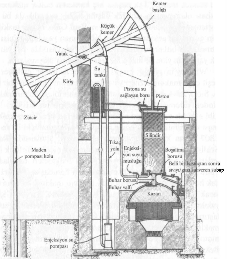
Şekil II.4. Tipik bir Newcomen buhar makinesinin 1715 yılına ait çizimi, içi buhar dolu silindir, su püskürtülerek soğutuluyor. Bu işlemin sonucu olarak silindirin içindeki buhar yoğunlaşarak kısmî bir vakum yaratır. Böylece pistonun dış yüzeyini sıkıştıran hava basıncı pistonun ilk konumuna dönmelerini ve gel-git hareketini tamamlamasını sağlar. Piston, hareket yönündeki en alt noktaya ulaştığında silindirin içine buhar aktarılır ve böylece pistonun iki ucundaki basınç dengelenir. Daha sonra maden pompası mekanizmasının ağırlığı, pistonu silindirin en üst noktasına yükselterek kirişin dönmesini sağlar. Dikkat ederseniz bu makinede buharın ve soğuk suyun silindire girişini ve atık suyun bir pompa aracılığıyla dışarı atılışını kontrol eden subaplar ve musluklar elle çalıştırılacak biçimde tasarlanmıştır. Kaynak: O. B. Barton, The Cornish beam engine (Bath, 1969), s. 17.
