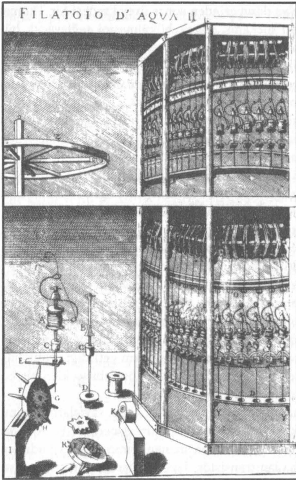
Şekil III.6. Vittorio Zonca'nın suyla çalıştırılan İtalyan ipek ibrişim bükme makinesini gösteren oyma resmi. Resmin yer aldığı bölümün başlığı, makinenin işleyiş biçimlerinden bazılarının daha açık şekilde gösterileceğini imâ ediyordu, ama mekanizmanın iç işleyişine ilişkin bir şey belirtmiyordu. Bu oymanın yayımlanmasından sonra bile İtalyanlar, yüzyıldan daha uzun bir süre boyunca ipek ibrişim endüstrisini tekellerinde bulundurmaya başarmışlardır. Kaynak: Macmillan Yayınevi'nin izniyle, Alex G. Keller'in A theatre of Machines (Makineler Tiyatrosu) adlı kitabından alınarak yeniden yayımlanmıştır, s. 38, 1964.
