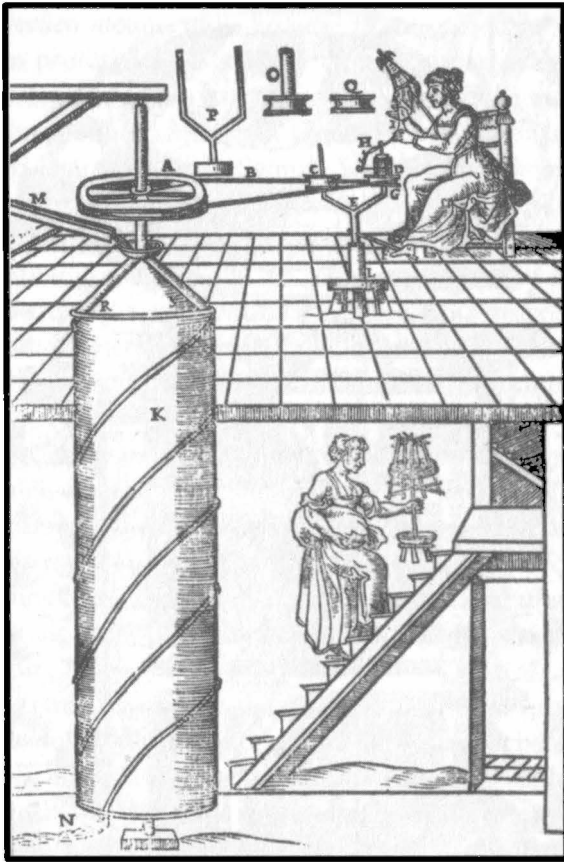
Şekil III.1. Hidrolik Çıkırık. Çıkırık, suyun M kanalından, K silindirin etrafında sarılı bulunan boruya aktarılarak bu boru aracılığıyla akıtılması ile çalıştırılıyor. Bu makinenin resmi Giovanni Branca'nın 1629 yılında yazdığı bir kitapta yer almaktadır. Branca, bu makinenin ipliği eğirmek, sarmak veya dolamak amacıyla kullanılabileceği konusunda bizi temin etmektedir. Ama normalde tek bir ayak pedalı ile çalıştırılan bir çıkırığı döndürebilmek için neden bu kadar fazla enerjiye ve böylesine karmaşık bir mekanizmaya gerek duyulduğu konusunda hiçbir açıklama yapmaz. Kaynak: MacMillan Publishing Company'nin izniyle Alex G. Keller'in A Theatre of Machines (Makineler Tiyatrosu; 1964) adlı kitabından alınmıştır, s.32.
