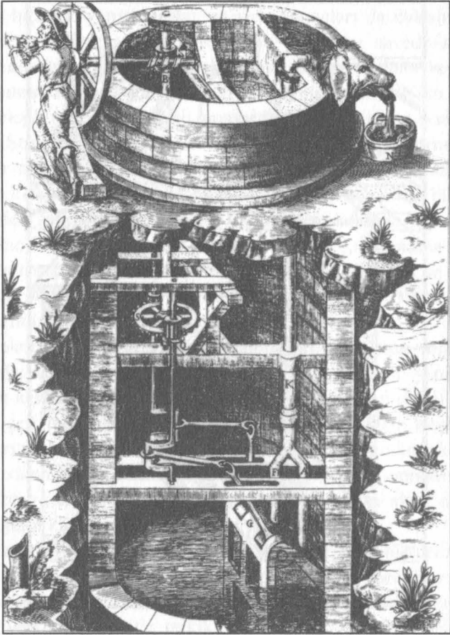
Şekil III.2. Ramelli'nin kitabında yer alan bir su pompasının resmi. Ana pompalama mekanizması, kuyunun sağ alt tarafında bulunan iki büyük kepçeden oluşuyor. Krankın çevrilmesiyle birlikte G odasındaki kepçeler suyu F ve A borularına akmaya ve K borusundaki bir valfın içinden geçmeye zorluyorlar. K borusundaki valf, suyun kuyuya geri akmasını önüyor. Sonuçta su, kuyunun sağ üst köşesinde görülen köpeğin ağzından yerde duran N leğenine akana değin K borusu boyunca yükseliyor. Kaynak: Agostino Ramelli, The various and ingenious machines of Agostino Ramelli (Agostino Ramelli'nin Farklı ve Marifetli Makineleri; Baltimore, 1976), s. 68.
