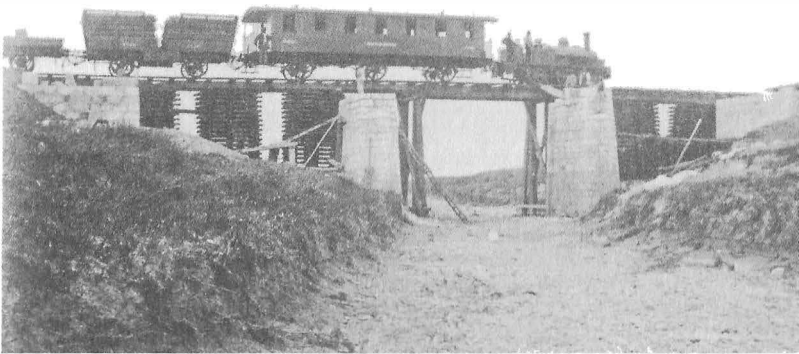
Tarsus yakınlarında (Cydnos) Berdan çayı üzerine inşa edilen demiryolu köprüsü
