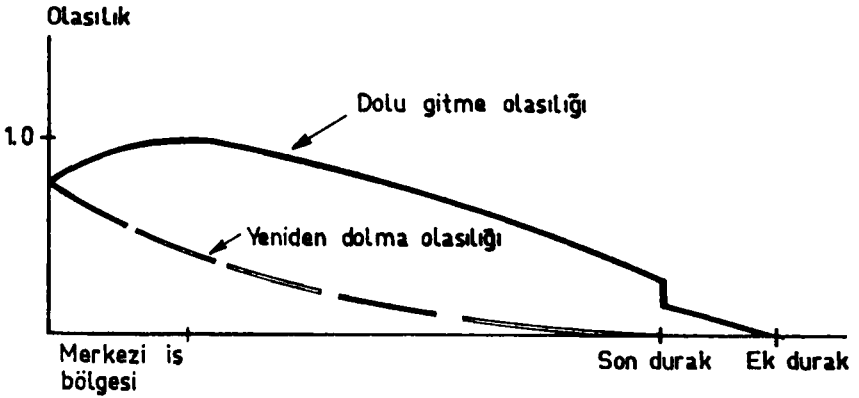
Çizim: 6.7 Bir minibüs dolmuşun dolu gitme ve yeniden dolma olasılıkları
