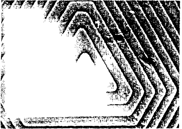
Plaka 2- Silikon karbid kristallerinin oluşumu (400 kez büyütülmüş)
