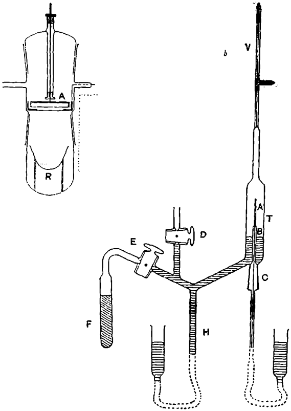
Resim 15 : Rutherford'un radyoaktivite üzerine olan ve kullanılan aletlerin olağanüstü basitliğini gösteren iki esas deneyi
