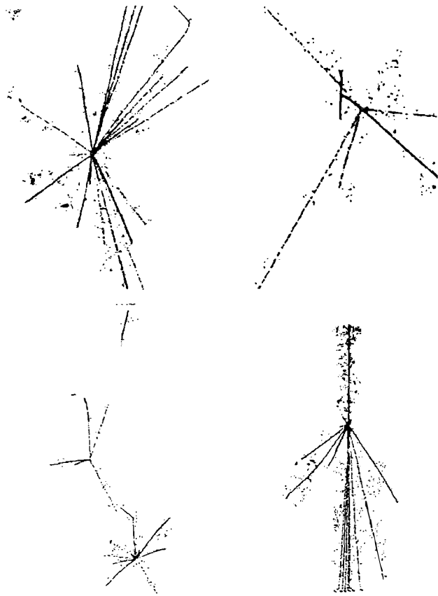
Plaka 1- Kozmik ışınların ürettiği ve fotoğraflık emülsiyonlar üzerine kaydedilen çekirdek parçalanmaları
