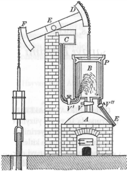
Resim 9: Thomas Newcomen'in buhar makinesi çizimi.
