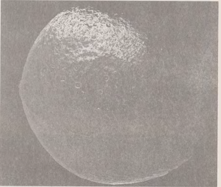
Görsel 25: Iapetus
