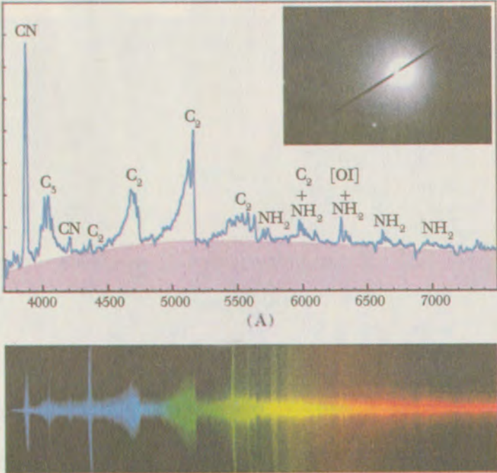
Görsel 23: Neat Kuyruklu yıldız Tayfı
