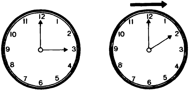
Şekil-19: Artık fizikçiler için rutin bir deneyim olan zaman genişlemesi etkisi, hızlı hareket eden hassas atomik saatler veya bozunum oranları bilinen atomaltı parçacıklar kullanılarak gösterilebilir. Hareket eden saat diğer saate göre daha yavaş işler. Bir astronotun yüksek hızlı bir uzay yolculuğundan dünyadaki kardeşinden birkaç yıl daha genç bir halde döndüğü ünlü "ikizler etkisi" buradan doğmaktadır.
