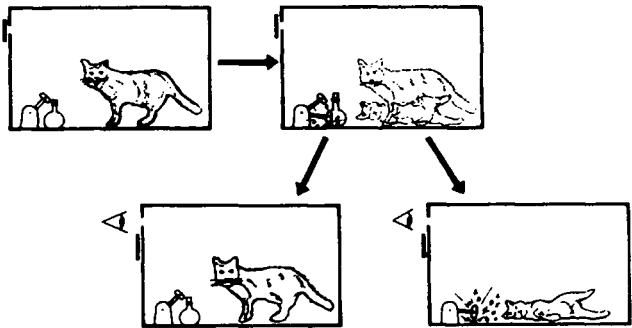
Şekil-17: Schrödinger'in kedisinin acıklı hikâyesi. Bir kuantum süreci siyanürün bırakılmasını yüzde 50'ye 50'lik bir olasılıkla tetikleyebilir. Kuantum kuramı gereğince sistem, bir gözlem yapıp ya bir canlı kedi ya da bir ölü kedi elde edilinceye dek hayalet benzer karma bir canlı-ölü kedi durumundadır. Bu düşünce deneyi kuantum kuramında gözlem faaliyetinde saklı olan acayip anlamı açığa çıkartmaktadır.
