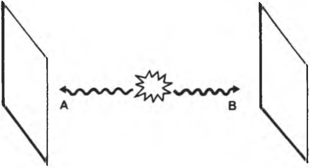
Şekil-12: Bağlantılı spin ve kutuplara sahip iki foton paralel iki kutuplaştıran malzemeye karşılaştıklarında yüzde yüz işbirliği gösterirler: Foton A engellendiğinde B de engellenir. Bu işbirliği, (i) foton ile kutuplaştırmacı arasındaki karşılaşmanın gerçek ürünü tamamen öngörülemez olduğunda bile ve (ii) fotonlar birbirlerinden çok uzakta olsalar bile gerçekleşir.
