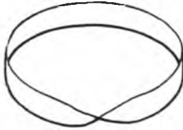
Şekil-10: Ünlü Möbius şeridi bir şeridin ters bükülerek iki ucunun bir halka oluşturacak şekilde birleştirilmesiyle yapılır. Yapılan dikkatli bir inceleme şeridin artık sadece tek bir taraf ve yüze sahip olduğunu gösterecektir.
