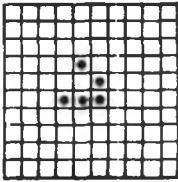
Şekil-26: "Planör" adı verilen beş taşlık düzenleme, pano boyunca çaprazlama hareket ederken bütünlüğünü aynen koruyabilme gibi ilginç bir özelliğe sahiptir. Sekiz taştan oluşan daha büyüğüne "uzay gemisi" denir ve o da bütünlüğünü korur, ancak ilerlerken "kıvılcımlar" salar.
