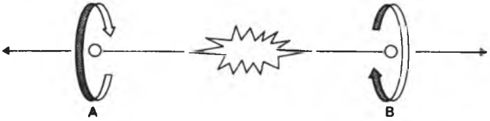
Şekil-11: Bir atomun veya çekirdek altı parçacığın bozunumu, zıt yönlerde muhtemelen büyük bir uzaklığa dek ilerleyen, birbirlerine zıt spinli iki parçacık üretebilir.
