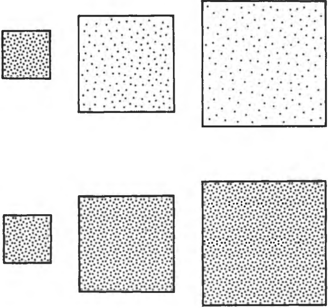
Şekil-3: Çizim genişleyen uzayın bir bölgesinin Büyük Patlama ve durağan evren modellerinde birbiri ardına üç "fotoğrafını" karşılaştırmaktadır. Büyük Patlamada (üstteki) verili bir uzay hacmindeki galaksilerin sayısı (noktalar) değişmeden kalır. Bu yüzden genişleme devam ettikçe noktaların yoğunluğu azalır. Durağan evren modelinde (alttaki) galaksilerin yoğunluğu tüm çağlar boyunca değişmeden kalır ancak genişleyen uzayın doğurduğu boşlukları doldurmak için sürekli yeni galaksilerin yaratılması şarttır.
