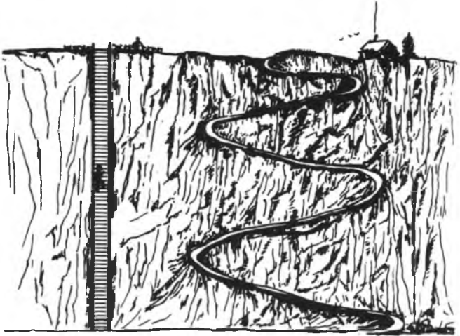
Şekil-24: Bayır yürüyüşü örneği soyut "ayar simetrisi" kavramını açıklayıcıdır. Bayırın tepesine ulaşırken harcanan toplam enerji, ister kısa zorlu dik rota ister uzun kolay zikzaklı rota seçilsin aynıdır. Bu kütleçekim alanının derin ve tesirli simetrisini yansıtır. Birleşik alan kuramlarının son dönemdeki matematik formülasyonları sayesinde doğanın diğer kuvvet alanlarında da benzer ama daha karmaşık simetrilere ulaşılmıştır.
