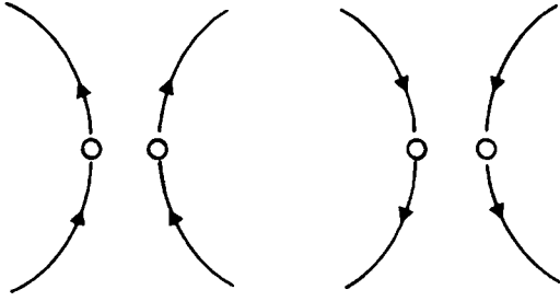
Şekil-22: Maddeyi atomik düzeyde incelediğimizde dünyadaki zaman asimetrisinin kökeni bir muammadır. Herhangi iki molekül arasındaki çarpışma tamamıyla geri döndürülebilir niteliktedir ve ayrıcalıklı bir geçmiş-gelecek uyumlanması sergilemez.
