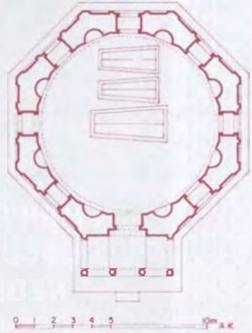
Hürrem Sultan Türbesi'nin planı
