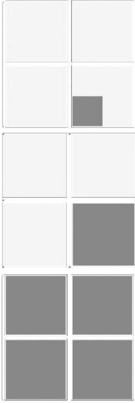
ŞEKİL 2. Yeniden normalleştirme grubu, birden üçe kadar aşamalar (yukarıdan başlayarak): Dört kutu içeren üç kutu, kutulardan biri birinci aşamada koyu renkli, onu azınlık kuralının ardışık uygulamaları takip ediyor.
