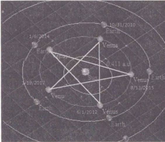
Venüs Döngüsü
