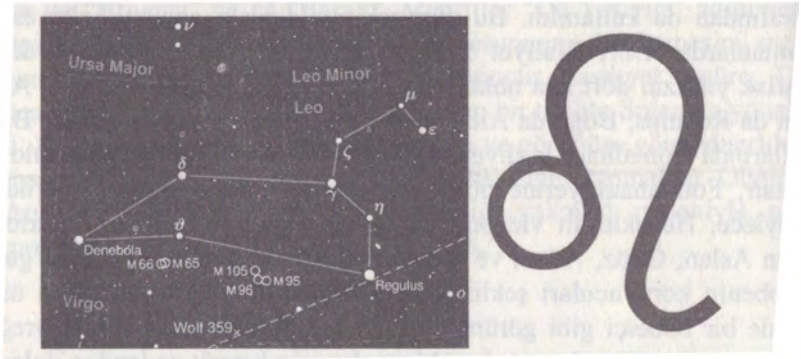
Aslan Takımyıldızı
