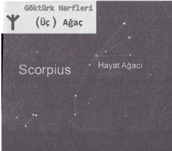
Akrep Takımyıldızı
