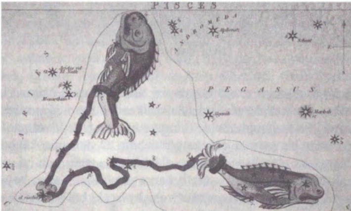
Balık Takımyıldızı
