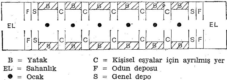
38. Bir Irok uzun evi planı.
