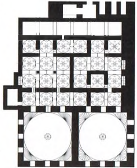
Haseki Sultan Hamamı Kubbe Planı
