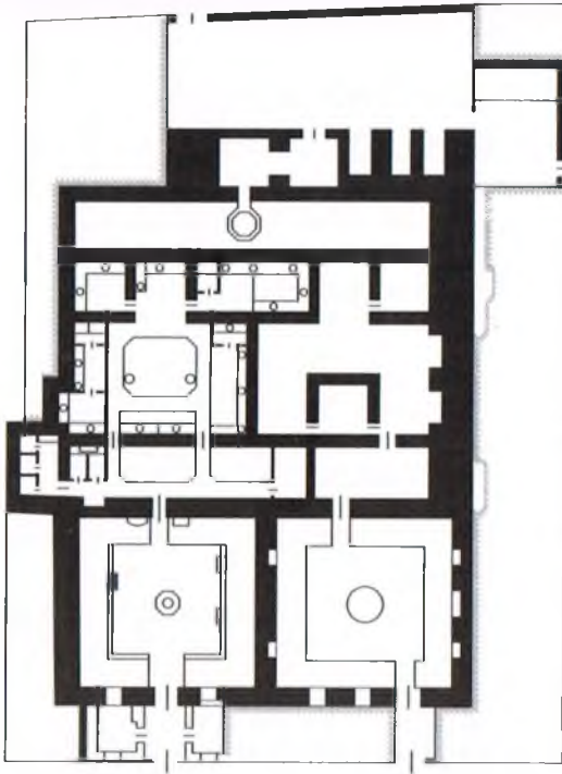
Haseki Sultan Hamamı Döşeme Planı
