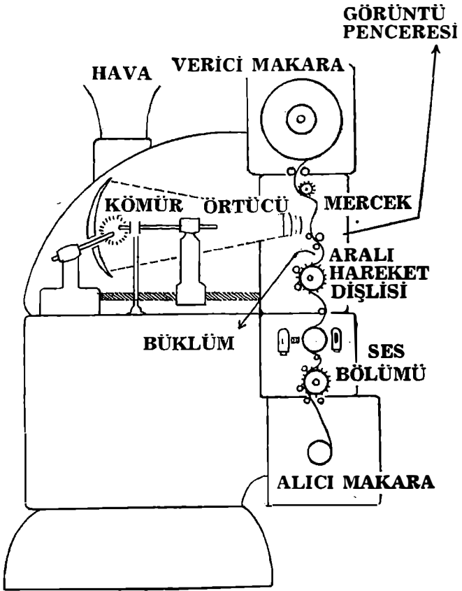
Göstericinin yapısı
