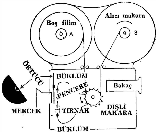
Alicının yapısı
