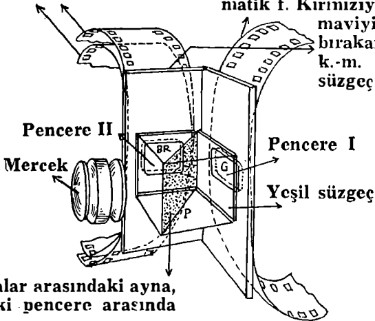
Technicolor alıcısının optik düzeni
