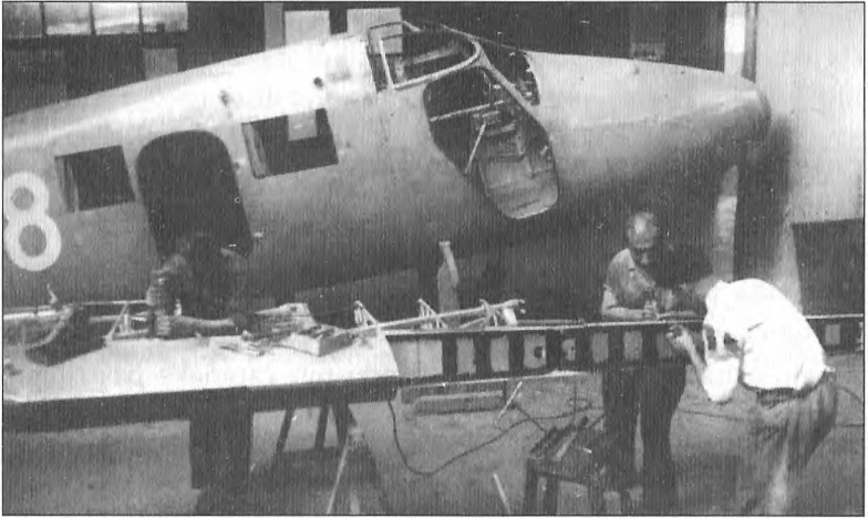
Nu.D-38'in yapım aşamalarından bir görünüş
