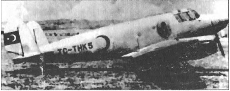
THK Uçak Fabrikası’nda üretilip Danimarka’ya ihraç edilen THK-5 ambulans uçağı
